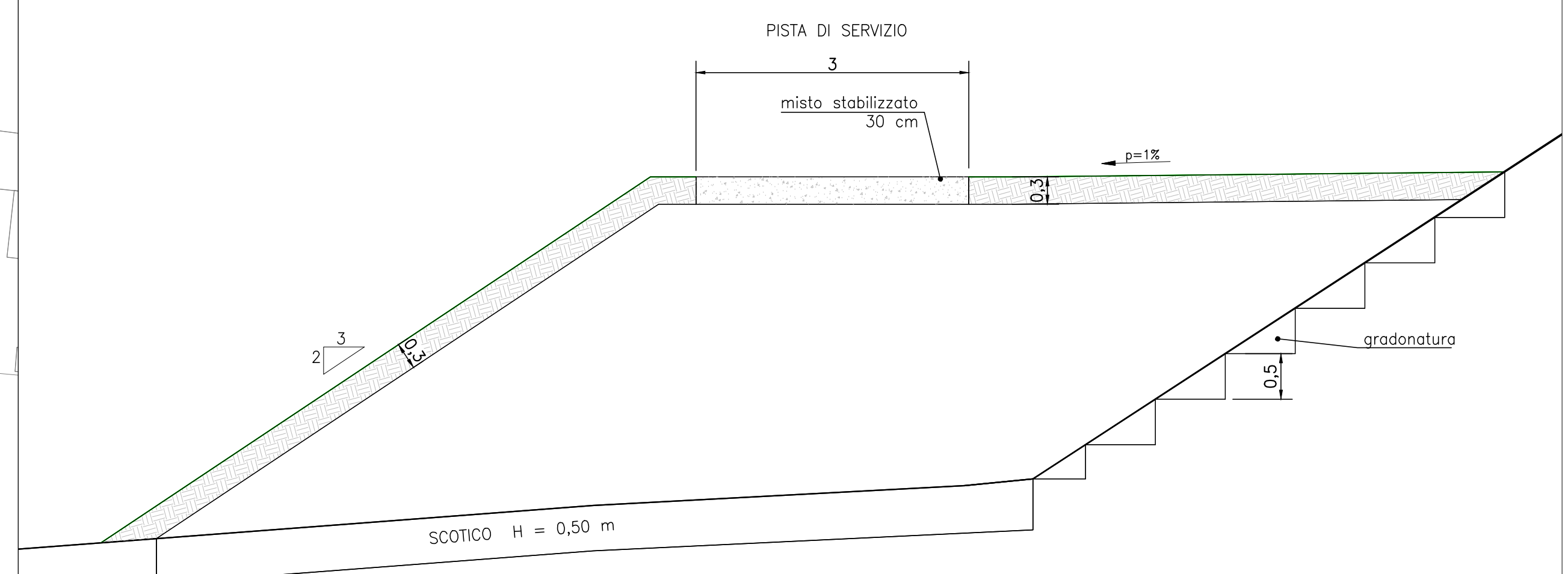
SEZIONE TIPO - PISTA DI SERVIZIO Scala 1:50
