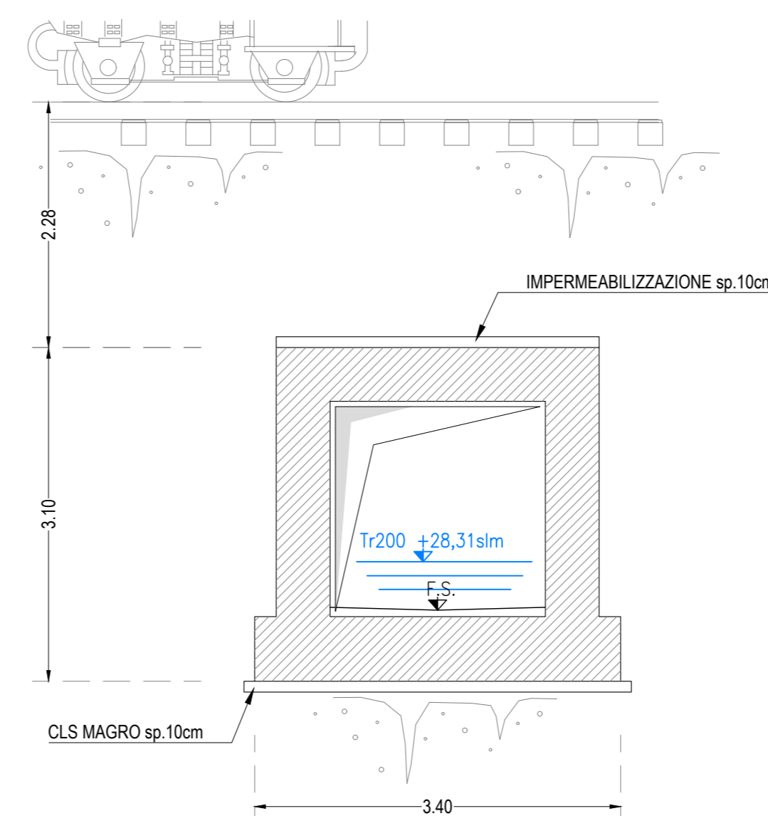
SEZIONE TIPOLOGICA MANUFATTO DI ATTRAVERSAMENTO scala 1:50
