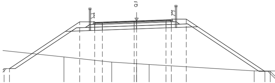
Figura 8.3.2: Sezione A2 del rilevato di approccio alla spalla A, tra pk 0+180 e pk 0+160
