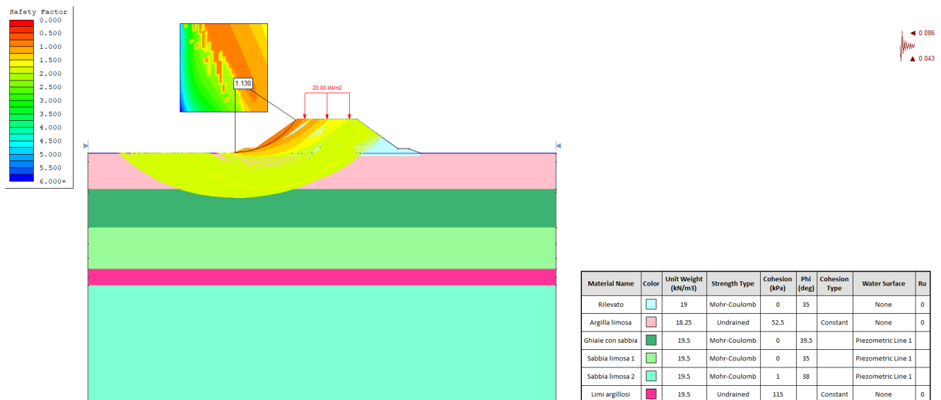
Figura 9.1.3: Spalla A: Rilevato H=6.2 m, - Analisi di stabilità globale in campo sismico
