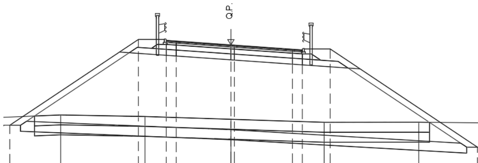
Figura 8.3.4: Sezione B2 del rilevato di approccio alla spalla B, tra pk 0+440 e pk 0+460
