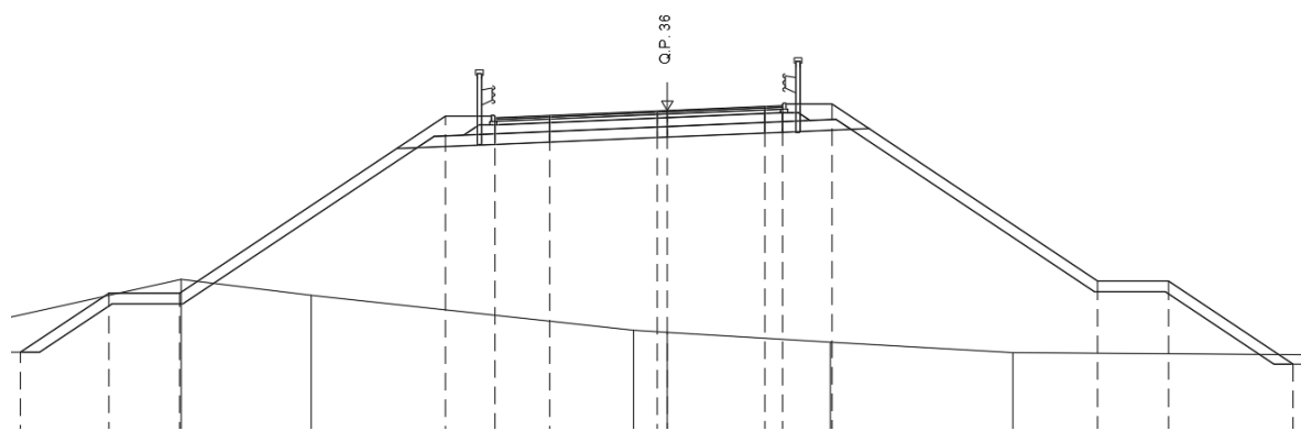
Figura 8.3.1: Sezione A1 del rilevato di approccio alla spalla A, tra pk 0+219 e pk 0+180
