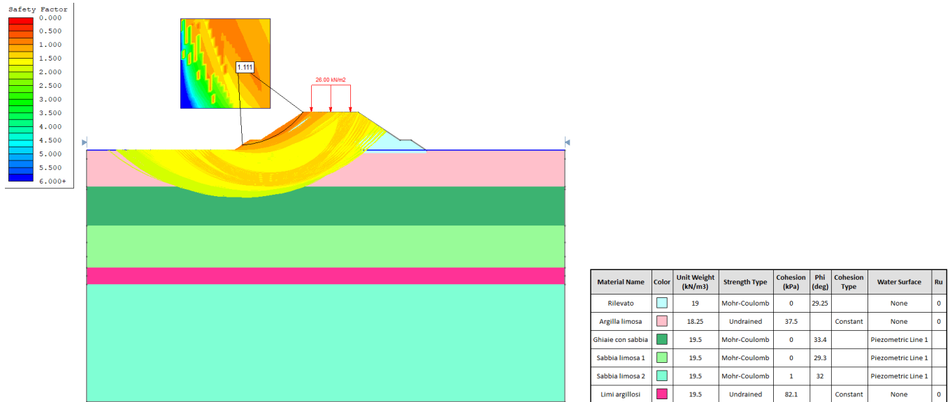
Figura 9.1.4: Spalla B. Rilevato H=6.8 m, - Analisi di stabilità globale in campo statico
