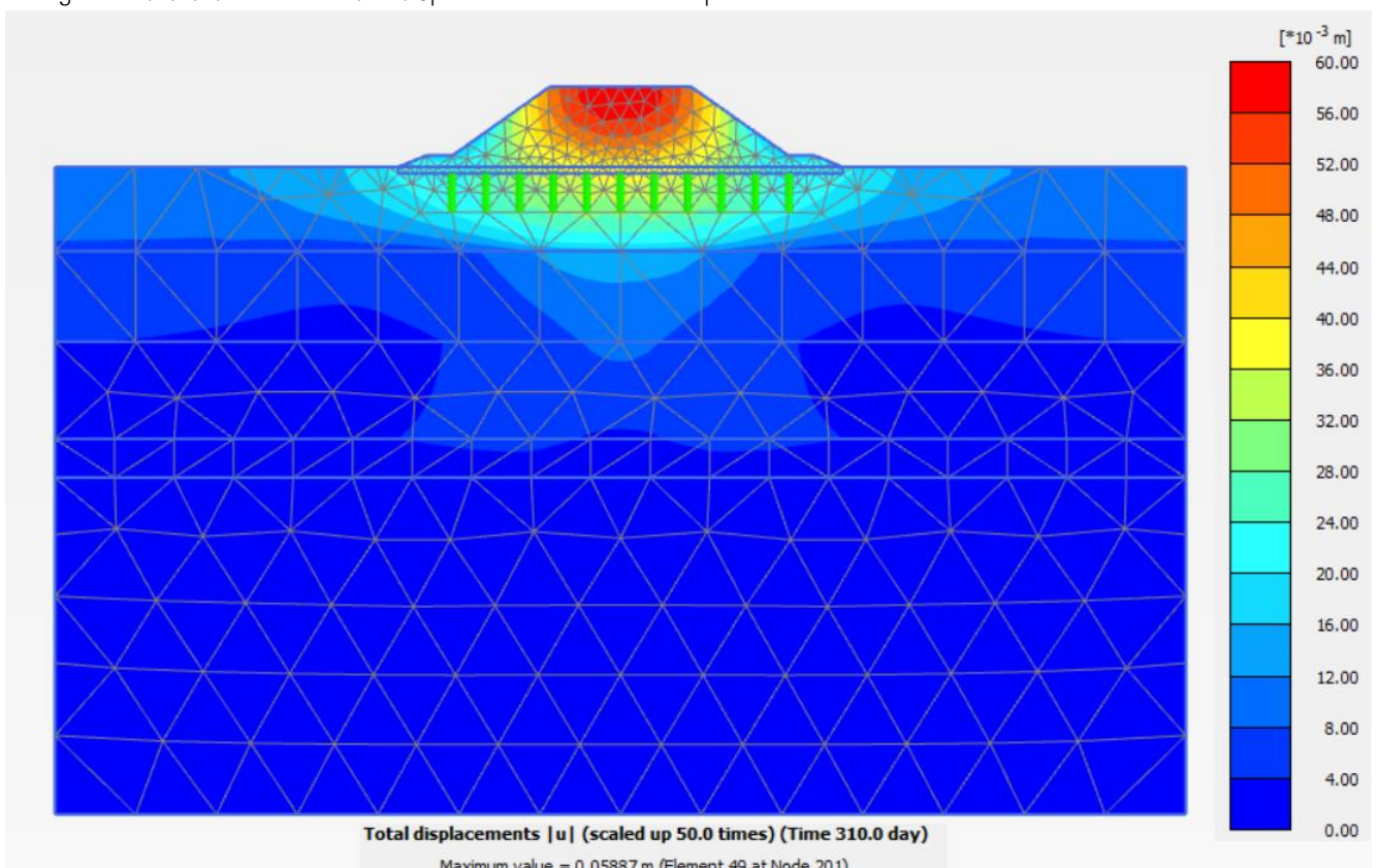
Figura 10.1.1.3: Rilevato sez. A1 - Spostamenti totali termine costruzione
