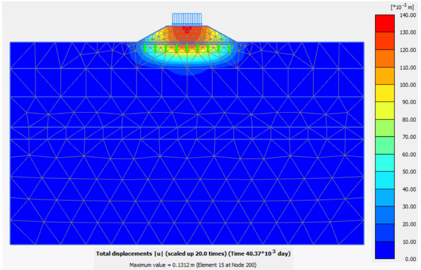
Figura 10.1.2.4: Rilevato sez. A2 – Spostamenti totali lungo termine
