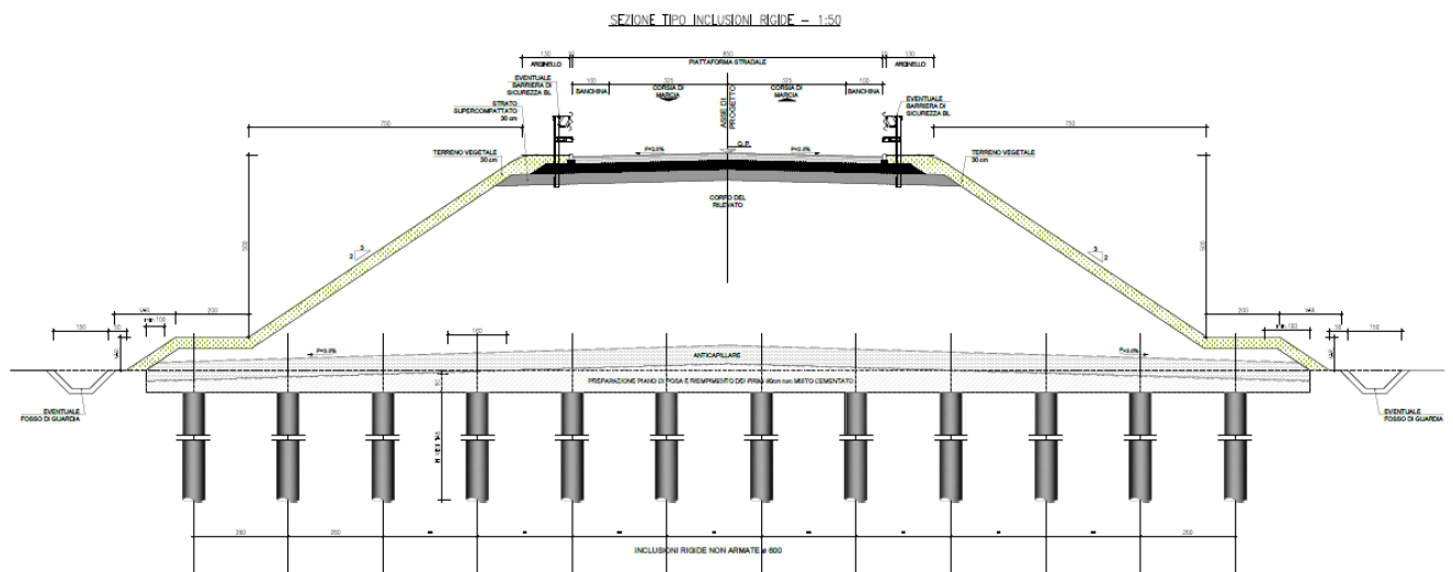
Figura 4.1 – Sezione tipo del rilevato di approccio spalla A-B con inclusioni rigide
