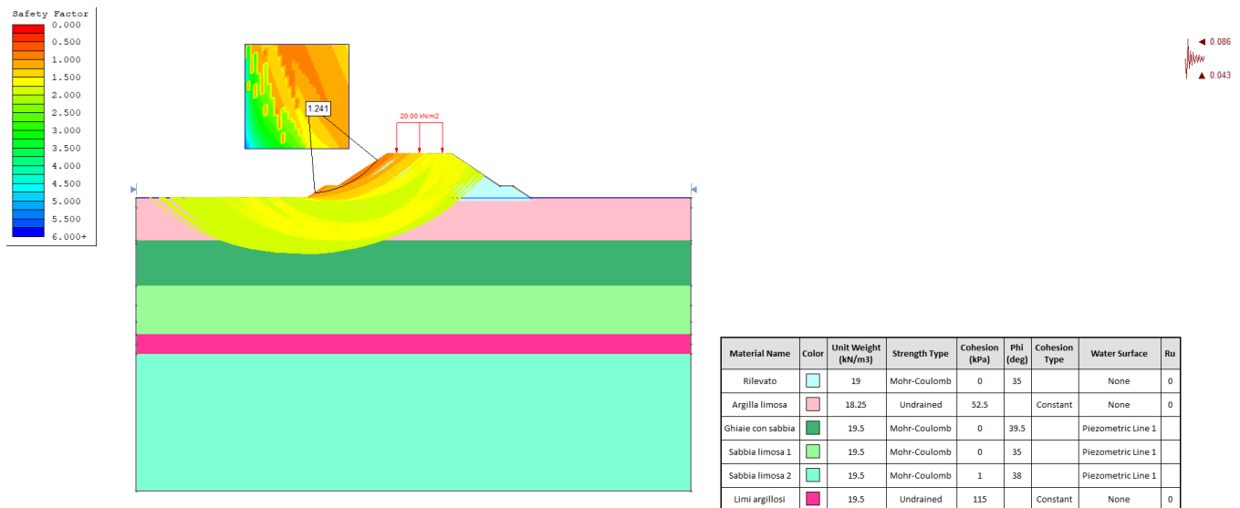
Figura 9.1.5: Spalla B: Rilevato H=6.8 m, - Analisi di stabilità globale in campo sismico
