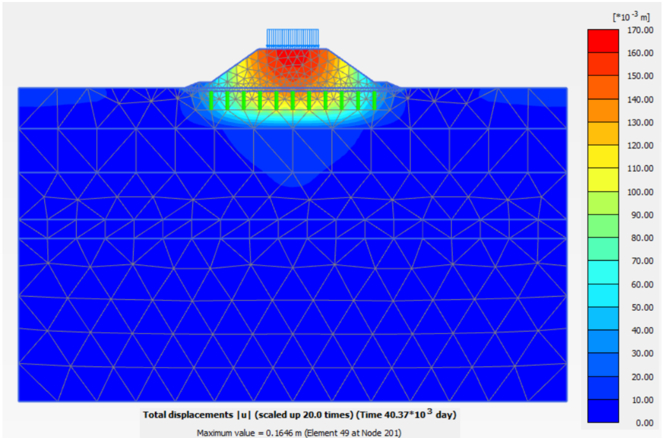
Figura 10.1.1.4: Rilevato sez. A1 - Spostamenti totali lungo termine
