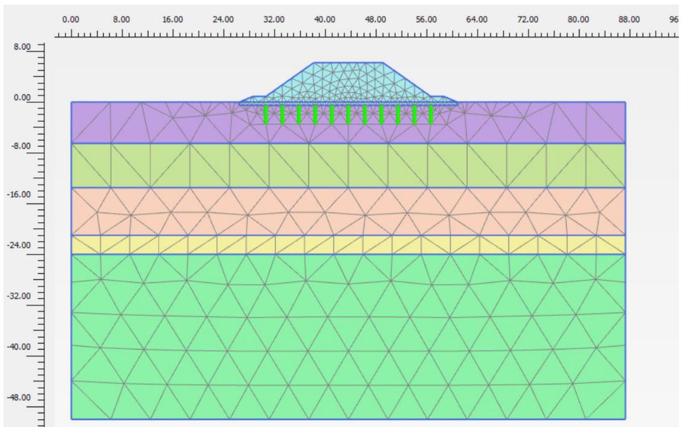
Figura 10.1.1.1: Modello rilevato sezione A1
