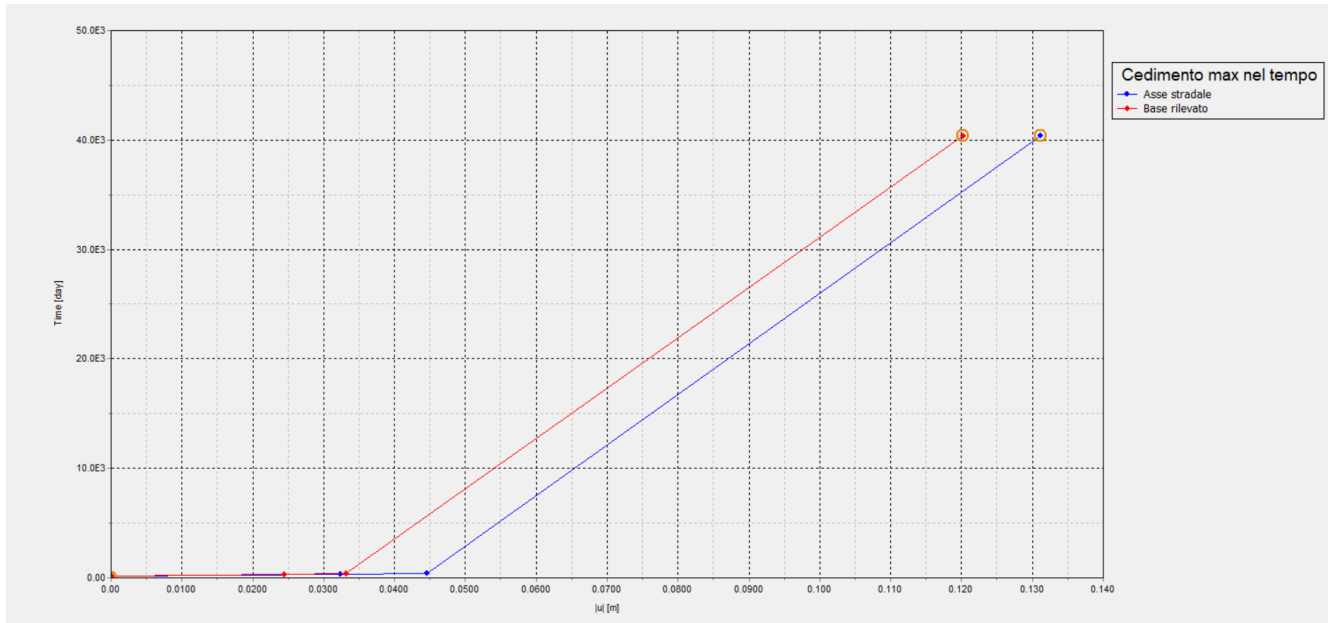
Figura 10.1.2.2: Rilevato sez. A2 – Spostamenti totali in corrispondenza sia dell'asse stradale che della base del rilevato
