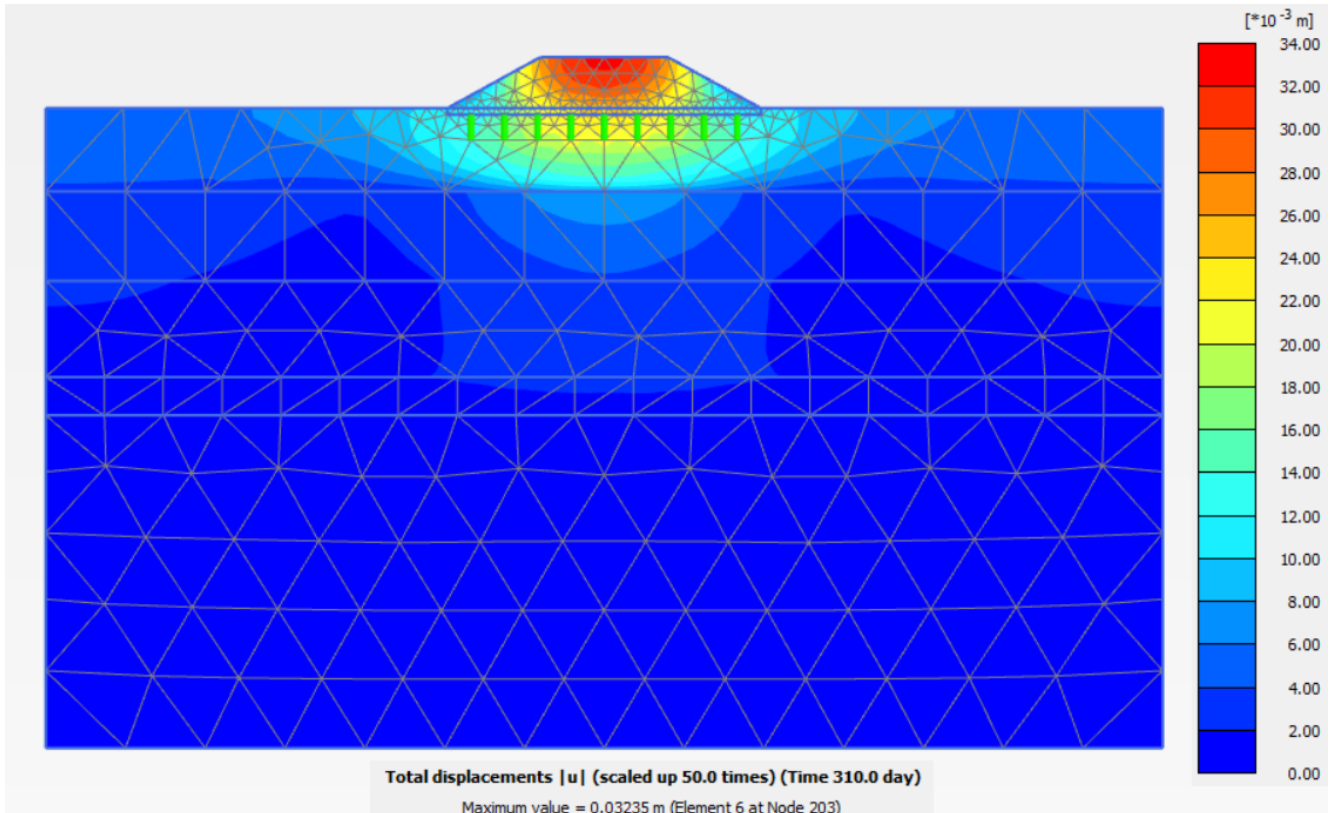
Figura 10.1.2.3: Rilevato sez. A2 – Spostamenti totali termine costruzione
