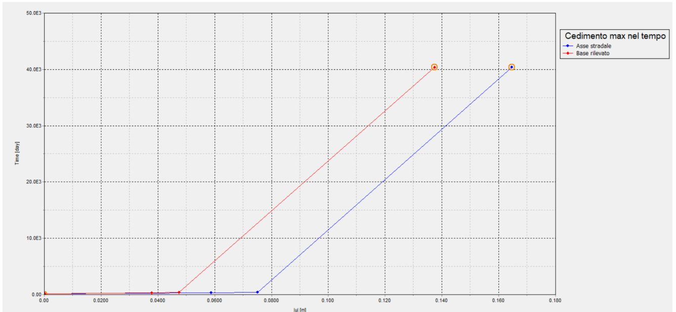
Figura 10.1.1.2: Rilevato sez. A1: Spostamenti totali in corrispondenza sia dell'asse stradale che della base del rilevato
