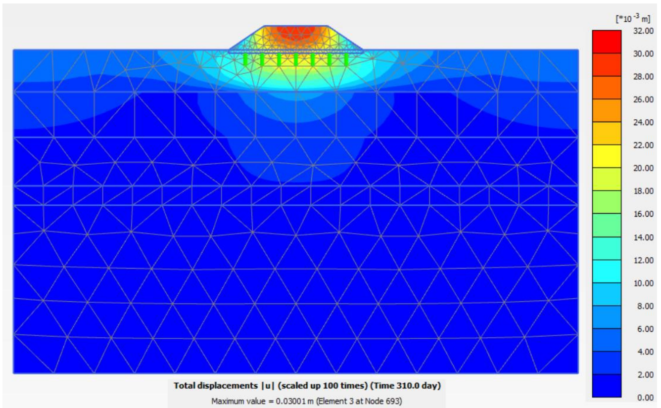
Figura 10.1.4.3: Rilevato sez. B2 – Spostamenti totali termine costruzione
