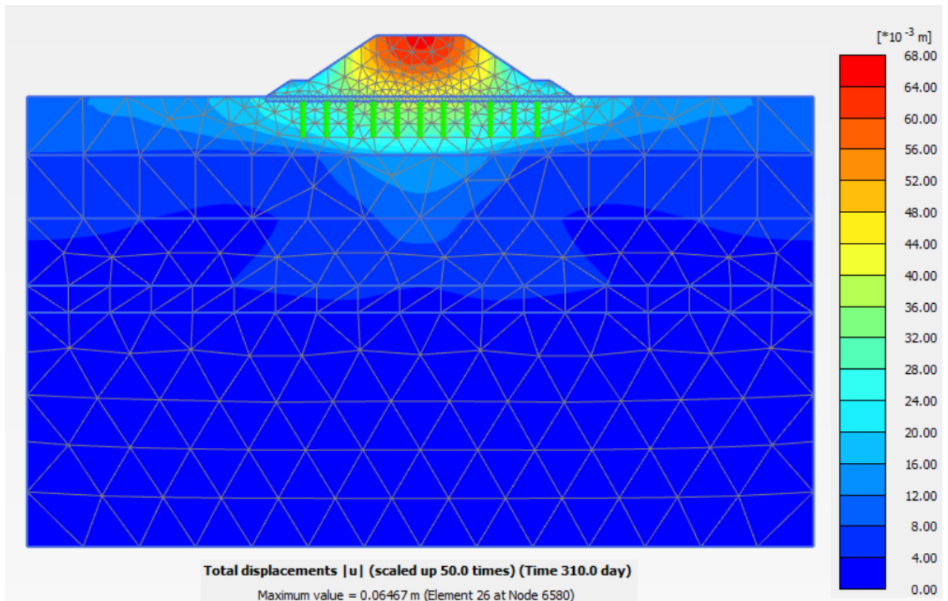
Figura 10.1.3.3: Rilevato sez. B1 – Spostamenti totali termine costruzione
