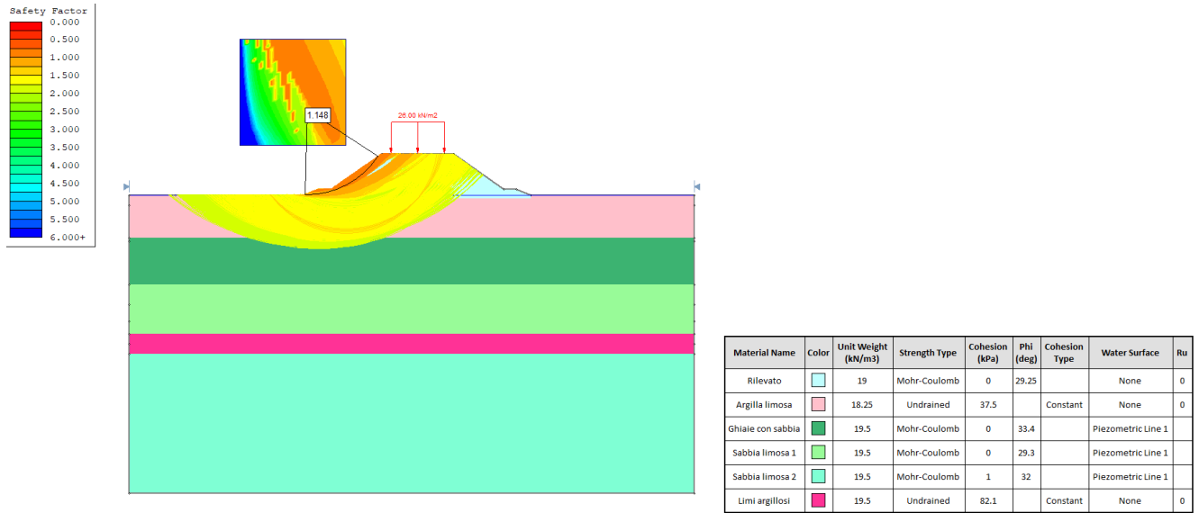
Figura 9.1.2: Spalla A. Rilevato H=6.2 m, - Analisi di stabilità globale in campo statico
