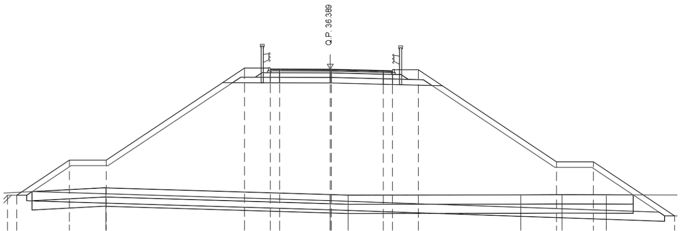
Figura 8.3.3: Sezione B1 del rilevato di approccio alla spalla B, tra pk 0+403 e pk 0+440
