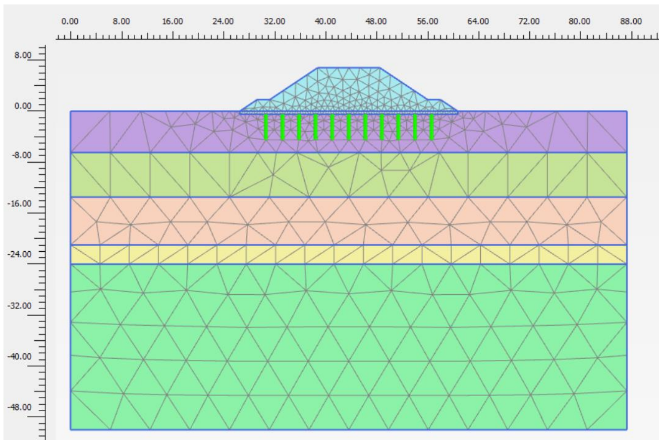
Figura 10.1.3.1: Modello rilevato sezione B1
