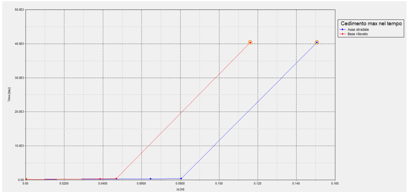
Figura 10.1.3.2: Rilevato sez. B1 – Spostamenti totali in corrispondenza sia dell'asse stradale che della base del rilevato
