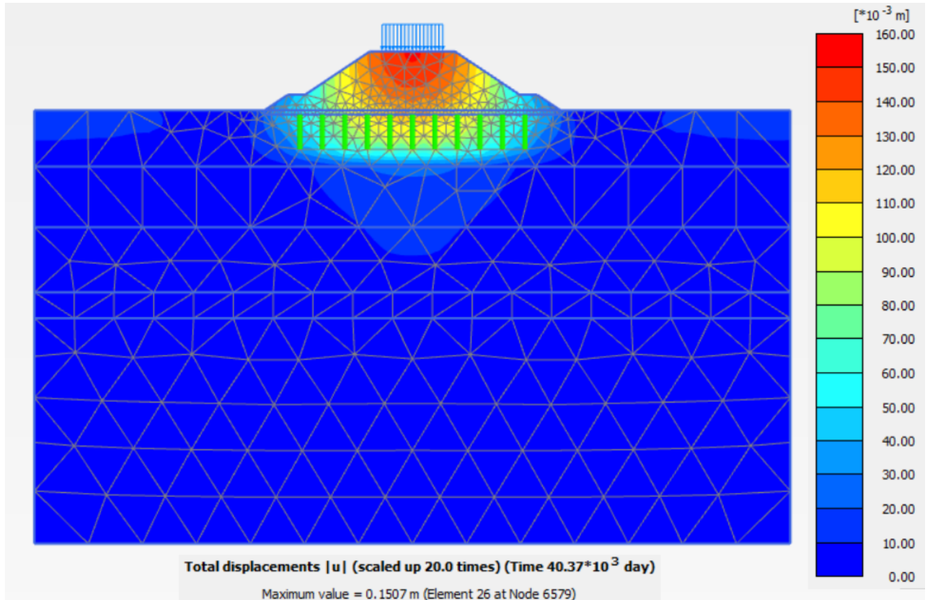
Figura 10.1.3.4: Rilevato sez. B1 – Spostamenti totali lungo termine
