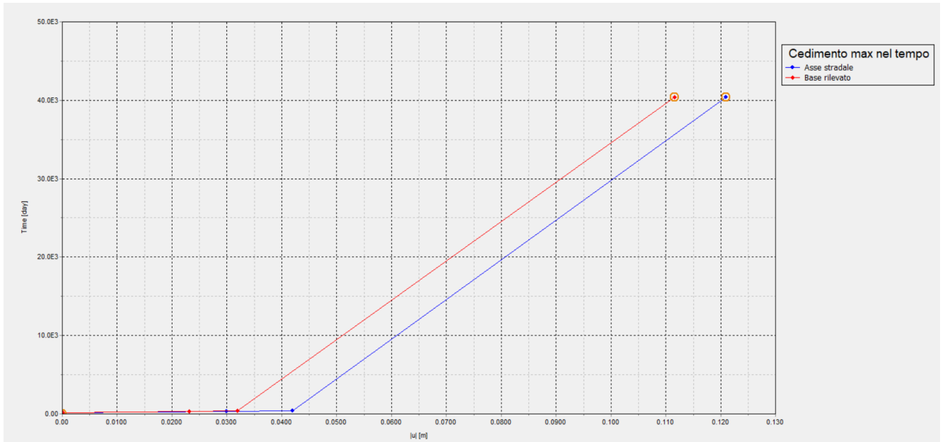
Figura 10.1.4.2: Rilevato sez. B2 – Spostamenti totali in corrispondenza sia dell'asse stradale che della base del rilevato
