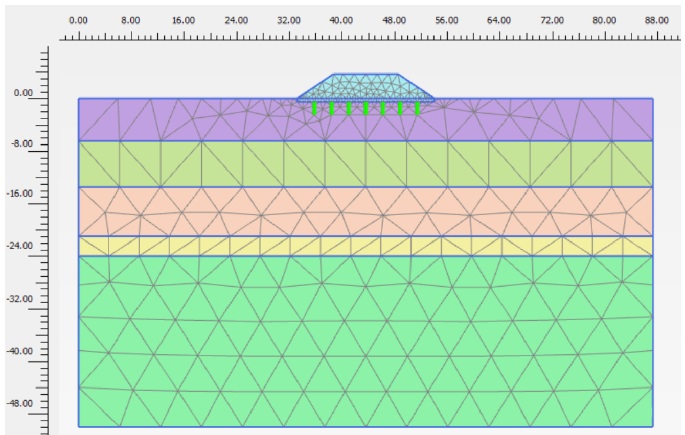
Figura 10.1.4.1: Modello rilevato sezione B2
