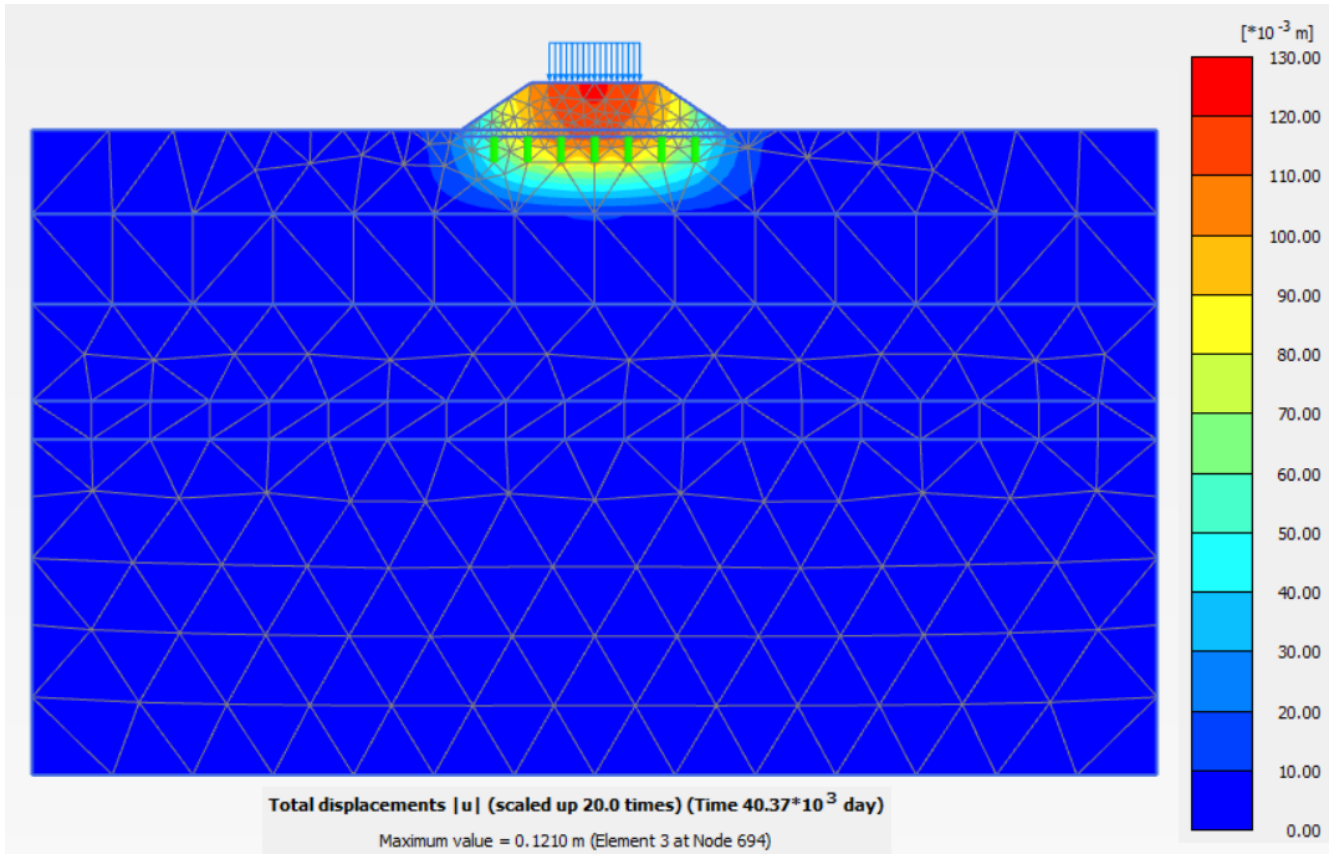
Figura 10.1.4.4: Rilevato sez. B2 – Spostamenti totali lungo termine
