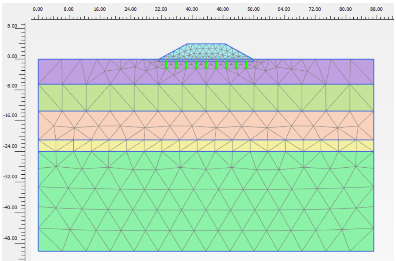
Figura 10.1.2.1: Modello rilevato sezione A2
