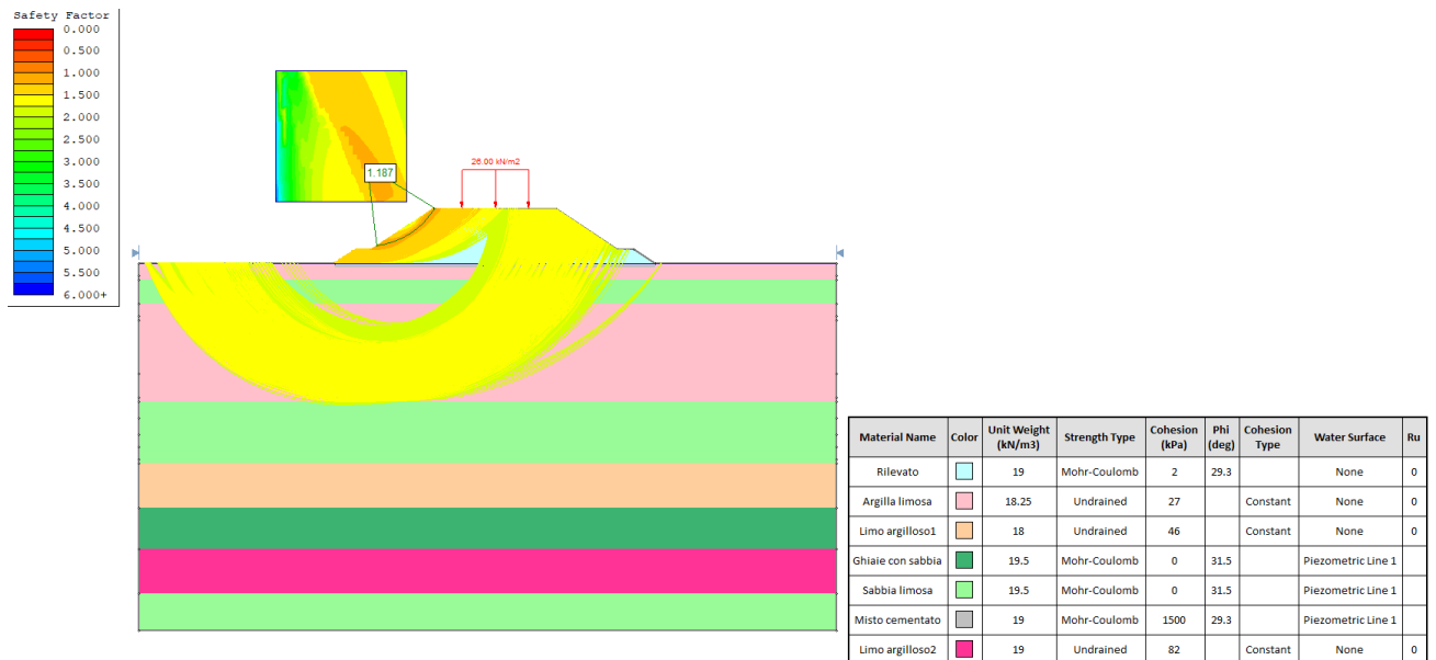
Figura 8.2.3: Spalla B. Rilevato H=7 m, - Analisi di stabilità globale in campo statico
