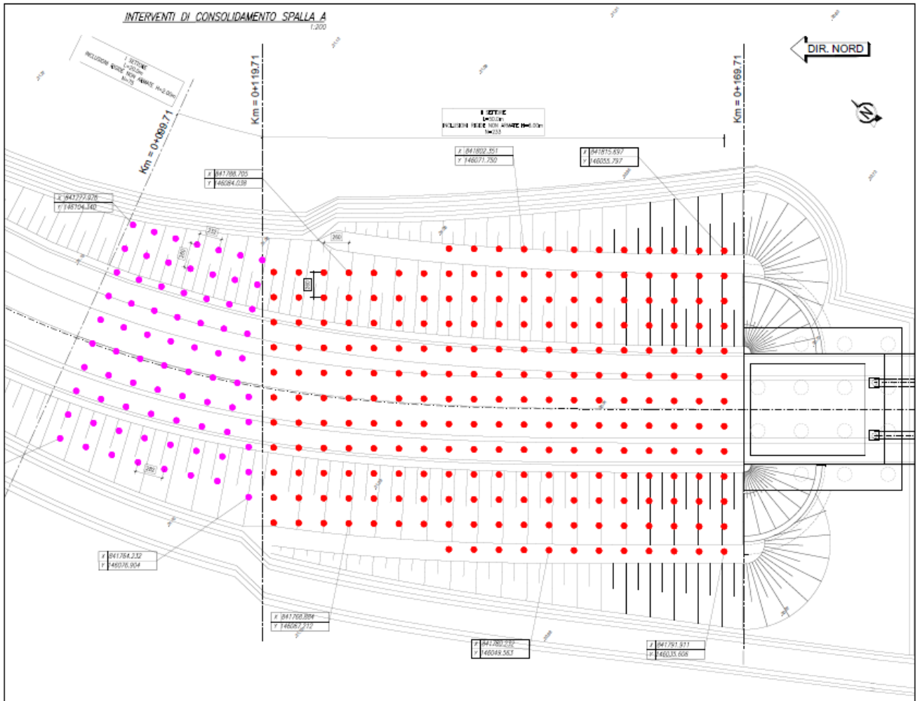
Figura 10.1: Rilevato di appoggio spalla A – Planimetria di progetto delle inclusioni rigide
