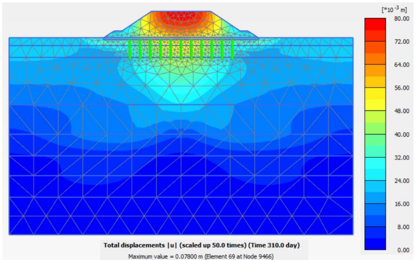
Figura 9.1.3.3: Rilevato sez. B1 – Spostamenti totali termine costruzione
