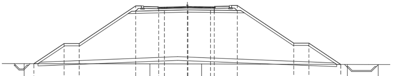
Figura 7.3.1: Sezione A1 del rilevato di approccio alla spalla A, tra pk 0+170 e pk 0+120
