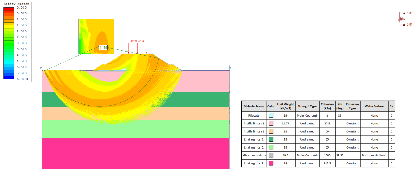
Figura 8.1.2: Spalla A: Rilevato H=7.6 m, - Analisi di stabilità globale in campo sismico
