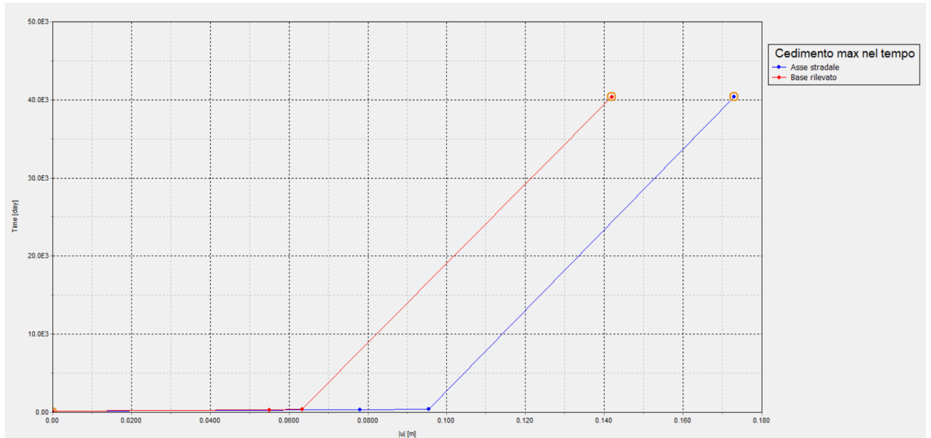
Figura 9.1.3.2: Rilevato sez. B1 – Spostamenti totali in corrispondenza sia dell'asse stradale che della base del rilevato
