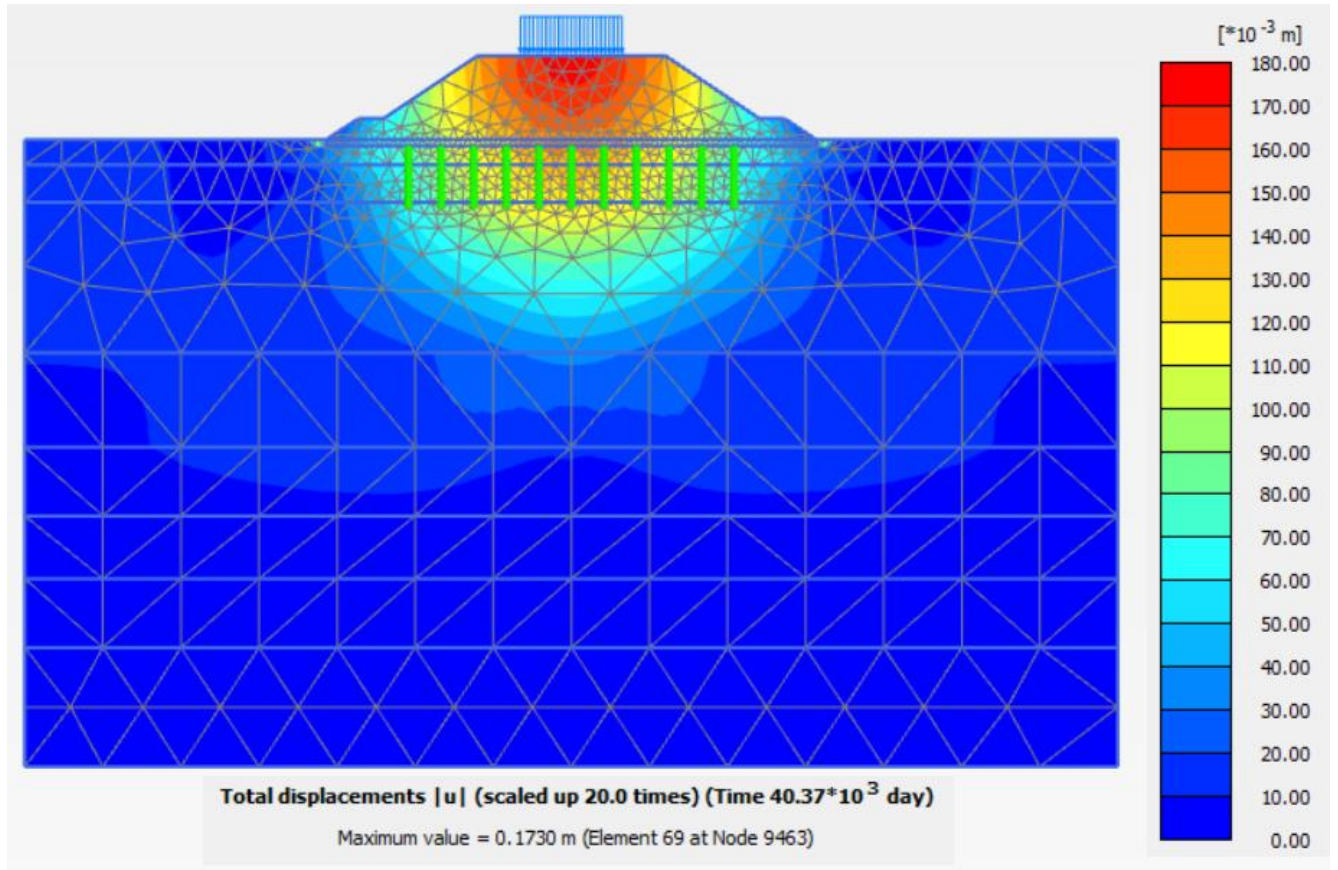
Figura 9.1.3.4: Rilevato sez. B1 – Spostamenti totali lungo termine
