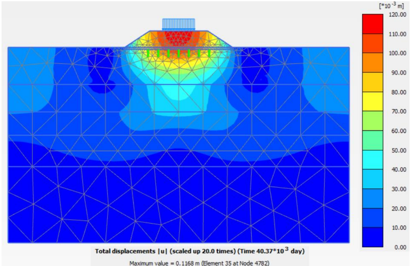
Figura 9.1.2.4: Rilevato sez. A2 – Spostamenti totali lungo termine
