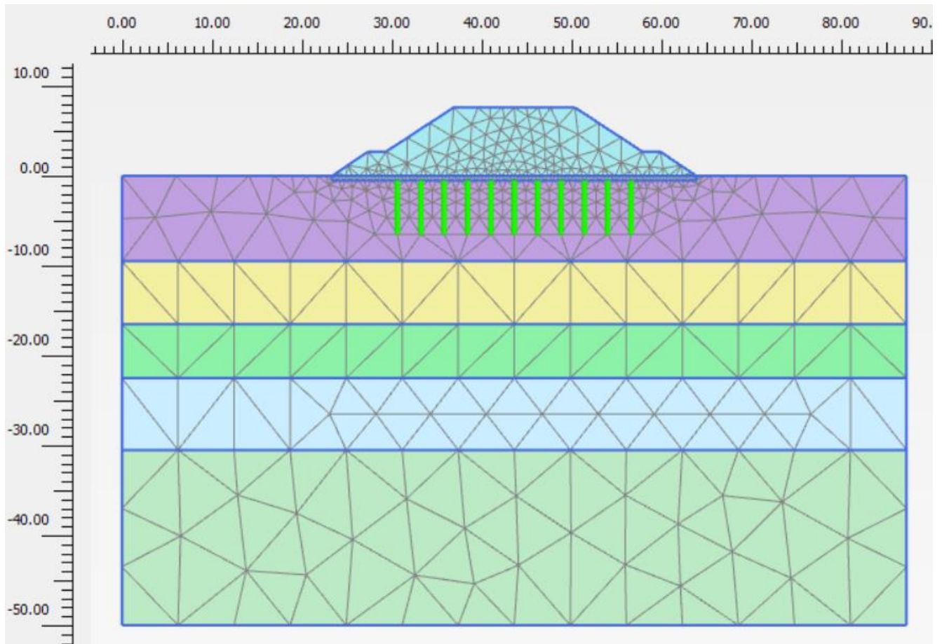
Figura 9.1.1.1: Modello rilevato sezione A1
