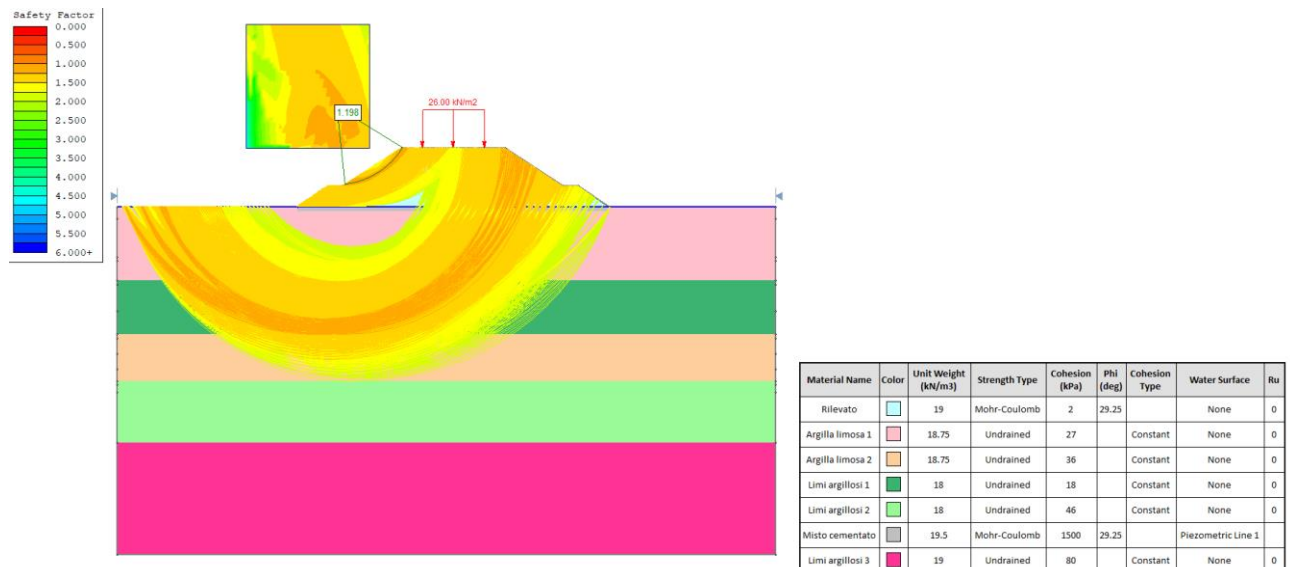
Figura 8.1.1: Spalla A. Rilevato H=7.6 m, - Analisi di stabilità globale in campo statico
