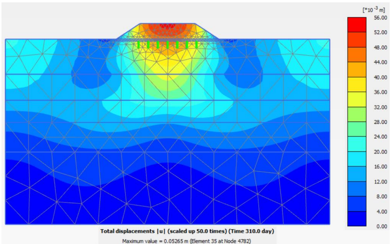
Figura 9.1.2.3: Rilevato sez. A2 – Spostamenti totali termine costruzione
