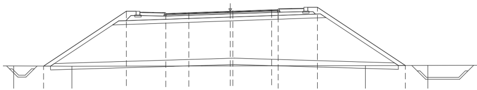
Figura 7.3.2: Sezione A2 del rilevato di approccio alla spalla A, tra pk 0+120 e pk 0+100
