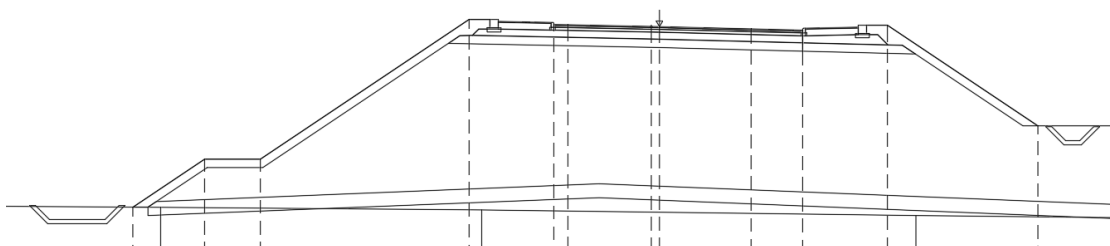
Figura 7.3.3: Sezione B1 del rilevato di approccio alla spalla B, tra pk 0+362 e pk 0+400
