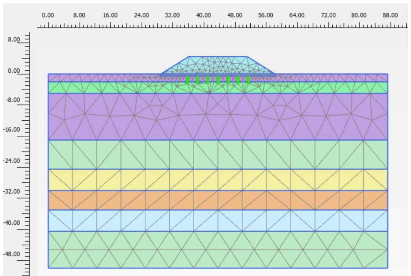
Figura 9.1.4.1: Modello rilevato sezione B2
