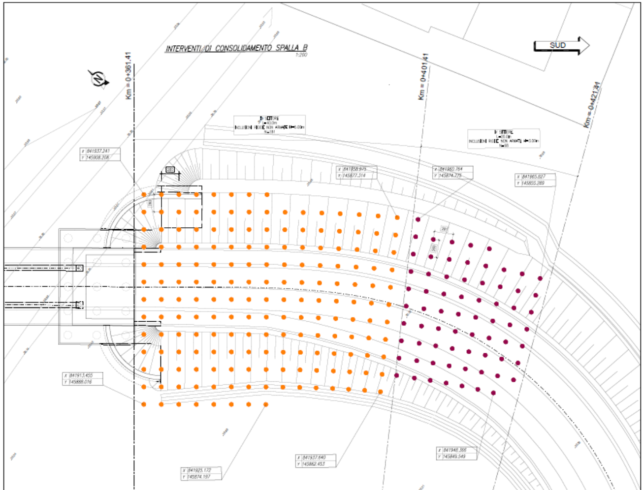
Figura 10.2: Rilevato di approccio spalla B – Planimetria di progetto delle inclusioni rigide
