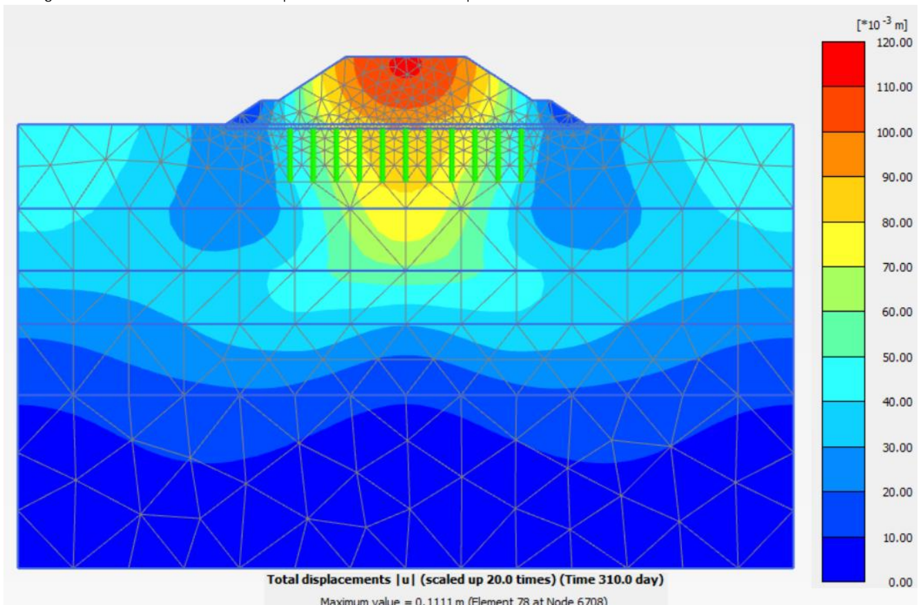
Figura 9.1.1.3: Rilevato sez. A1 - Spostamenti totali termine costruzione
