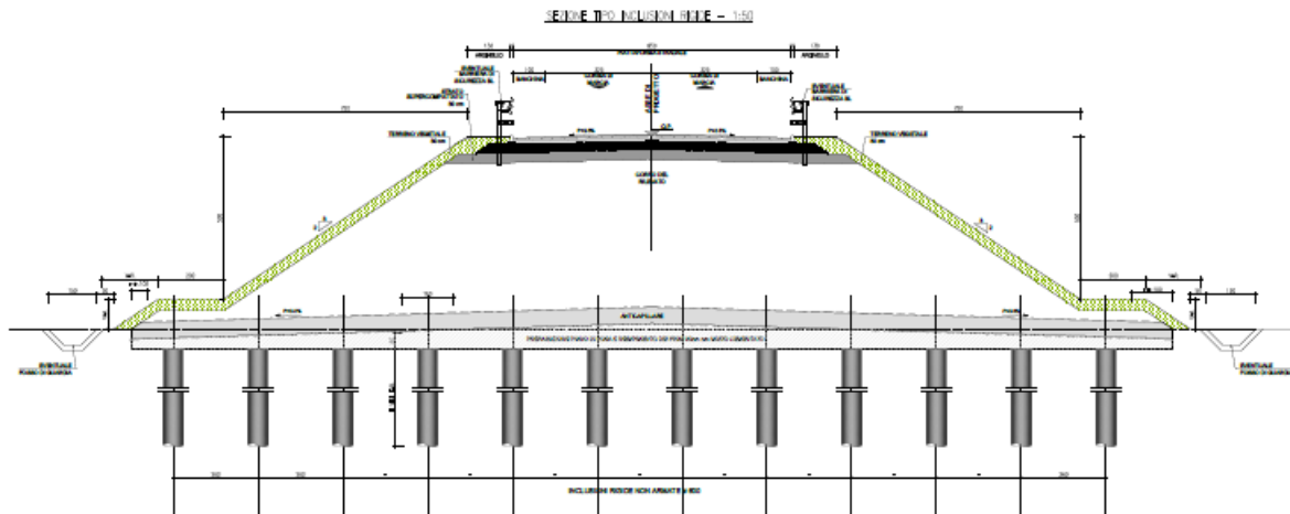
Figura 3.1 – Sezione tipo del rilevato di approccio spalla A con inclusioni rigide
