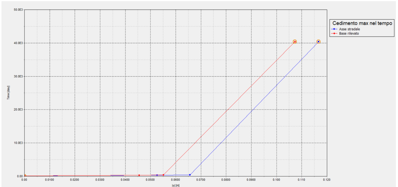
Figura 9.1.2.2: Rilevato sez. A2 – Spostamenti totali in corrispondenza sia dell'asse stradale che della base del rilevato
