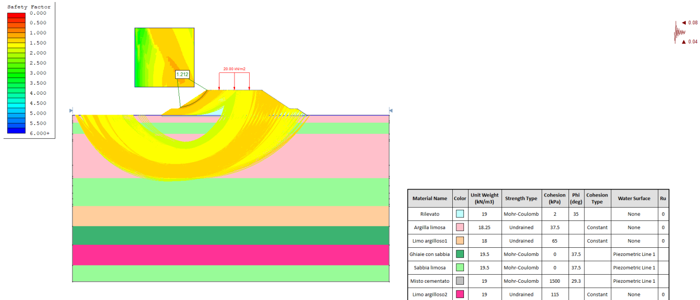
Figura 8.1.4: Spalla B: Rilevato H=7 m, - Analisi di stabilità globale in campo sismico
