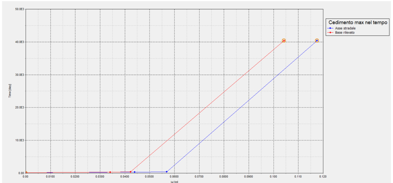
Figura 9.1.4.2: Rilevato sez. B2 – Spostamenti totali in corrispondenza sia dell'asse stradale che della base del rilevato
