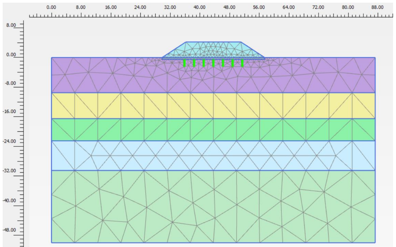
Figura 9.1.2.1: Modello rilevato sezione A2
