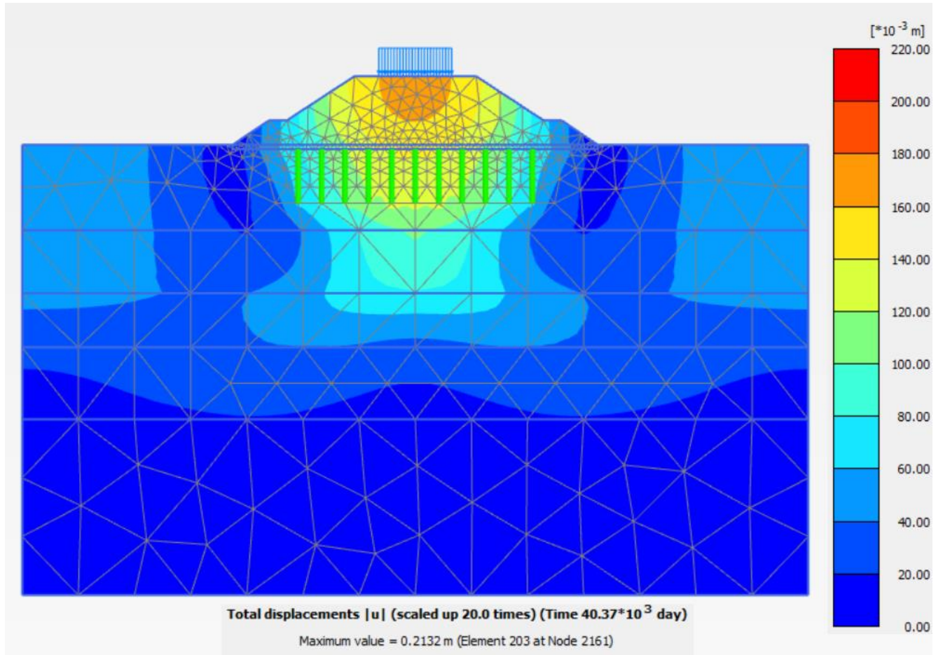
Figura 9.1.1.4: Rilevato sez. A1 - Spostamenti totali lungo termine
