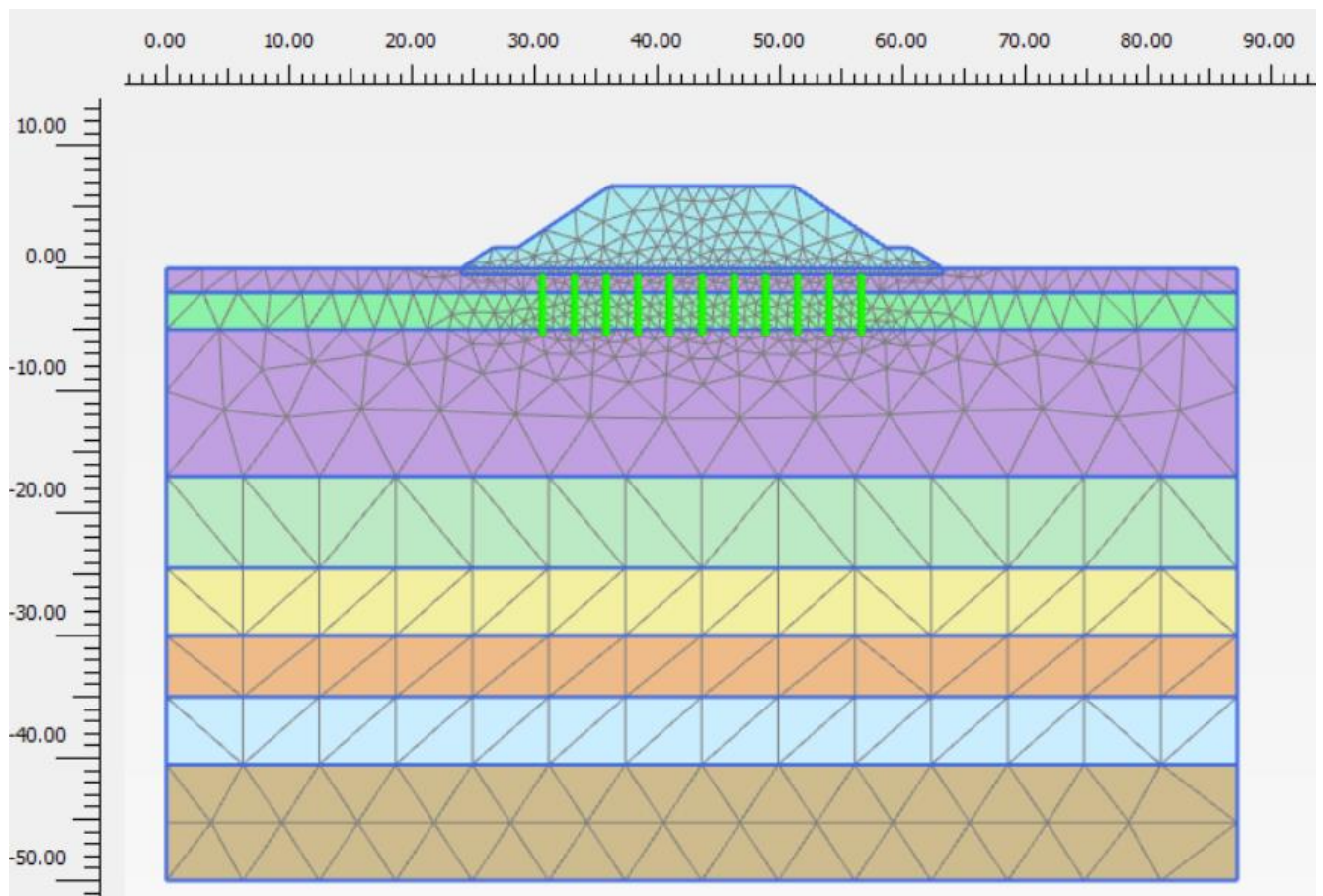
Figura 9.1.3.1: Modello rilevato sezione B1
