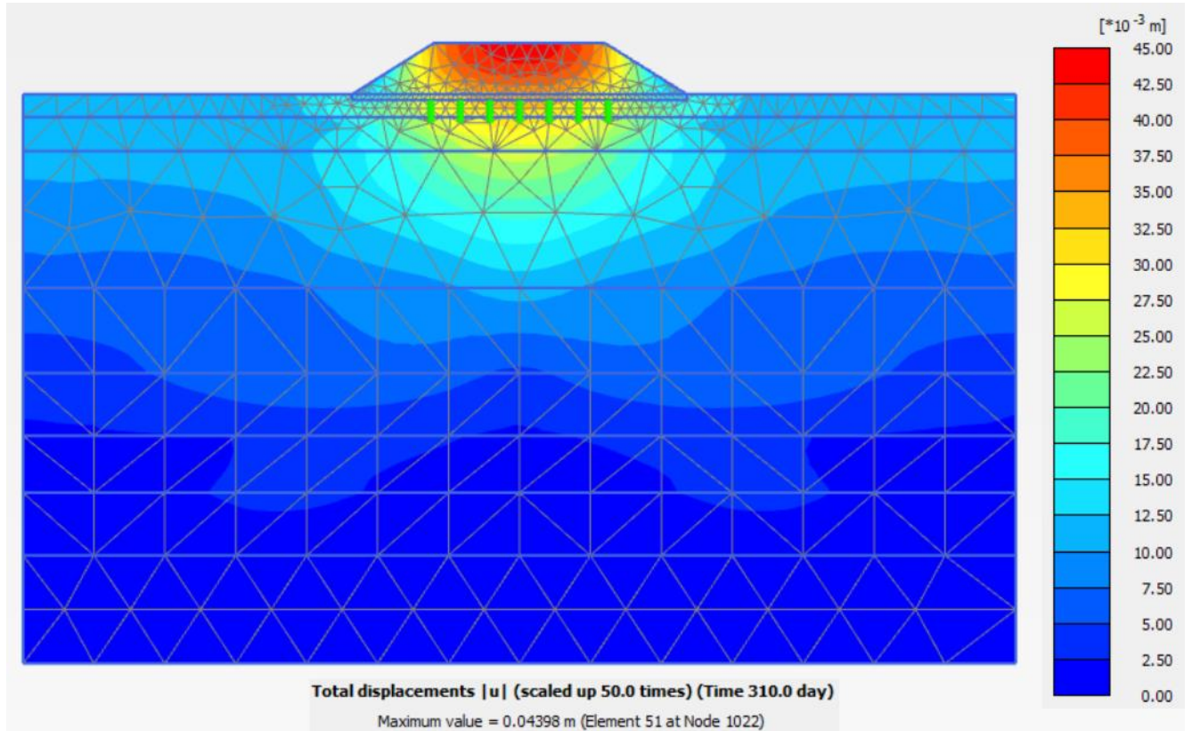
Figura 9.1.4.3: Rilevato sez. B2 – Spostamenti totali termine costruzione
