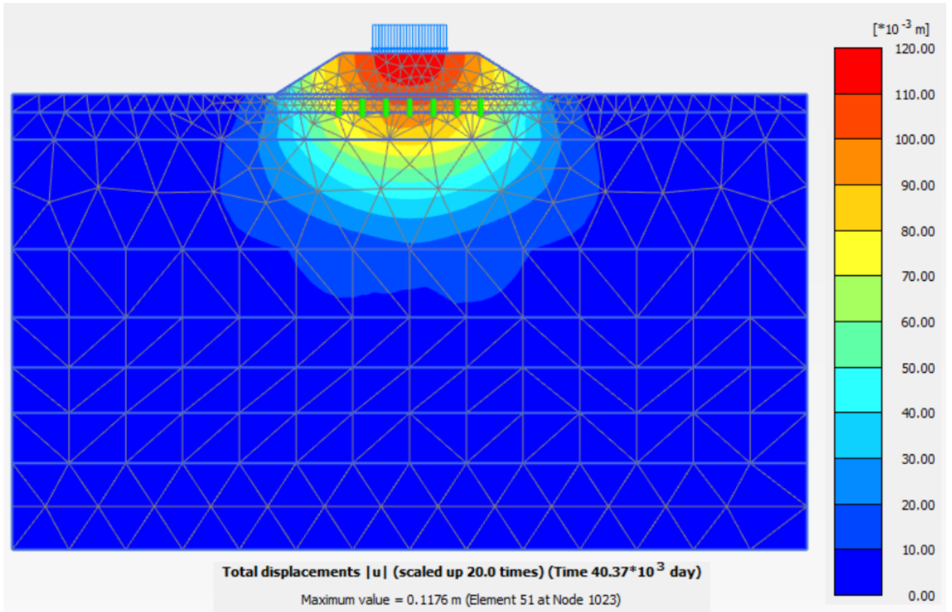
Figura 9.1.4.4: Rilevato sez. B2 – Spostamenti totali lungo termine
