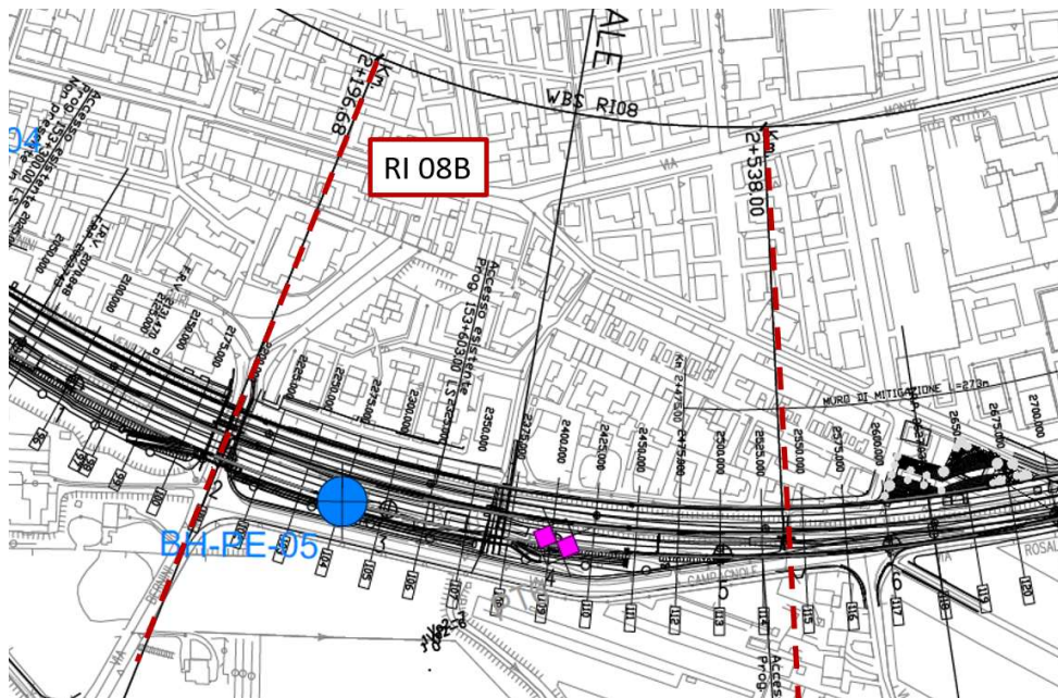
Figura 3 - Planimetria Rilevato RI08B, estratta dalla Planimetria Generale (Doc. Rif. [3])
