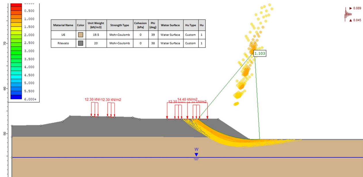
Figura 14 - Rilevato H=4.50 m (da pk 2+196 a pk 2+538) - Analisi SLU in campo sismico
