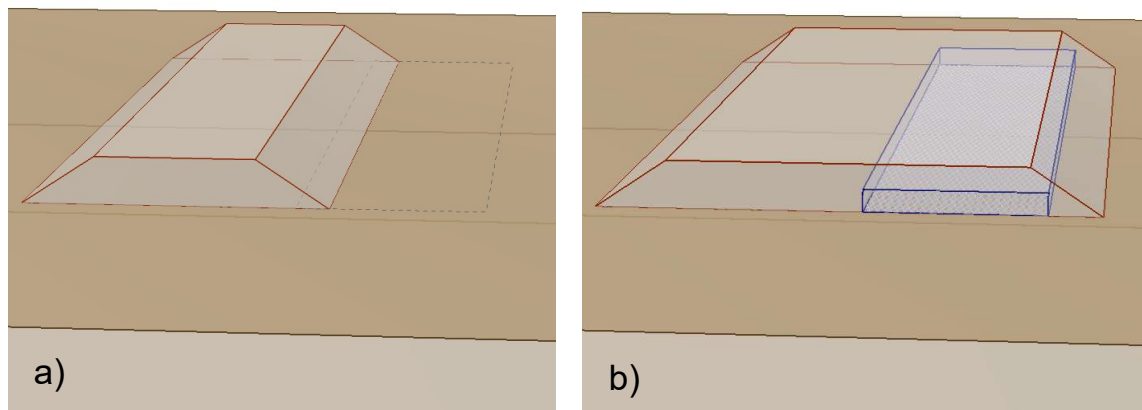
Figura 17 - Rilevato H=4.50 m (da pk 2+196 a pk 2+538) - Analisi SLE – Modello di calcolo
