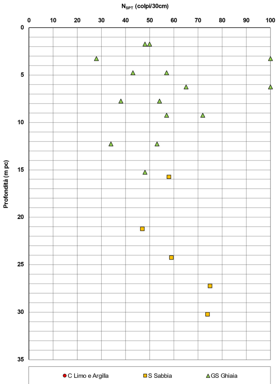
Figura 5 – Esito delle prove SPT tra pk 2+538,00 a pk 3+160,00
