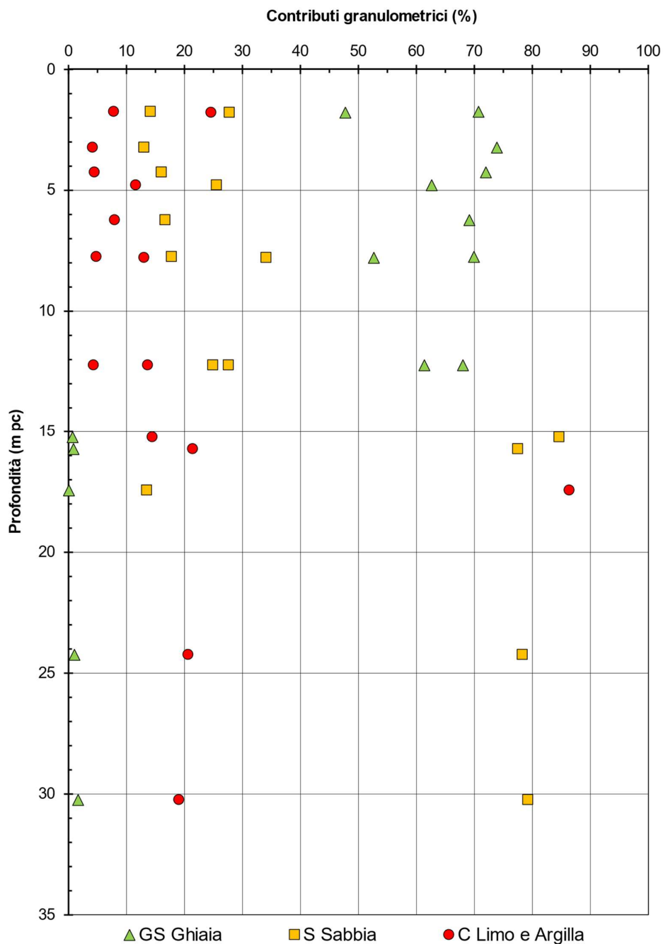
Figura 4 – Sintesi analisi granulometriche tra pk 2+538,00 a pk 3+160,00
