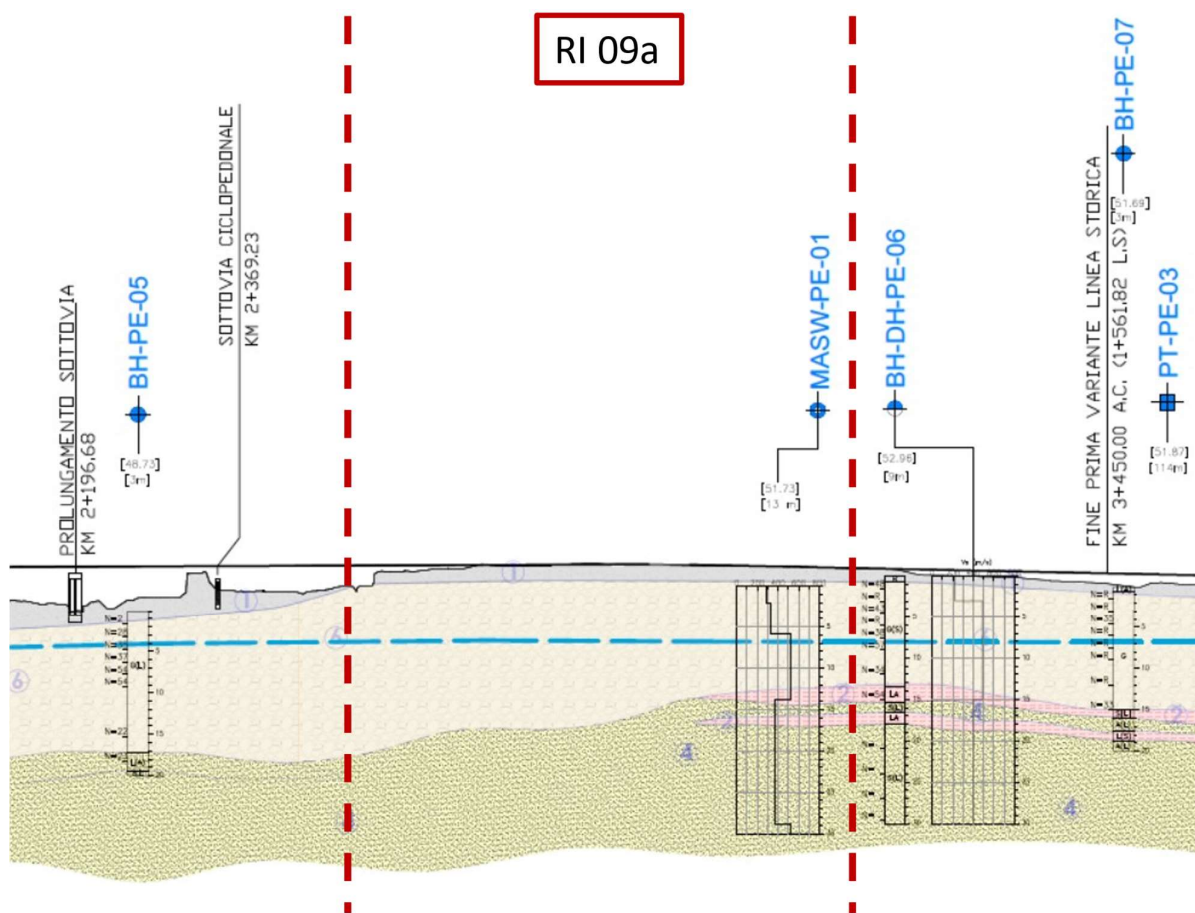
Figura 2 - Profilo Geotecnico Rilevato RI09a, estratto dal Profilo Geotecnico Generale (Doc. Rif. [3])
