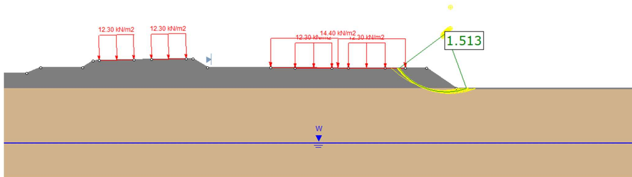
Figura 15 - Rilevato H=1.50 m (da pk 2+538 a pk 3+160) - Analisi SLU in campo sismico
