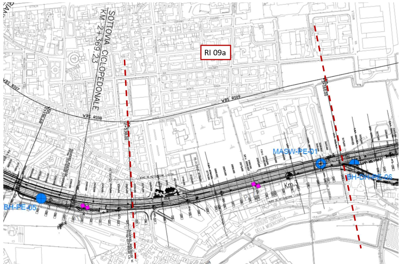
Figura 3 - Planimetria Rilevato RI09a, estratto dalla Planimetria Generale (Doc. Rif. [3])
