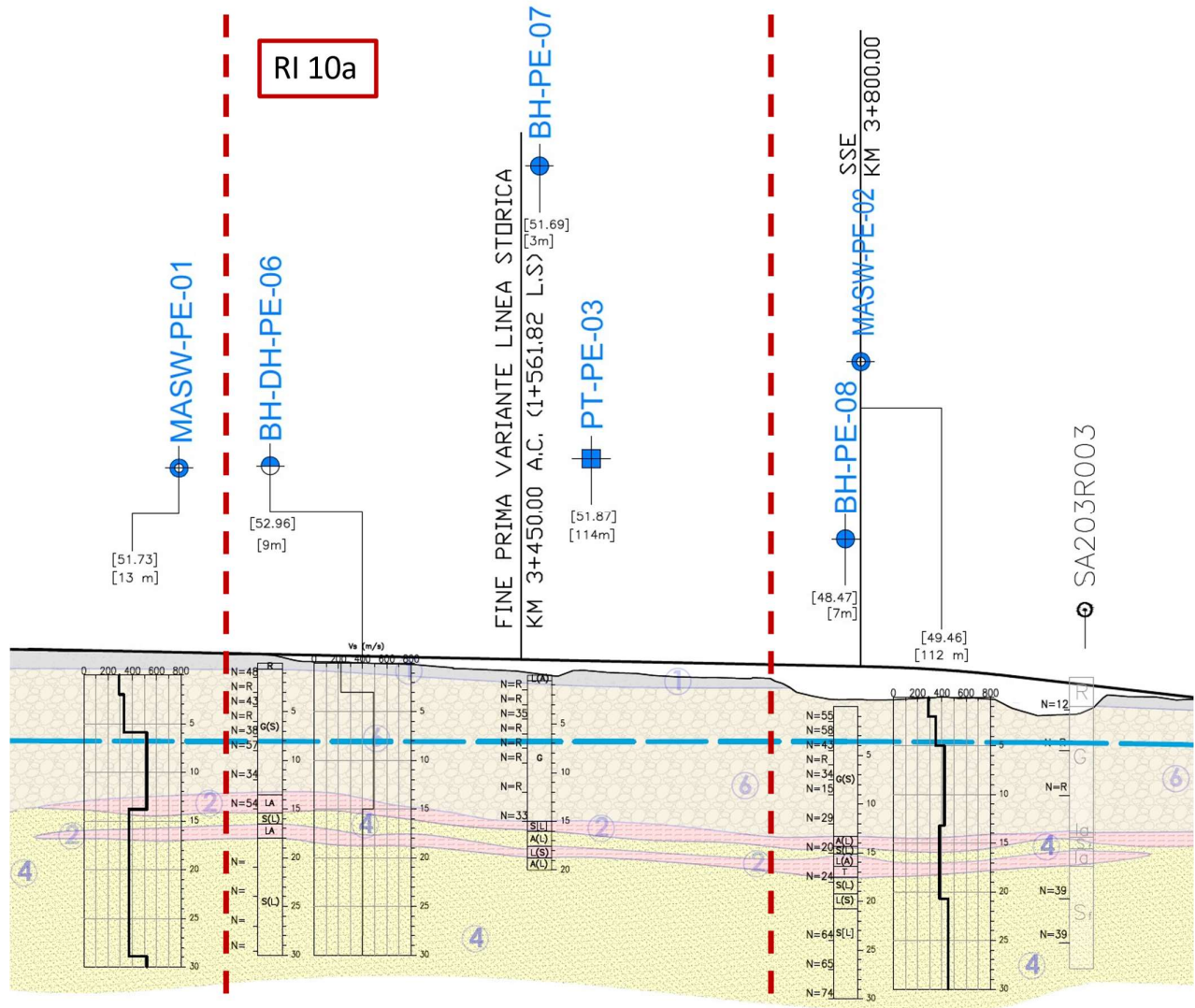
Figura 2 - Profilo Geotecnico Rilevato RI10a, estratto dal Profilo Geotecnico Generale (Doc. Rif. [3])
