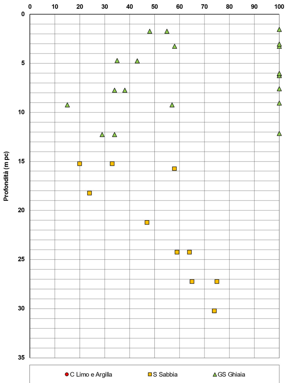
Figura 5 – Esito delle prove SPT tra pk 3+160 a pk 3+700
