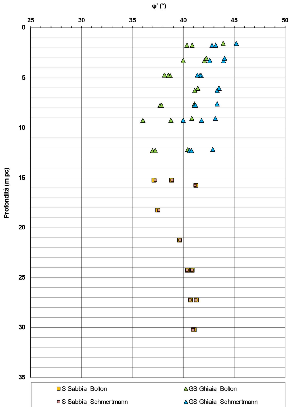
Figura 7 – Angoli di attrito da prove SPT tra pk 3+160 a pk 3+700
