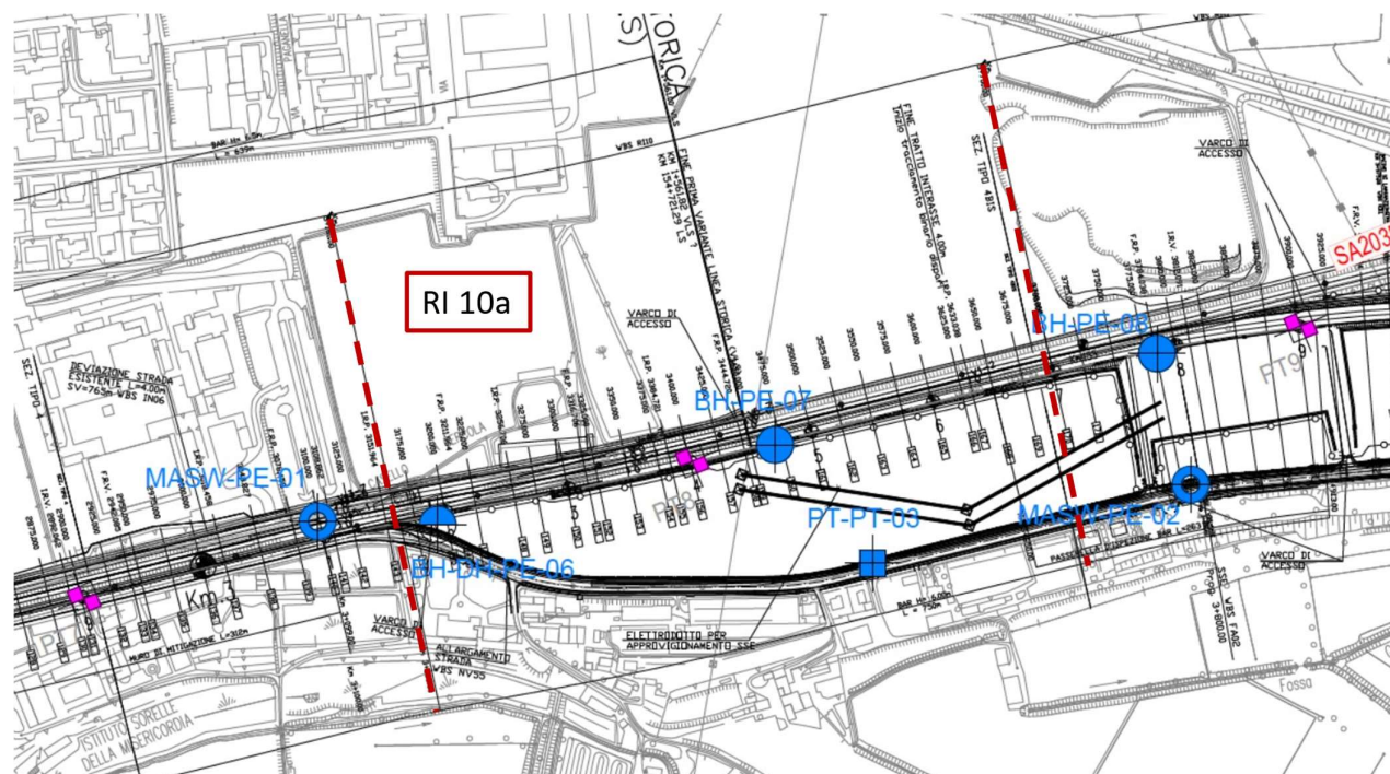
Figura 3 - Planimetria Rilevato RI10a, estratta dalla Planimetria Generale (Doc. Rif. [3])
