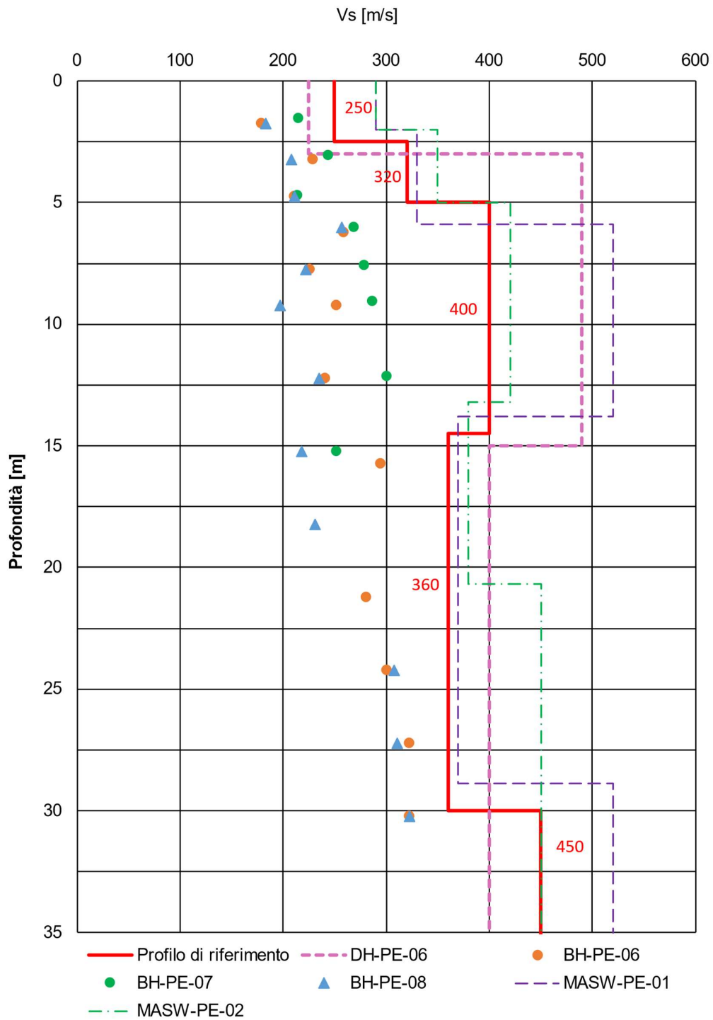
Figura 8 – Profilo di Vs di riferimento, a confronto con dati di correlazioni con SPT e prove geofisiche tipo MASW tra pk 3+160 e 3+700
