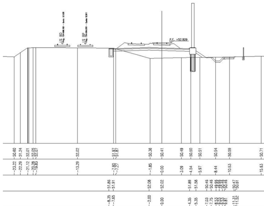
Figura 1 – Sezione di riferimento A (pk 3+700, n. 181) estratta da sezioni PE (Doc Rif. [1])
