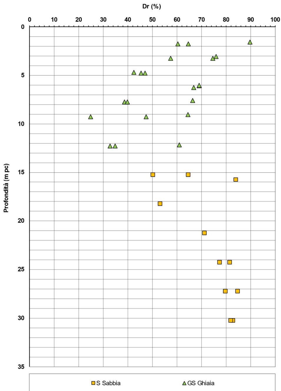
Figura 6 – Densità relativa da prove SPT tra pk 3+160 a pk 3+700
