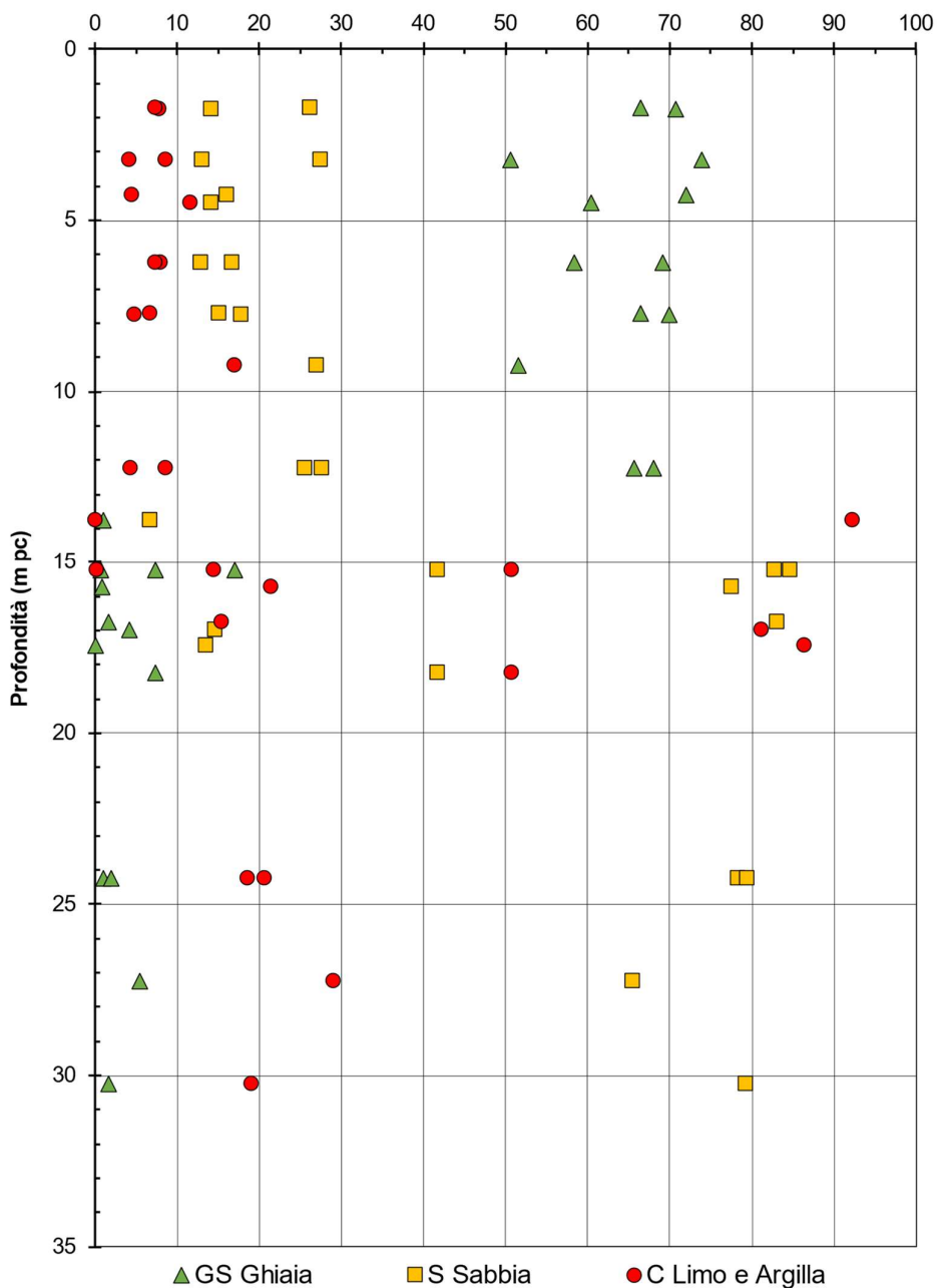
Figura 4 – Sintesi analisi granulometriche tra pk 3+160 a pk 3+700
