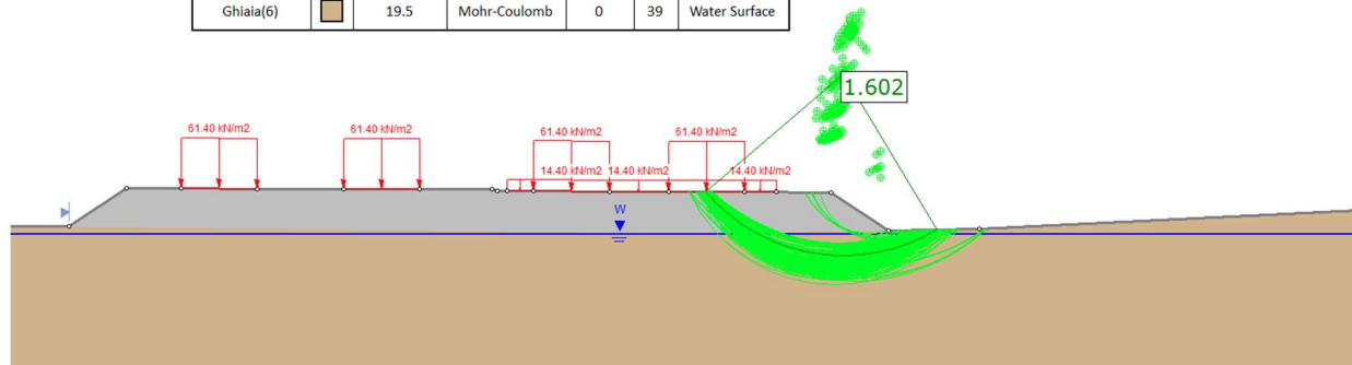
Figura 15 - Rilevato H=1.70 m (da pk 3+160 a pk 3+700) - Analisi SLU in campo statico DA1C2
