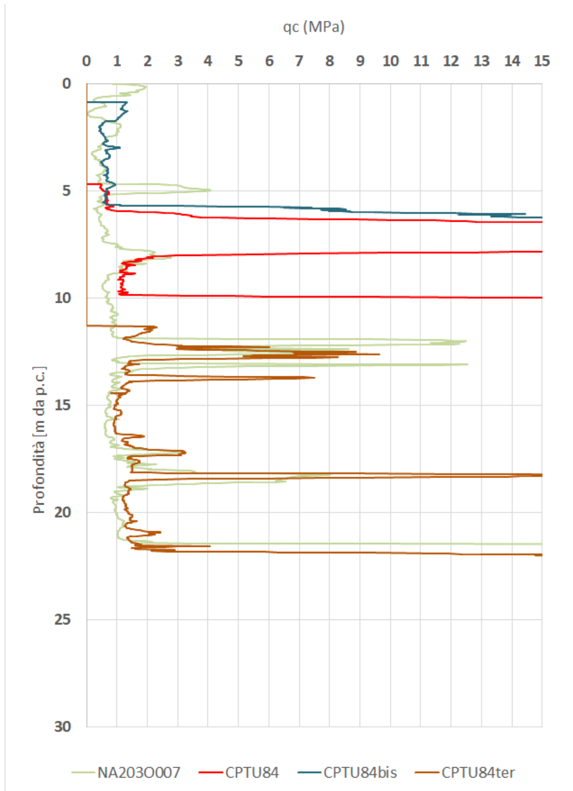
Figura 5 – Prove CPTU nell'area dell'RI56
