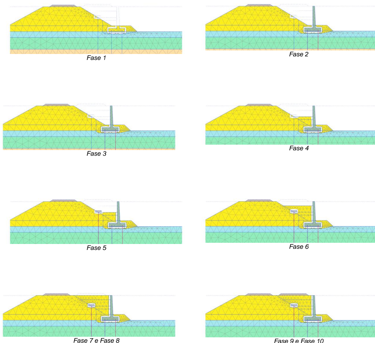
Figura 22 – RI56: fasi della modellazione a elementi finiti
