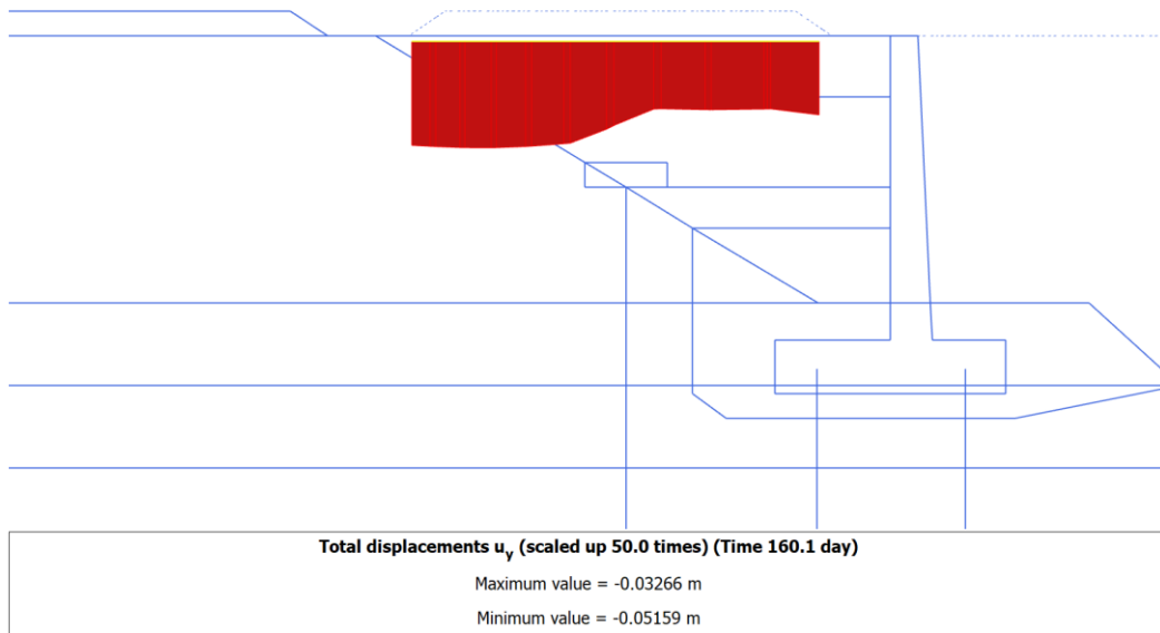
Figura 24 – RI56: Cedimenti totali prima della posa del ballast
