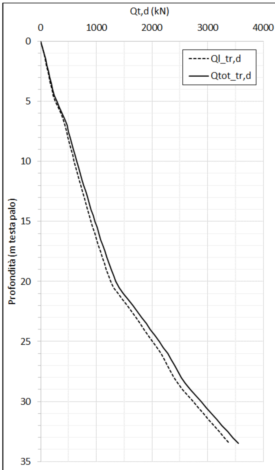
Figura 36 – Curve di capacità portante SLU, trazione per pali D=1000 mm
