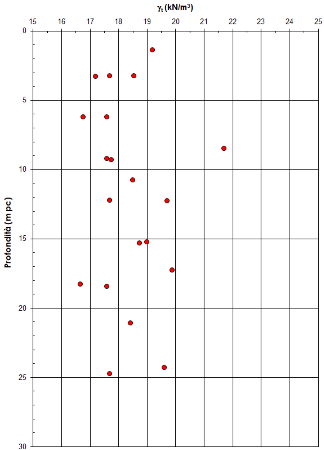
Figura 8 –Peso di volume dei campioni di terreno a grana fine nell'area di interesse.
