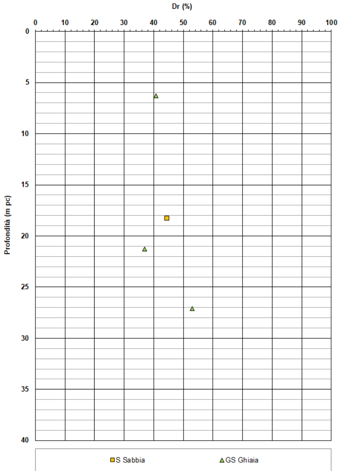
Figura 11 – Densità relativa da prove SPT da pk 30+640,00 a pk 30+940,00
