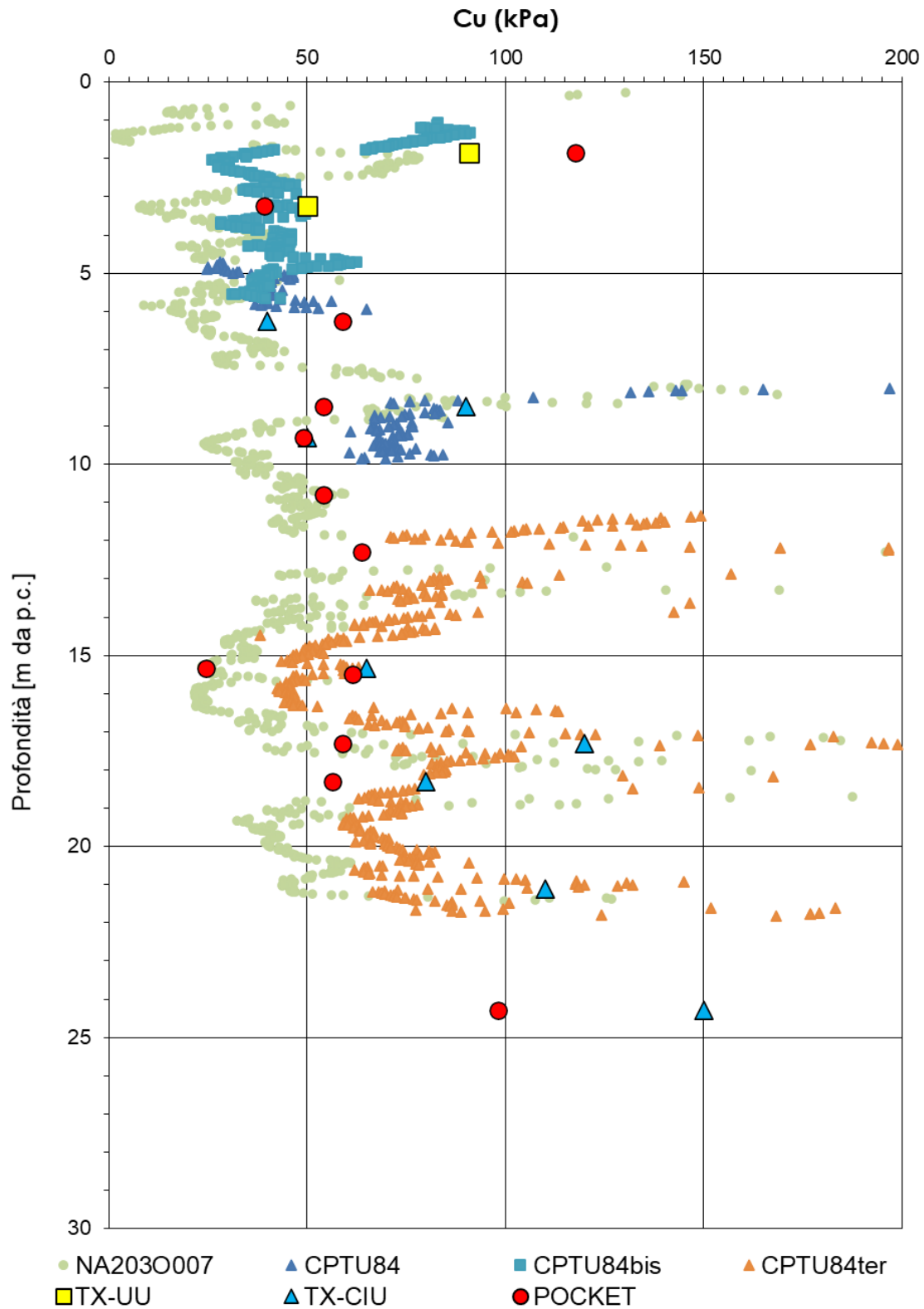
Figura 9 – Resistenza in condizioni non drenate da prove CPTU disponibili nell'intorno della WBS
