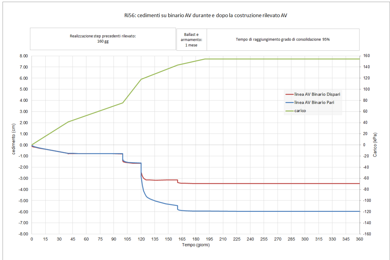
Figura 28 – RI56: Sviluppo nel tempo dei cedimenti totali alla base del rilevato di progetto (linee rossa e blu) in funzione del carico alla base del rilevato (linea verde) Cedimento a partire dalla realizzazione del ballast: \Delta u_y = 5 \text{ mm}
