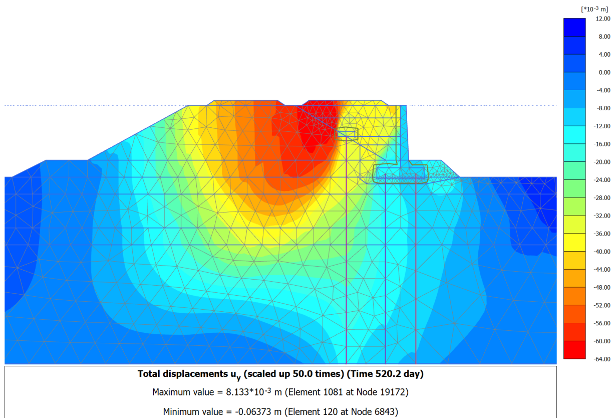
Figura 23 – RI56: Cedimenti totali al termine della costruzione del rilevato ferroviario AV
