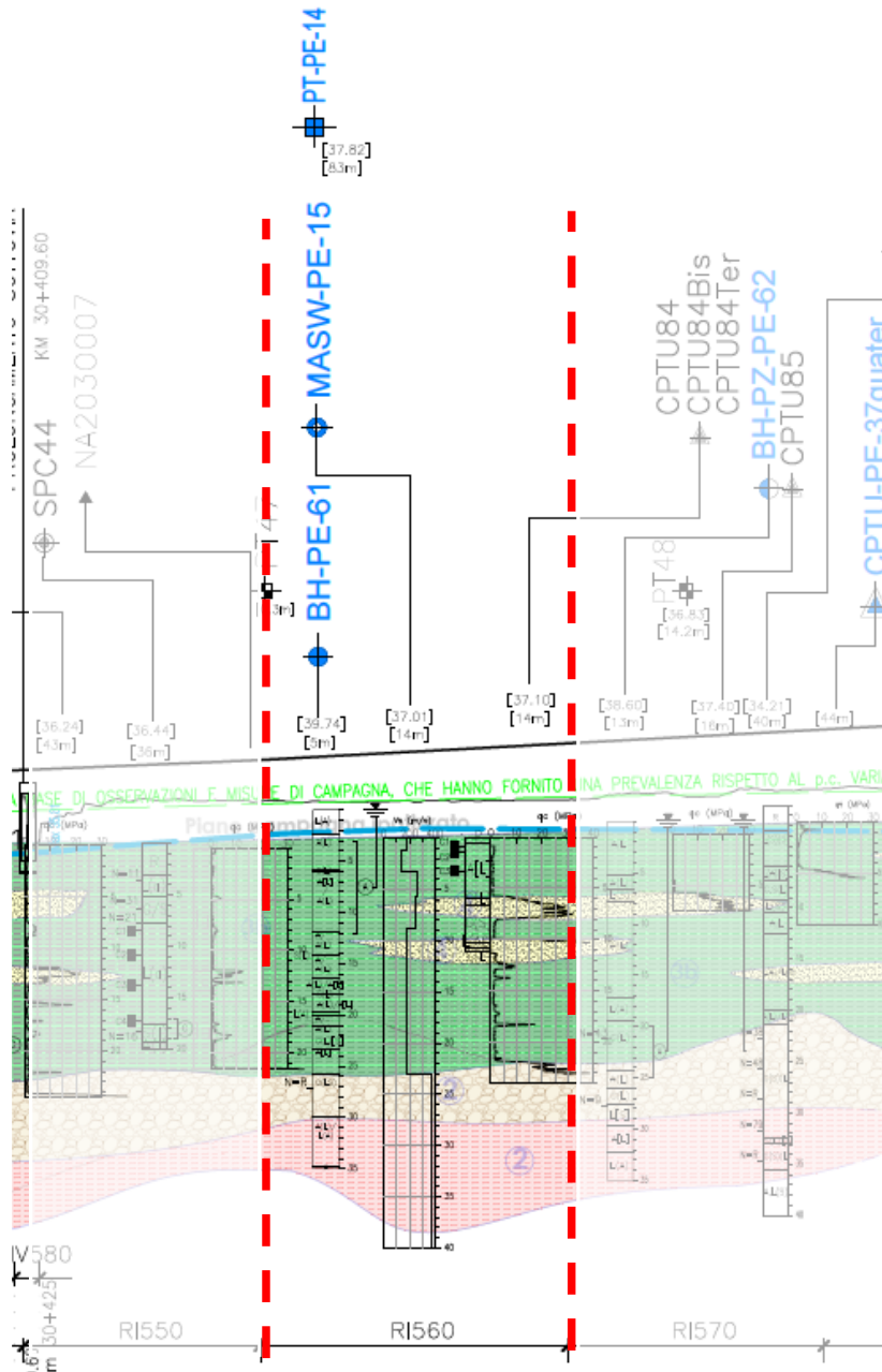
Figura 4 - Profilo Geotecnico Rilevato RI56, estratto dal Profilo Geotecnico Generale (Doc. Rif. [3])
