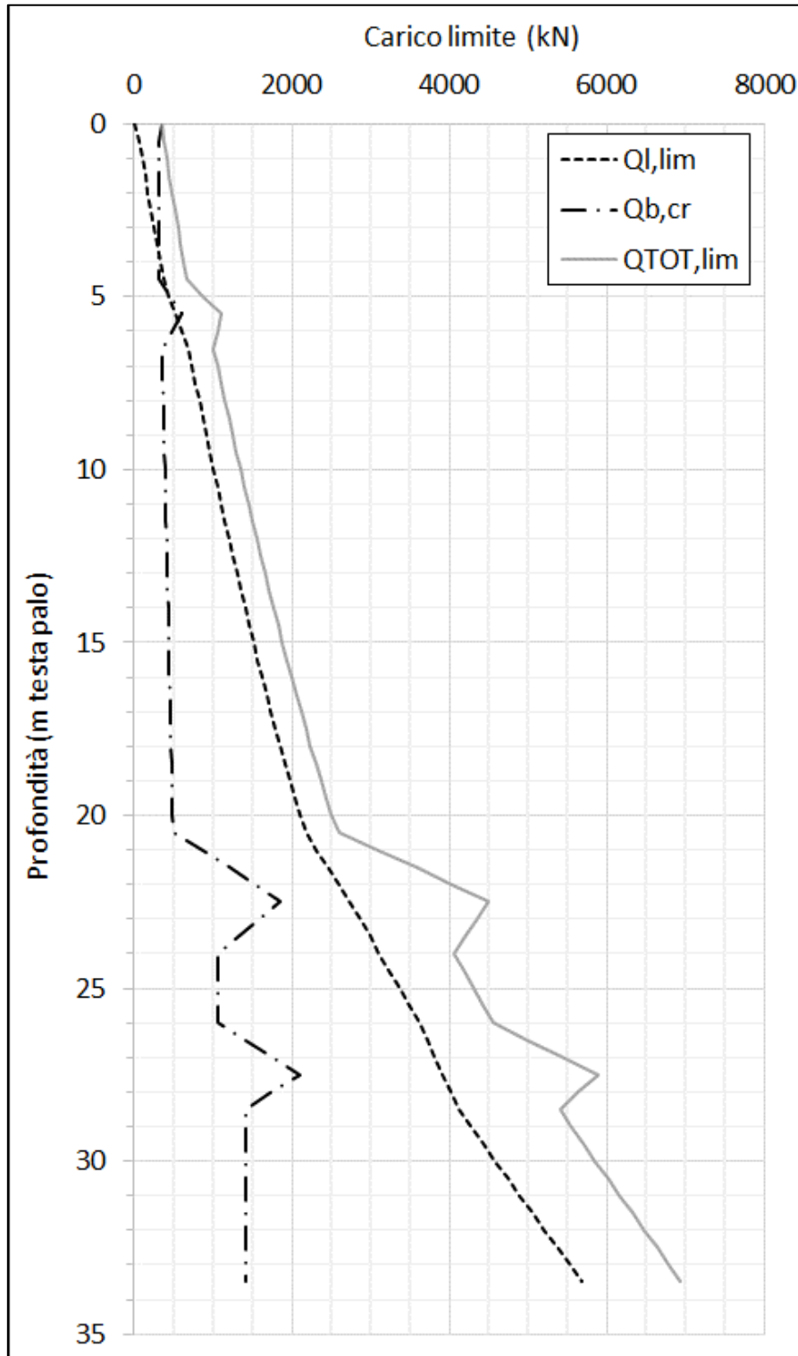
Figura 32 – Curve di Carico Limite Ultimo per pali D=1000 mm
