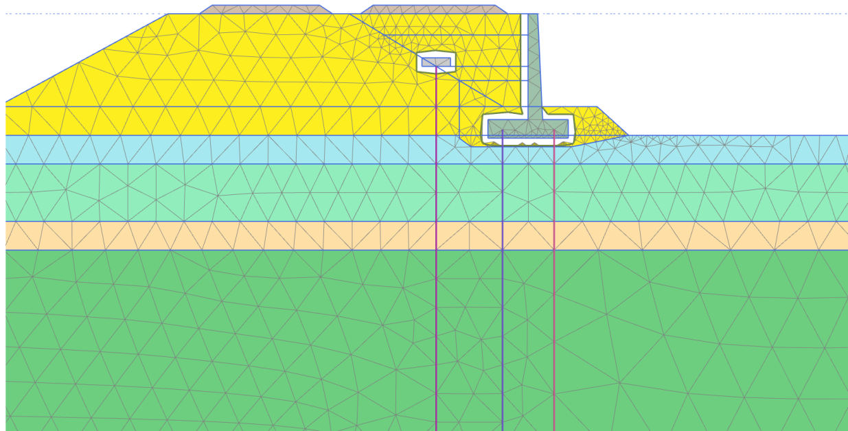
Figura 21 – RI56: modello agli elementi finiti
