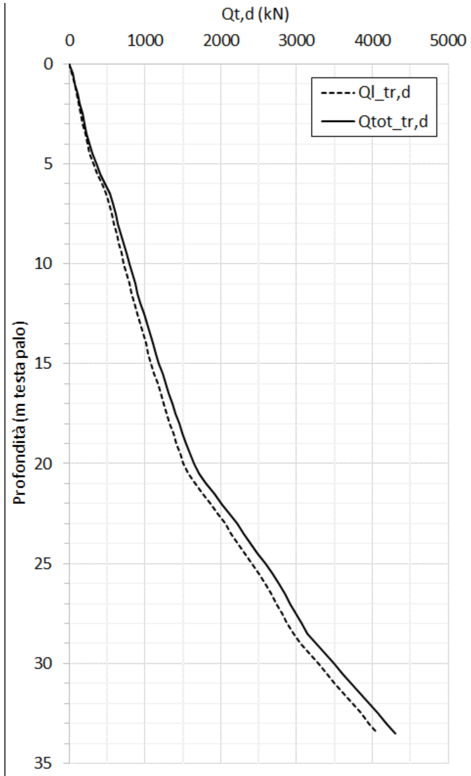
Figura 37 – Curve di capacità portante SLU, trazione per pali D=1200 mm
