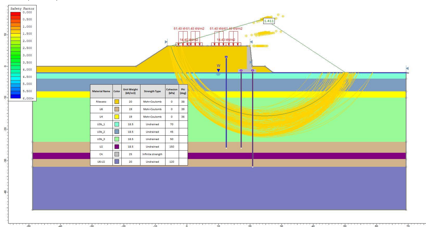
Figura 18 – Rilevato RI56 - Analisi SLU in campo statico DA1C2
