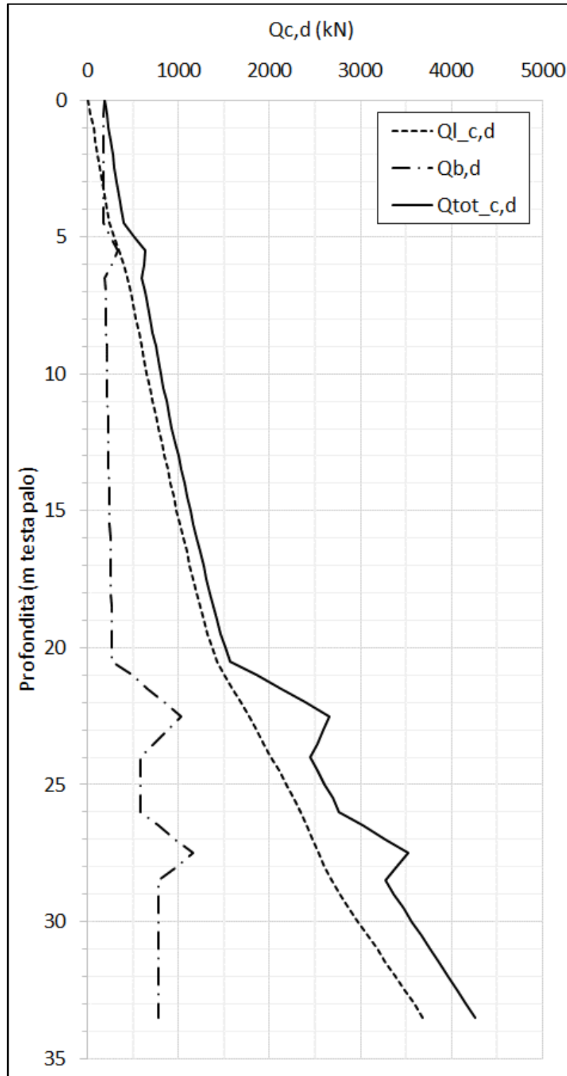
Figura 34 – Curve di capacità portante SLU, compressione per pali D=1000 mm
