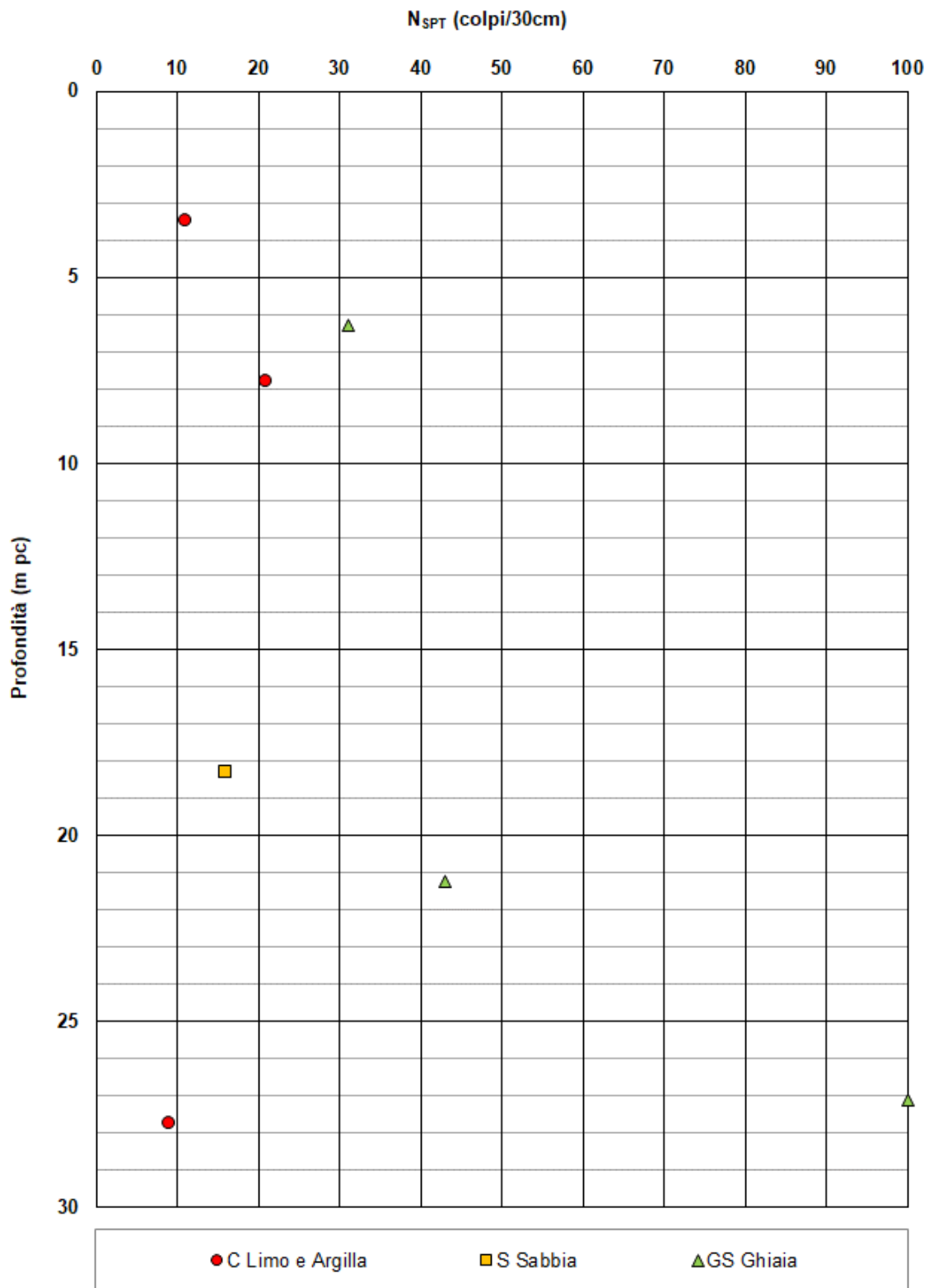
Figura 10 – Esito delle prove SPT da pk 30+640,00 a pk 30+940,00
