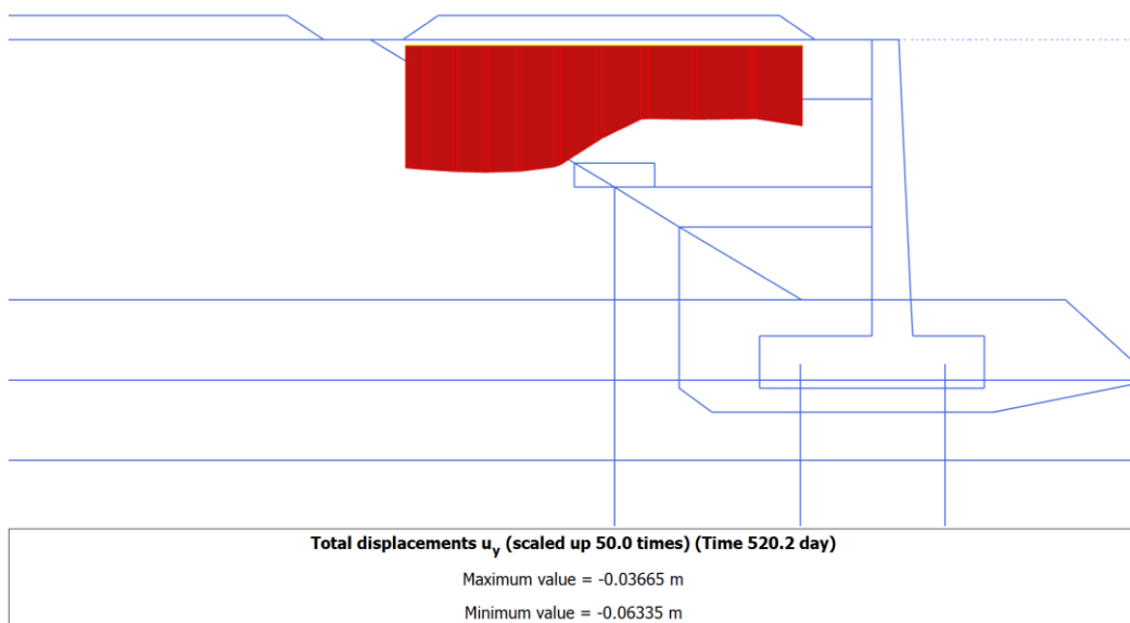
Figura 25 – RI56: Cedimenti totali di lungo termine: al termine della consolidazione
