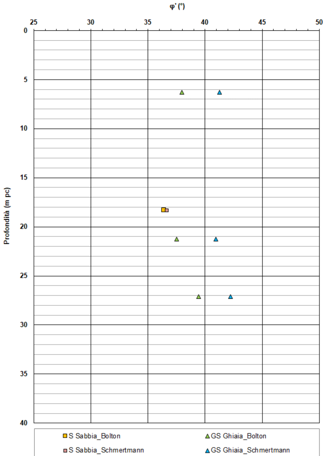
Figura 12 – Angoli di resistenza al taglio da prove SPT da pk 30+640,00 a pk 30+940,00
