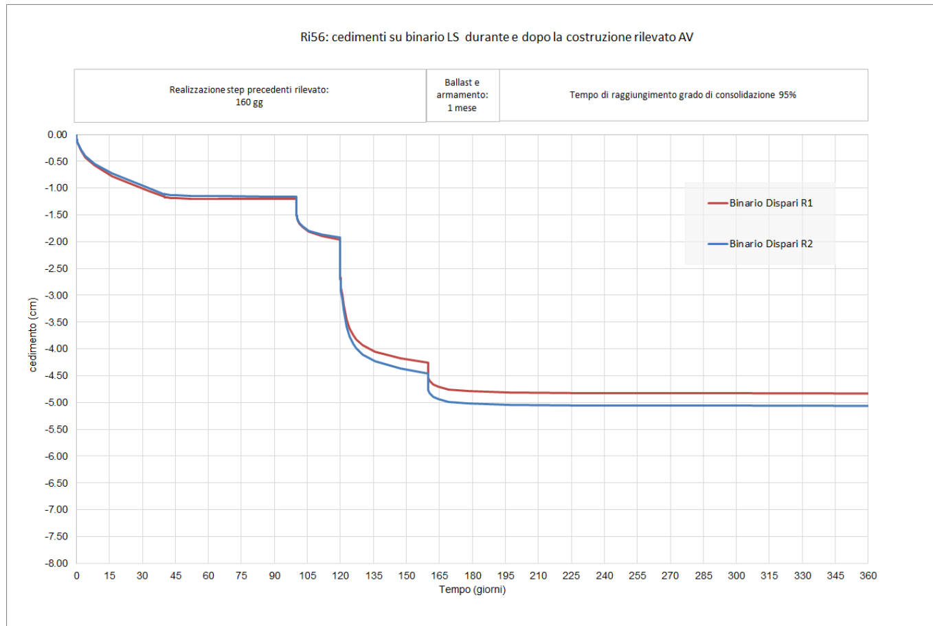
Figura 27 – Ri56: Sviluppo nel tempo dei cedimenti totali sul Binario Dispari della Linea Storica cedimento differenziale tra le rotaie \Delta u_y = 3.0 \text{ mm}
