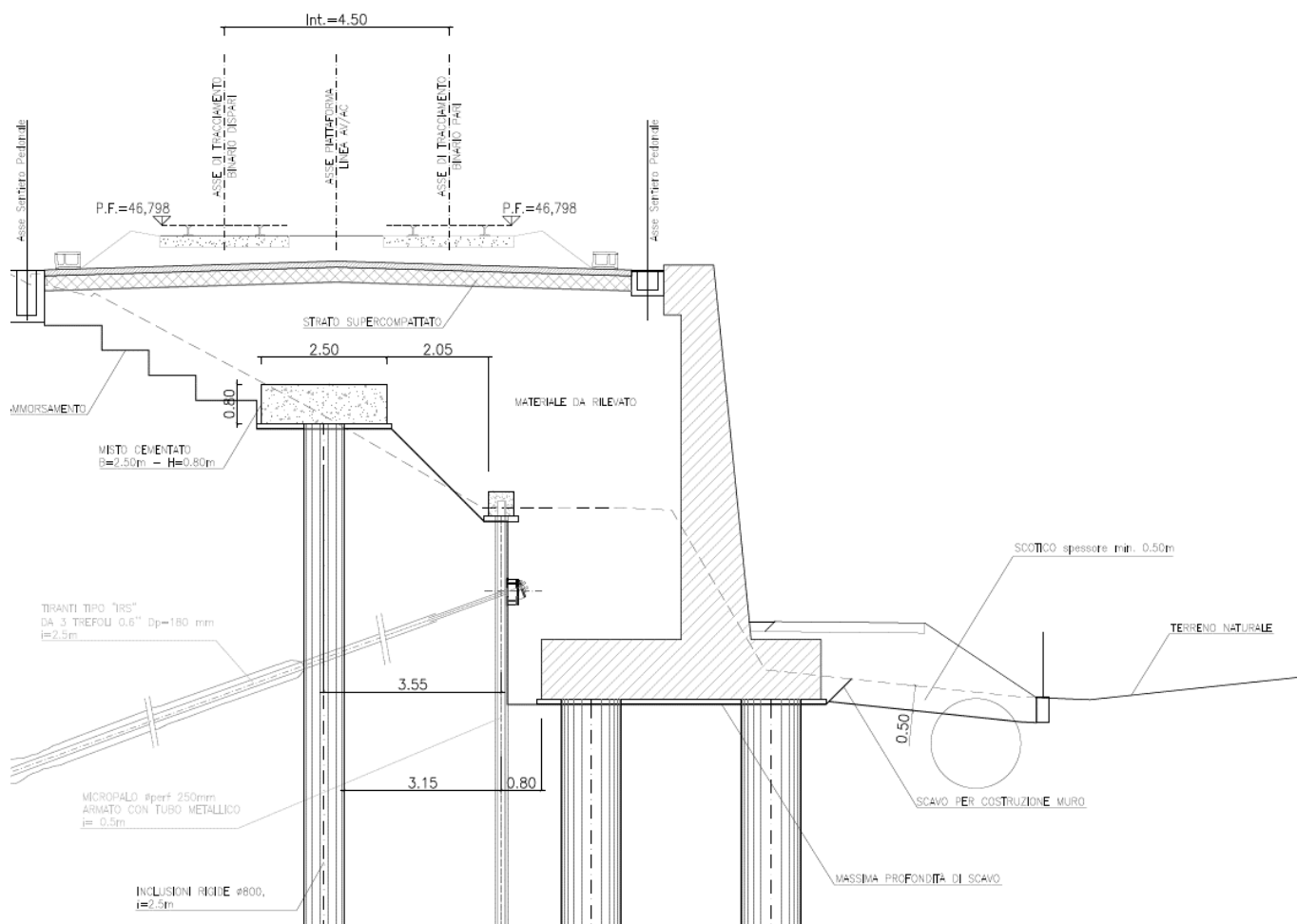
Figura 2 – Schema in sezione degli interventi
