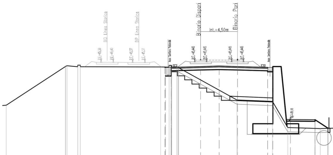
Figura 1 – Sezione di riferimento (pk 30+775,00 n. RI56-7) estratta da sezioni PE (Doc Rif. [1])
