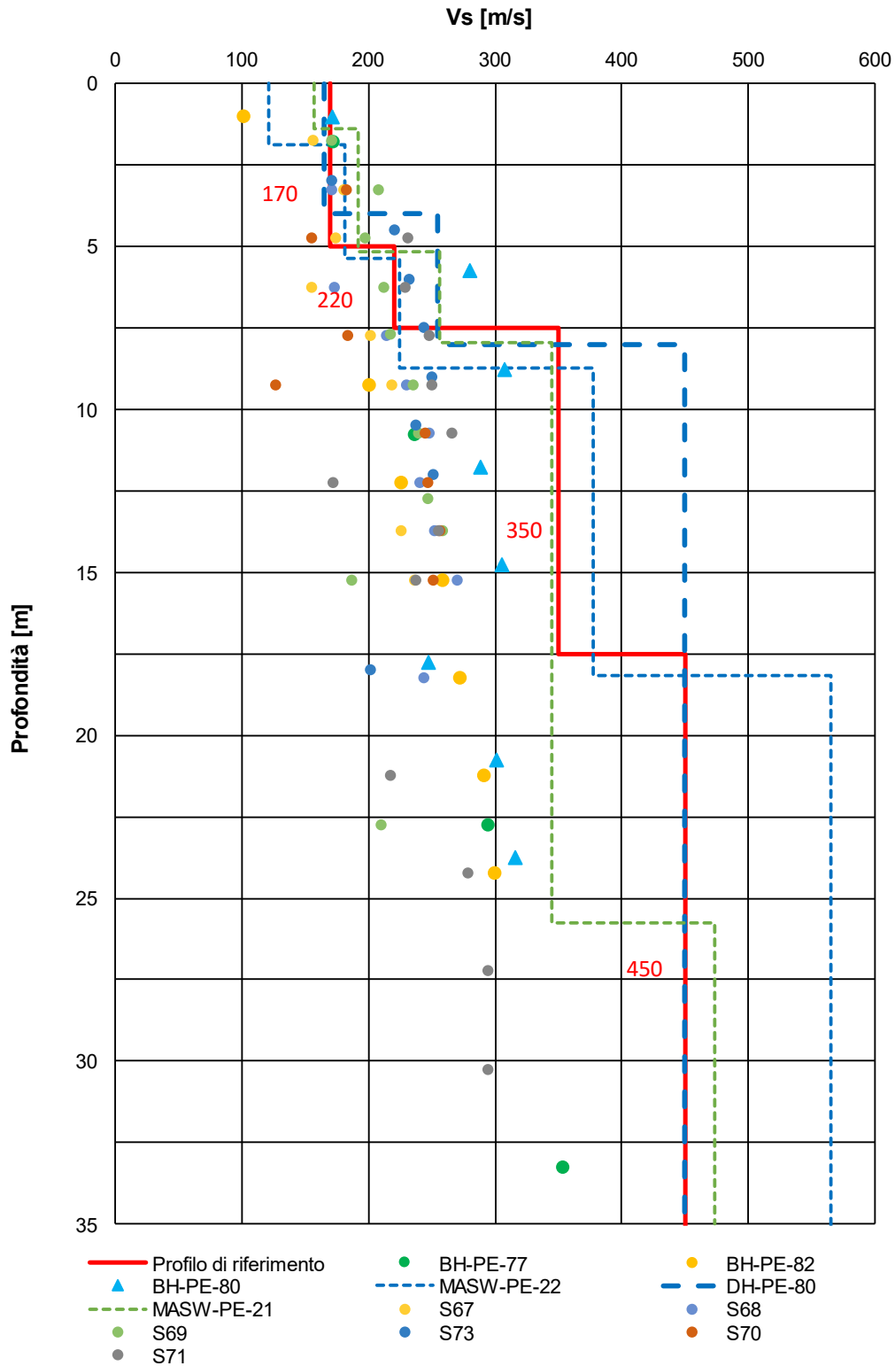
Figura 8 – Profilo di vs di riferimento, a confronto con dati di correlazioni con SPT e prove geofisiche tipo MASW tra pk 187+813,55 e pk 188+159,94 della LS
