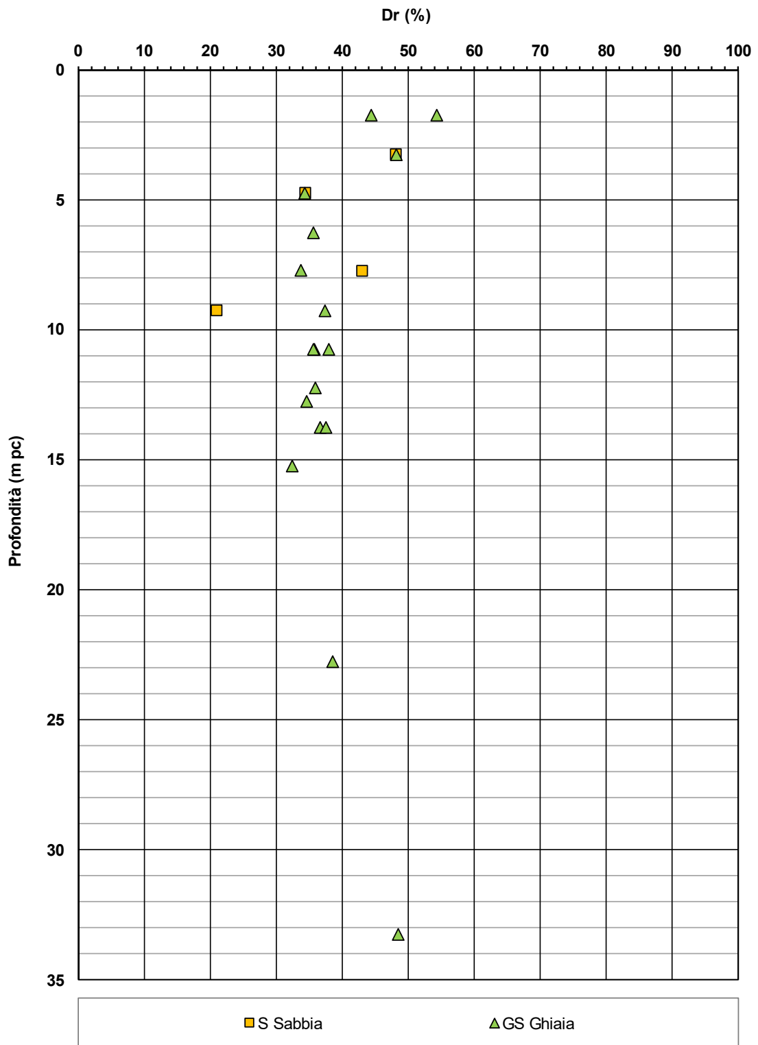
Figura 6 – Densità relativa da prove SPT tra pk 187+813,55 e pk 188+159,94 della LS
