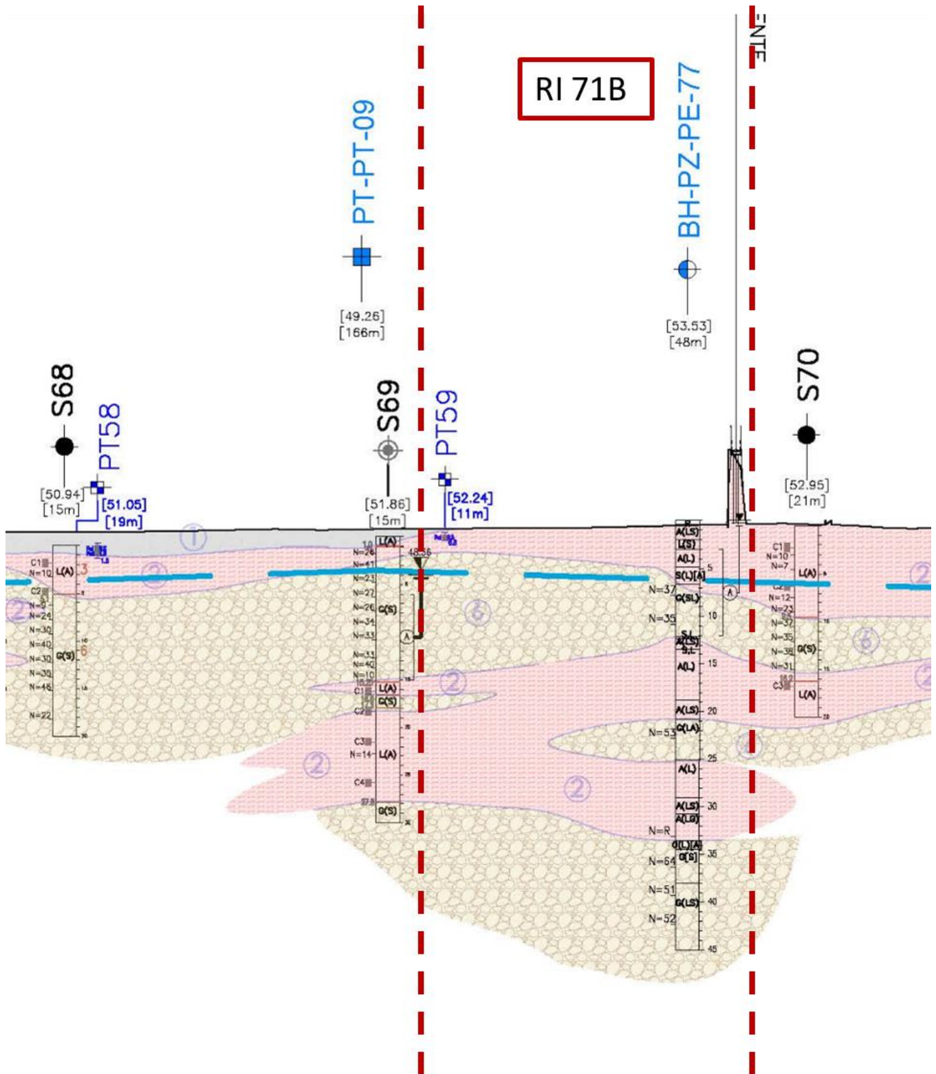
Figura 2 - Profilo Geotecnico Rilevato RI71B, estratto dal Profilo Geotecnico Generale (Doc. Rif. [3])
