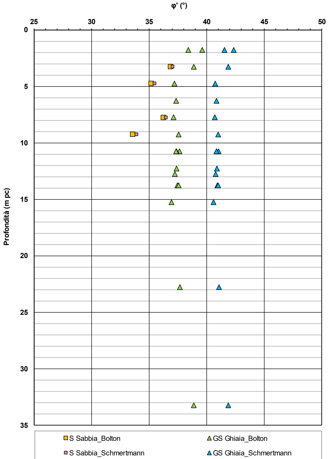
Figura 7 – Angoli di attrito da prove SPT tra pk 187+813,55 e pk 188+159,94 della LS
