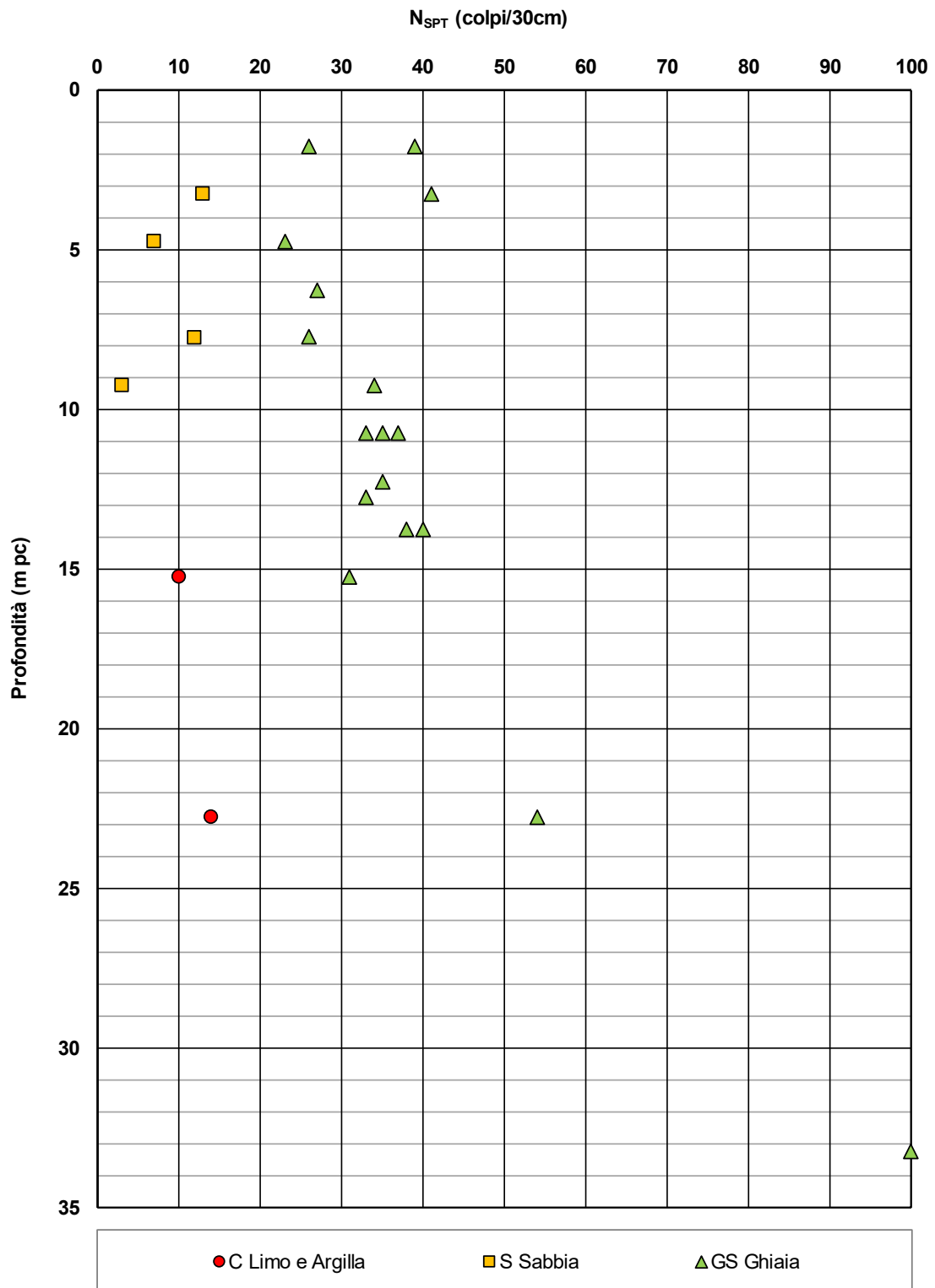
Figura 5 – Esito delle prove SPT tra pk 187+813,55 e pk 188+159,94 della LS
