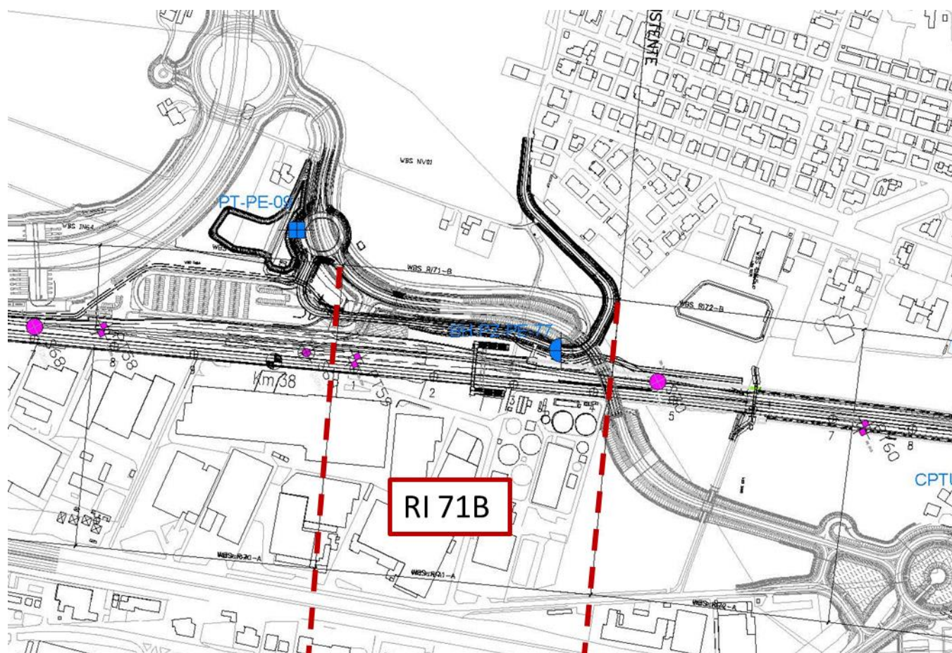
Figura 3 - Planimetria Rilevato RI71B, estratto dalla Planimetria Generale (Doc. Rif. [3])
