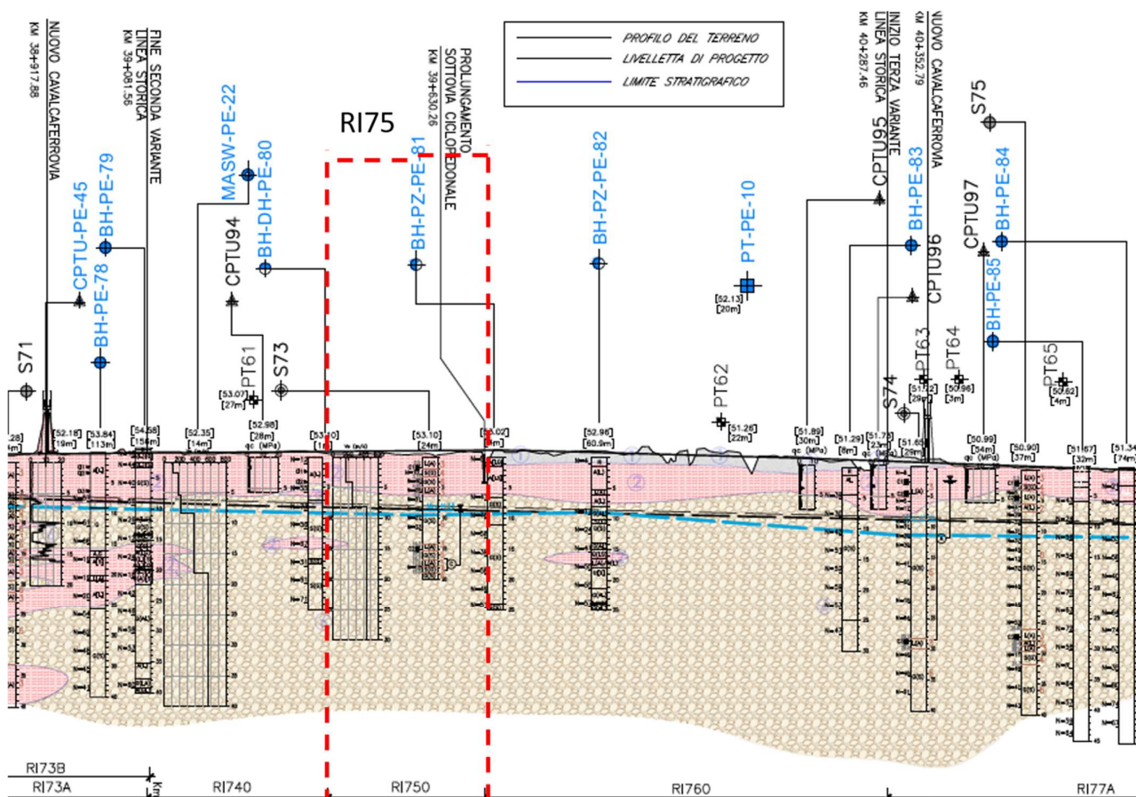
Figura 3 - Profilo Geotecnico Rilevato RI75, estratto dal Profilo Geotecnico Generale
