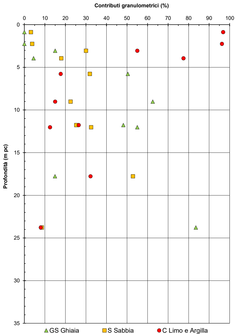
Figura 5 – Sintesi analisi granulometriche – RI75
