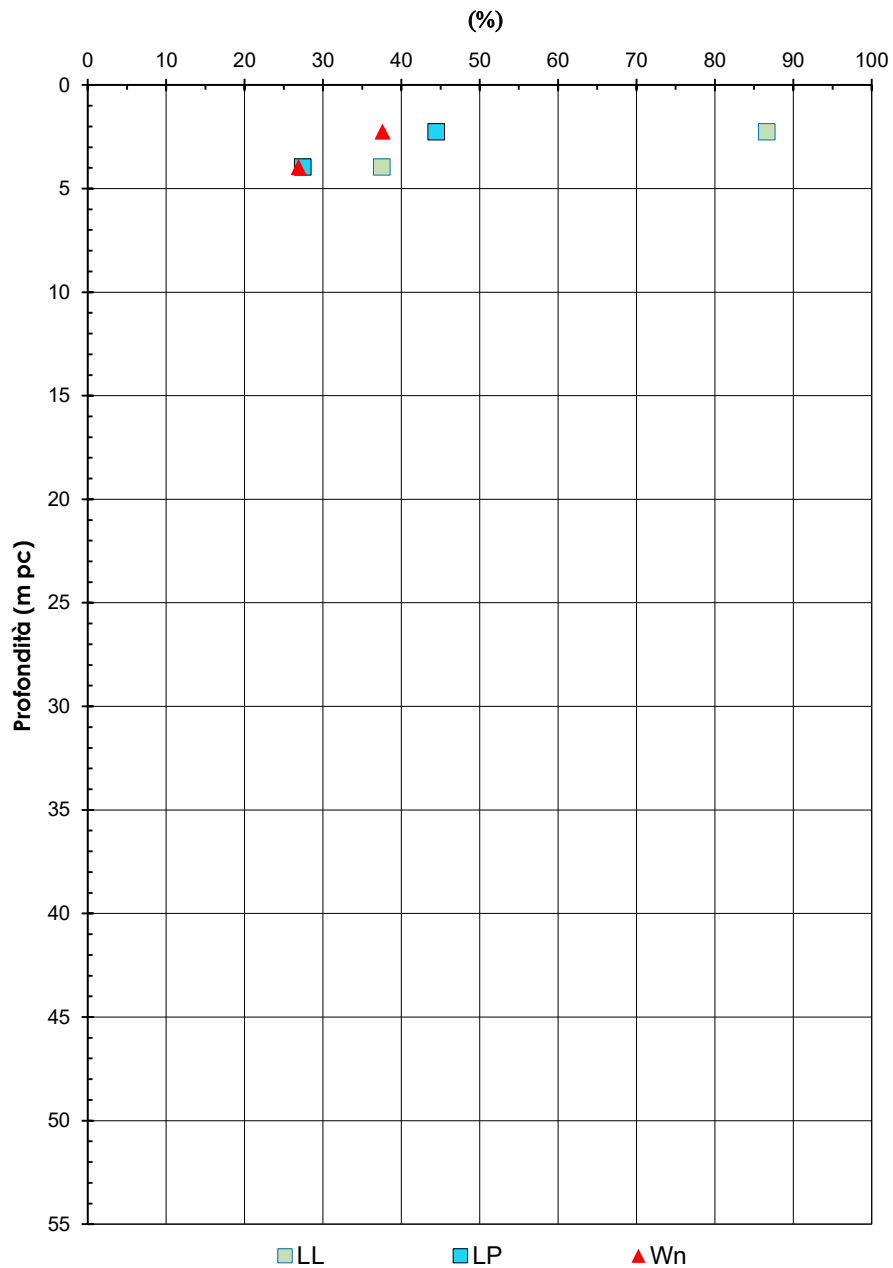
Figura 8 – Contenuto d’acqua, limite liquido e limite plastico – RI75
