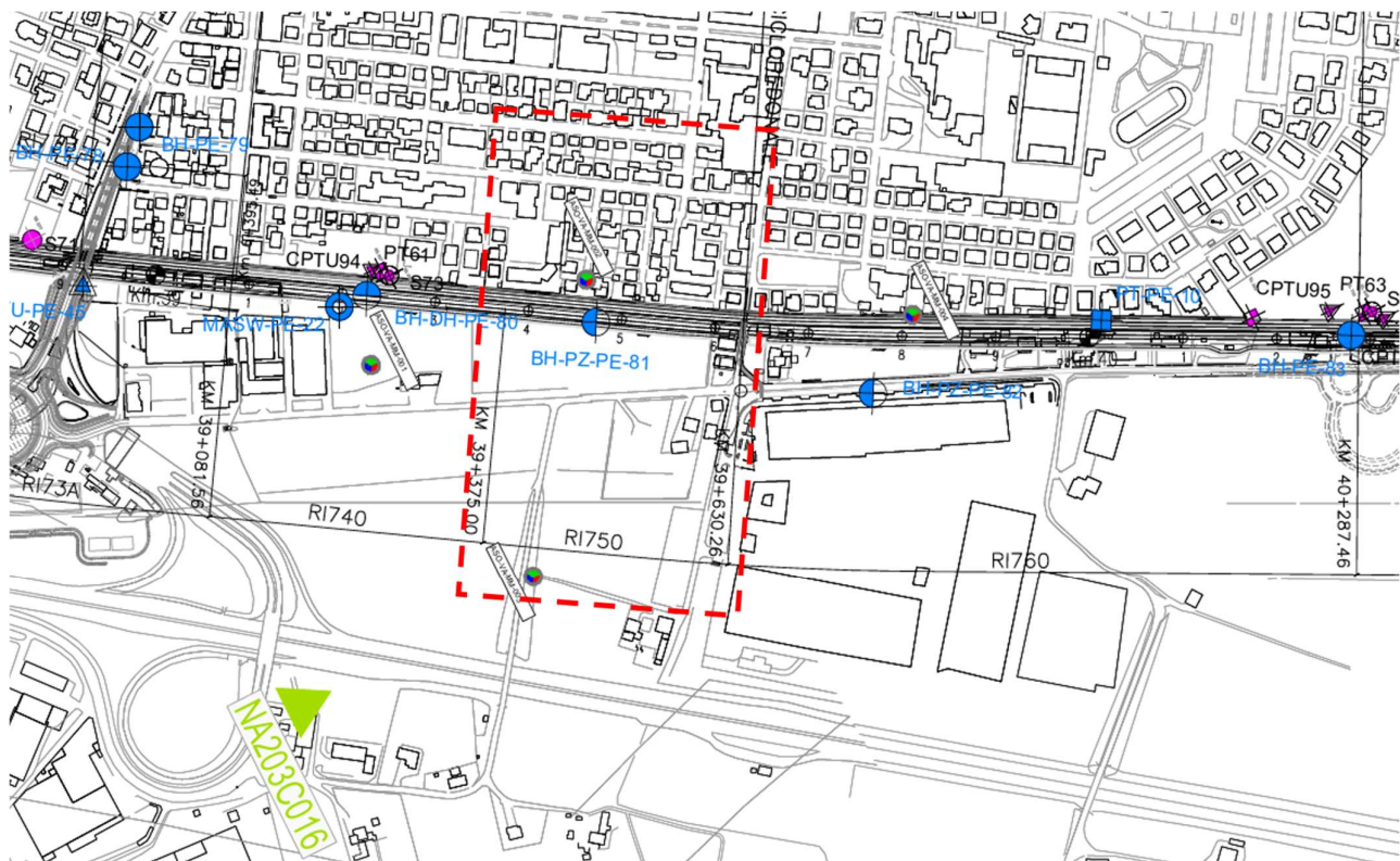
Figura 2 - Planimetria Rilevato RI75, estratto dalla Planimetria Generale (Doc. Rif. [3])
