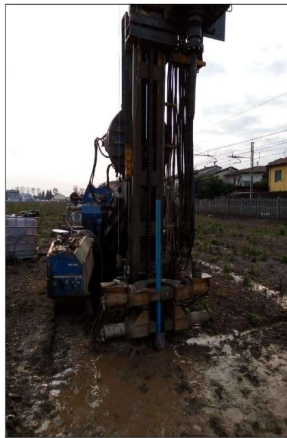
Tubo piezometrico
