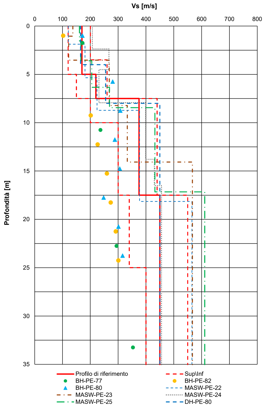
Figura 9 – Confronto Vs con dati di correlazioni da prove SPT e prove sismiche e Profilo generale tra pk 38+075 - pk 43+000 (Doc. Rif.[2])
