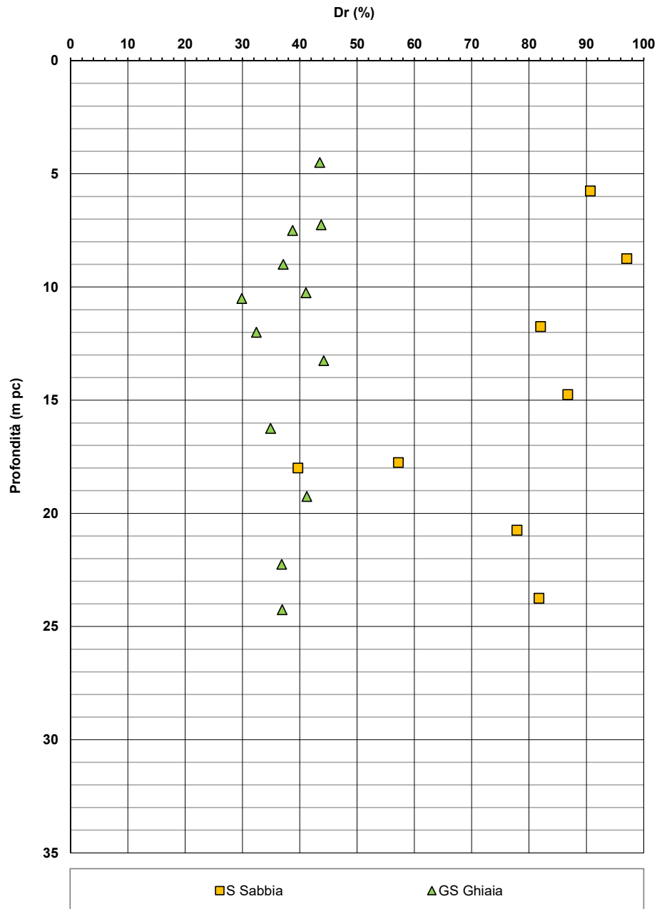
Figura 6 – Densità relativa da prove SPT – RI75
