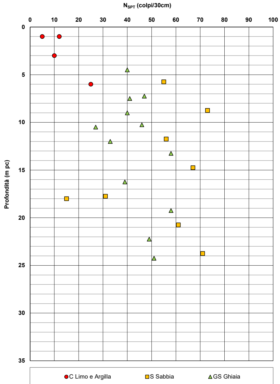
Figura 4 – Risultati delle prove SPT – RI75
