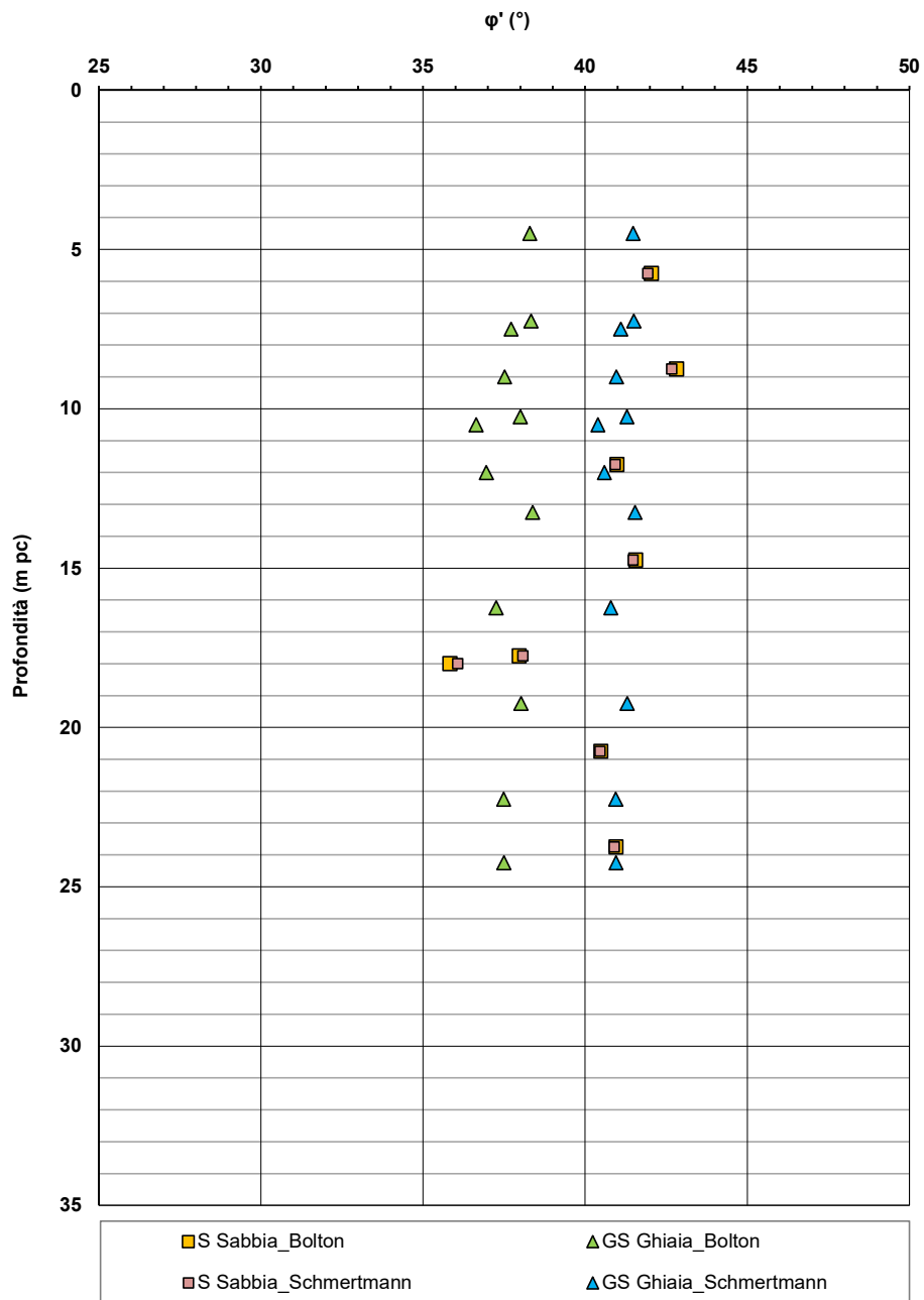
Figura 7 – Angoli di resistenza al taglio da prove SPT – RI75
