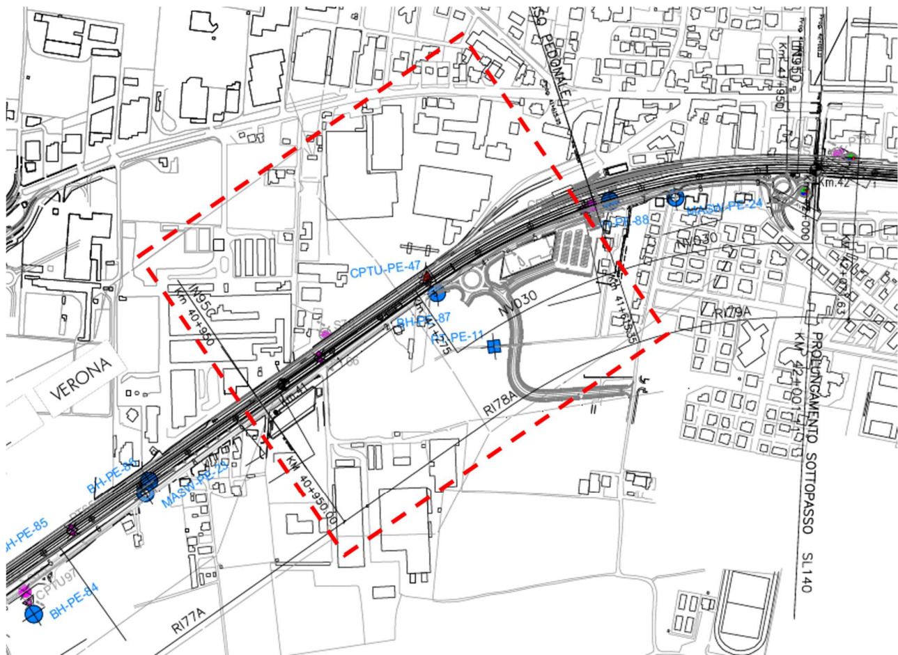
Figura 2 - Planimetria Rilevato RI78A, estratto dalla Planimetria Generale (Doc. Rif.[3])
