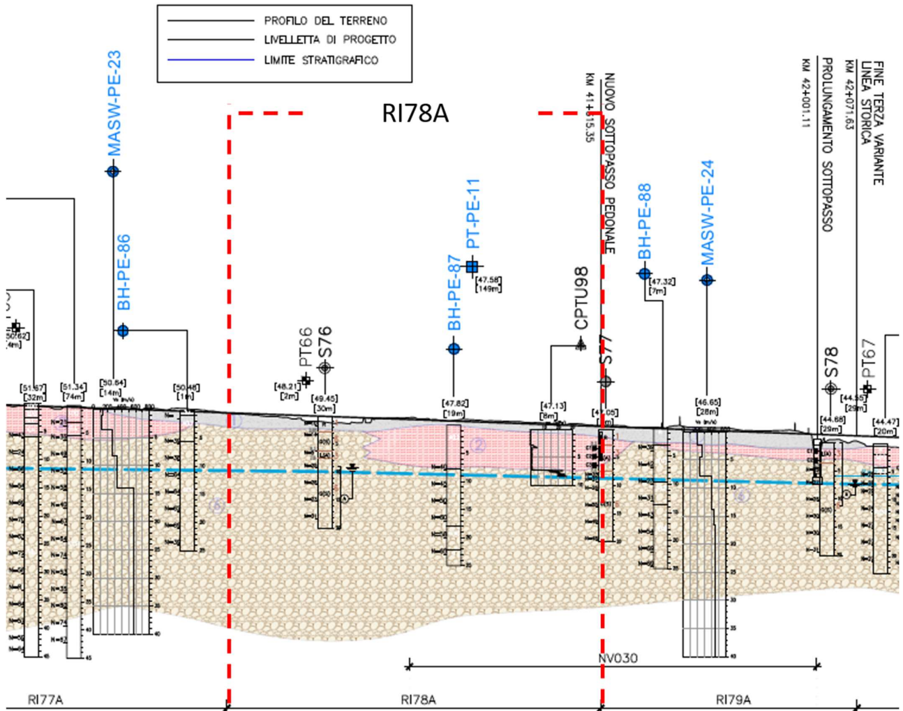
Figura 3 - Profilo Geotecnico Rilevato RI78A, estratto dal Profilo Geotecnico Generale
