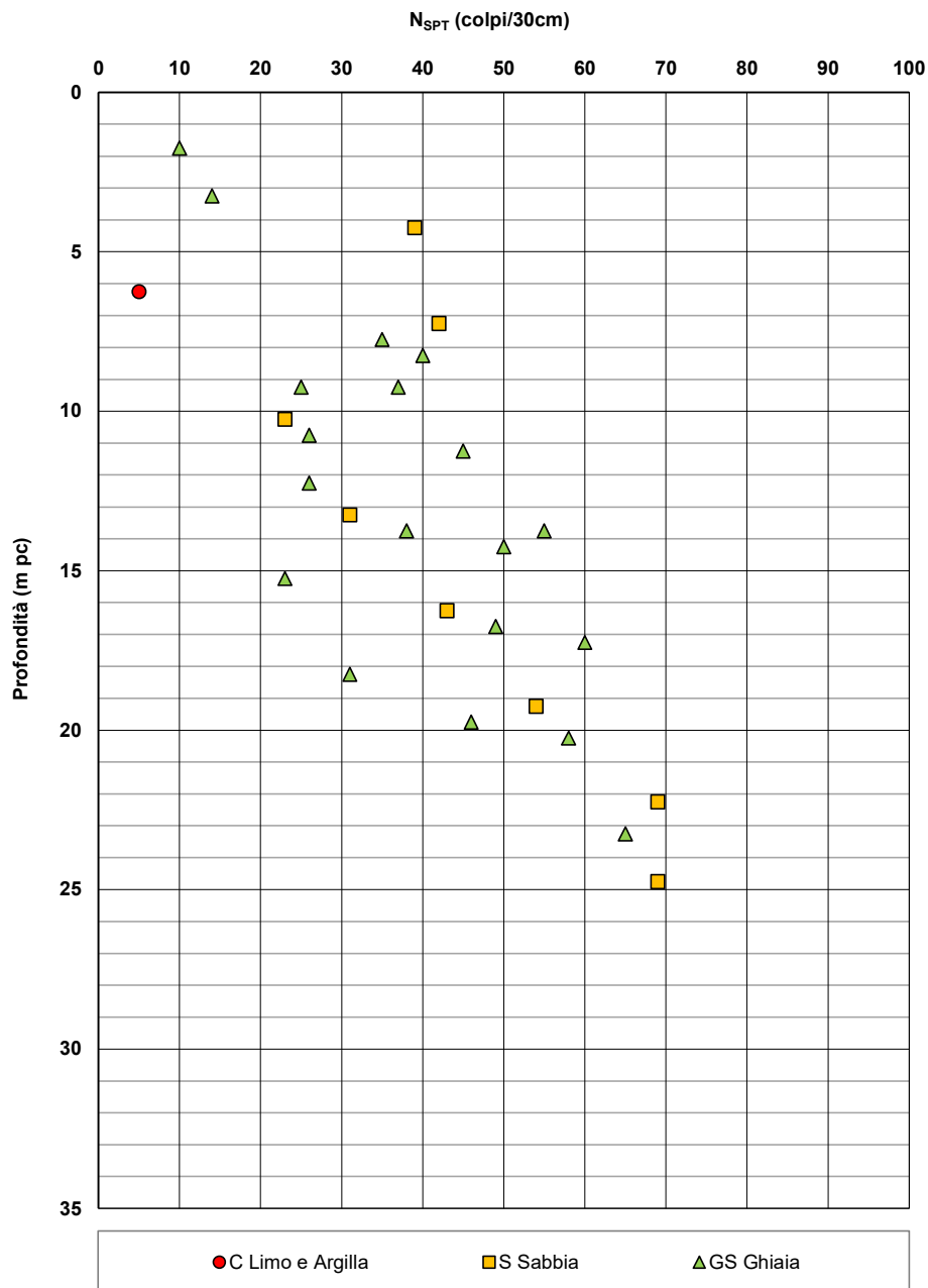
Figura 4 – Risultati delle prove SPT – RI78A
