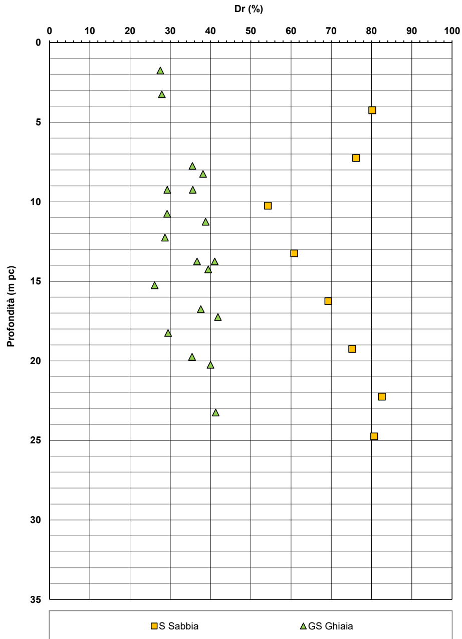
Figura 6 – Densità relativa da prove SPT – RI78A
