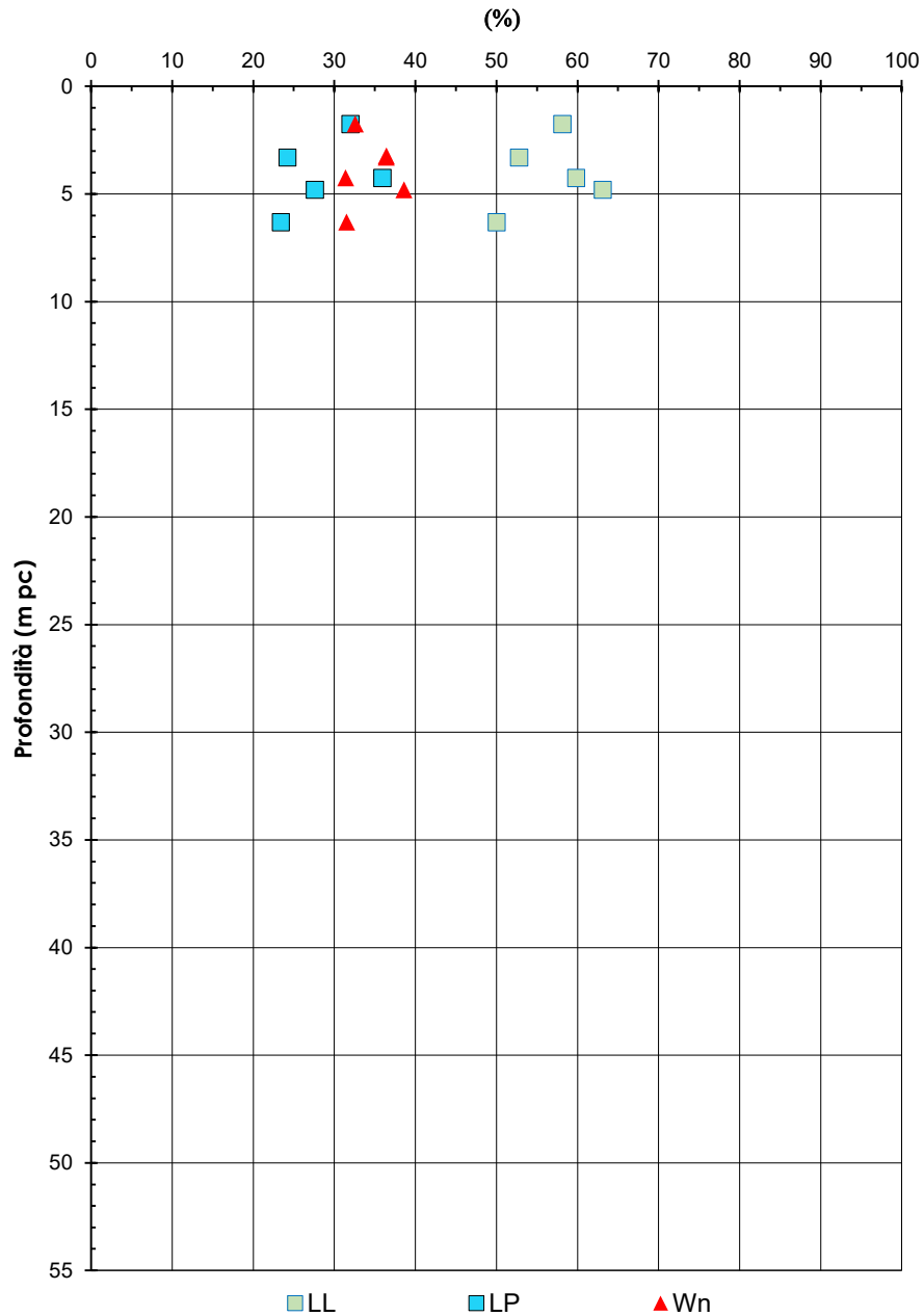
Figura 8 – Contenuto d'acqua, limite liquido e limite plastico – RI78A
