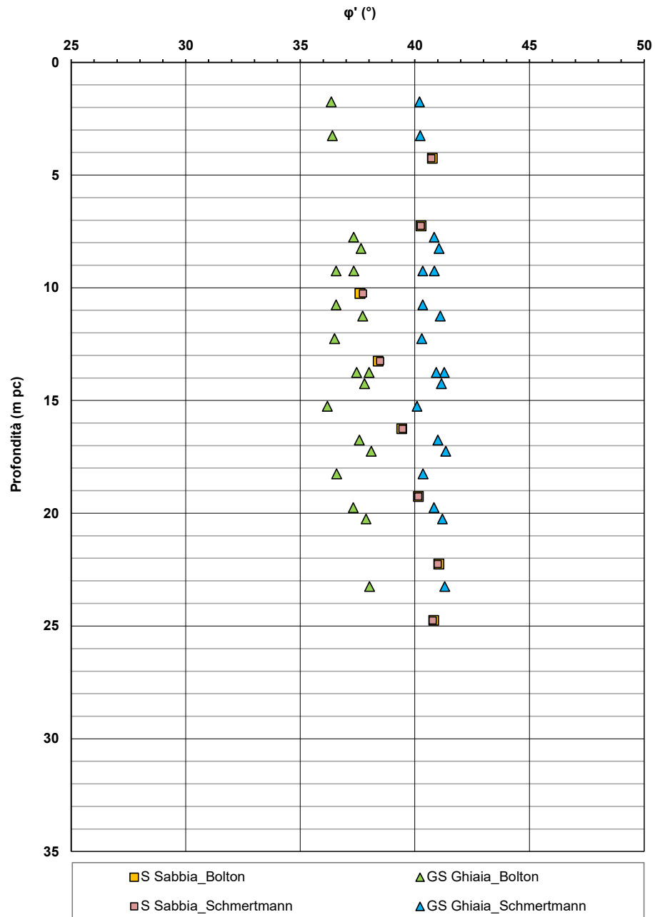
Figura 7 – Angoli di resistenza al taglio da prove SPT – RI78A
