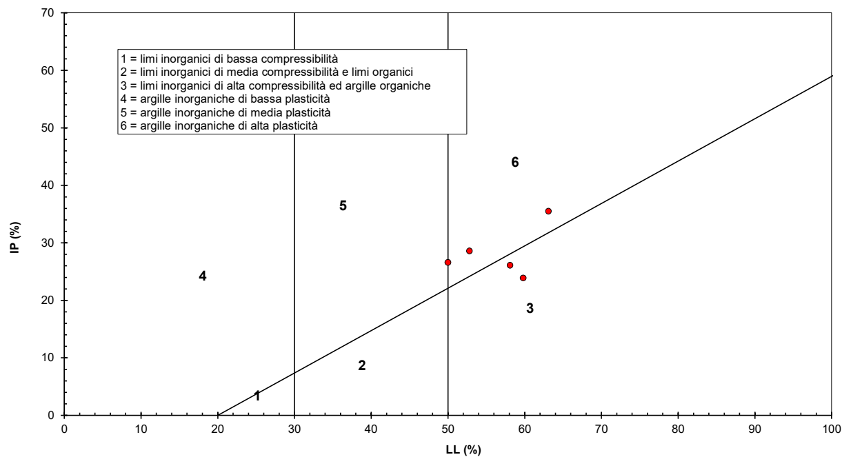
Figura 9 – Carta di Casagrande terreni Unità 2 – RI78A
