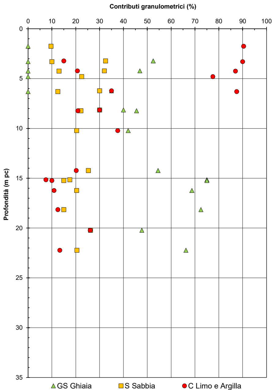
Figura 5 – Sintesi analisi granulometriche – RI78A
