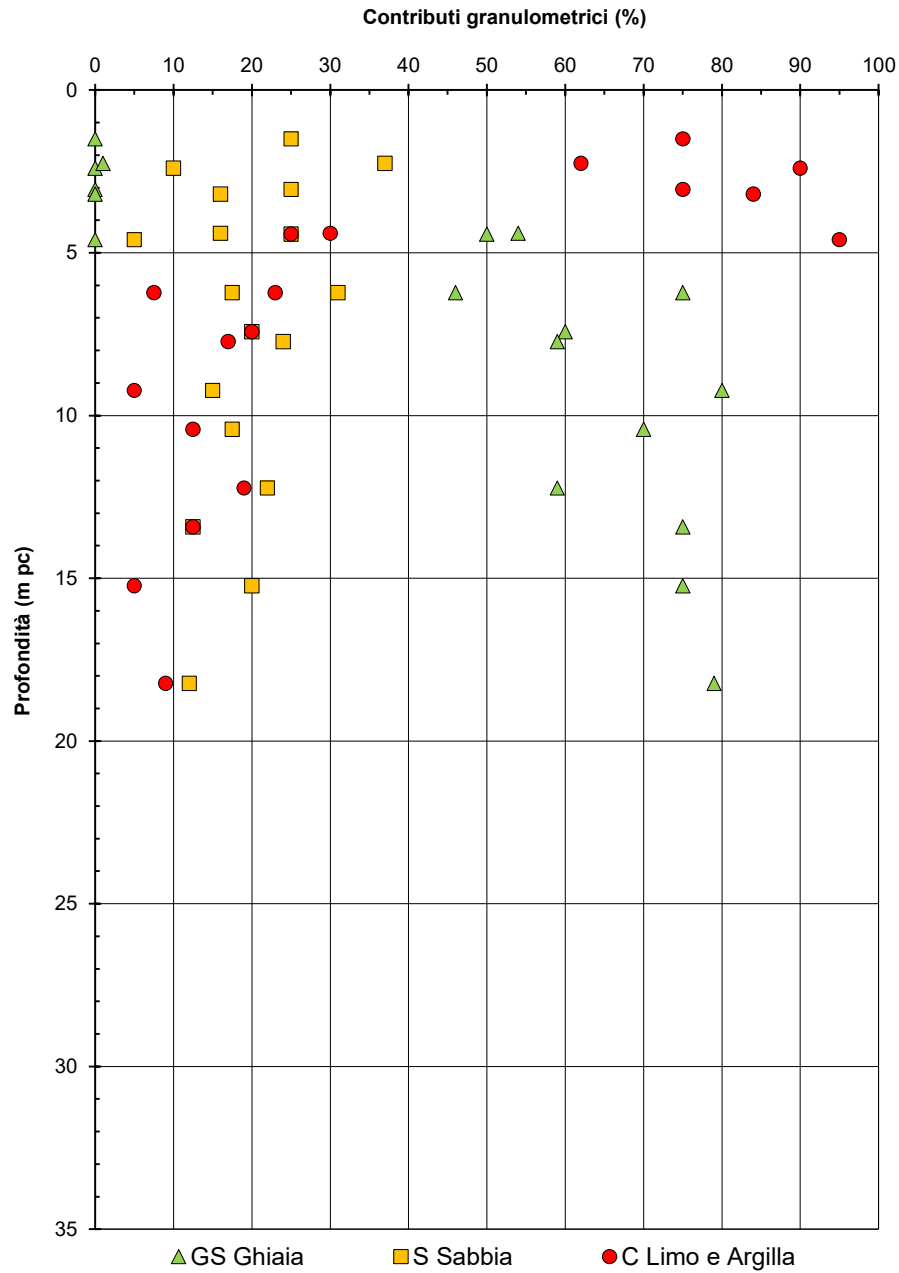
Figura 5 – Sintesi analisi granulometriche – RI800
