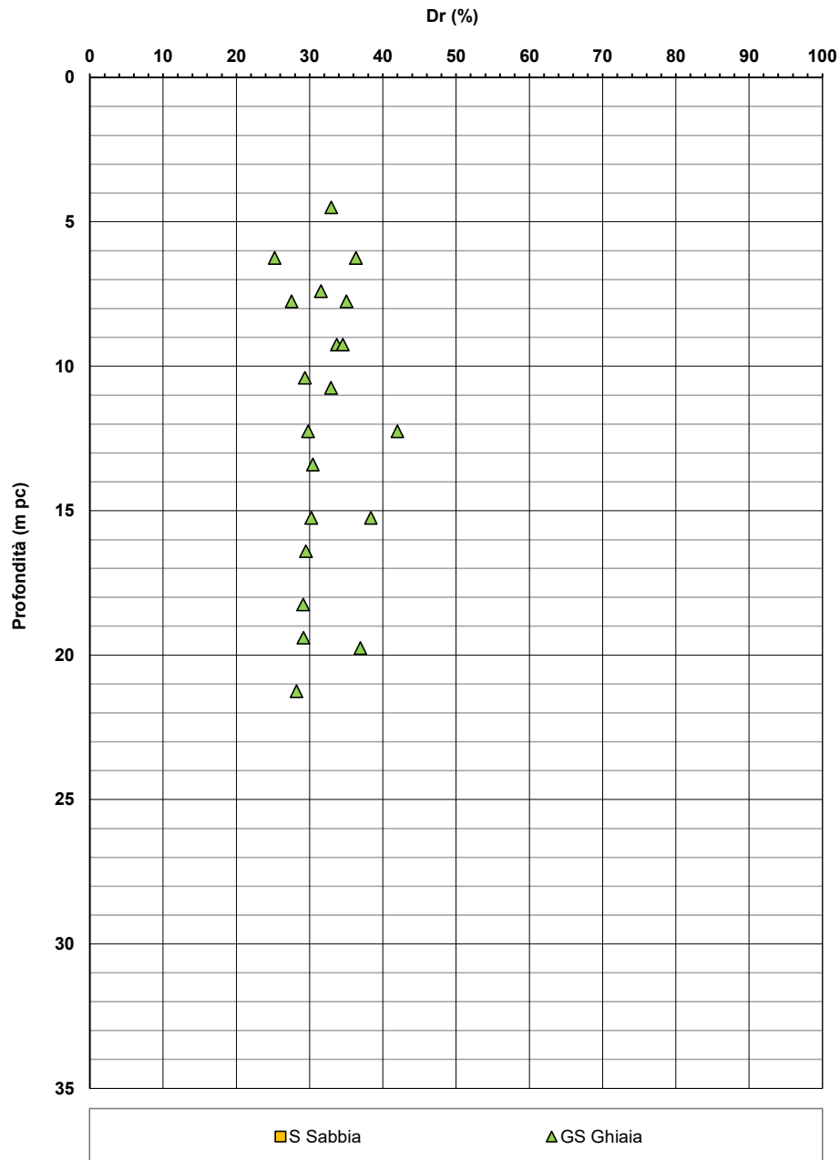
Figura 6 – Densità relativa da prove SPT – RI800
