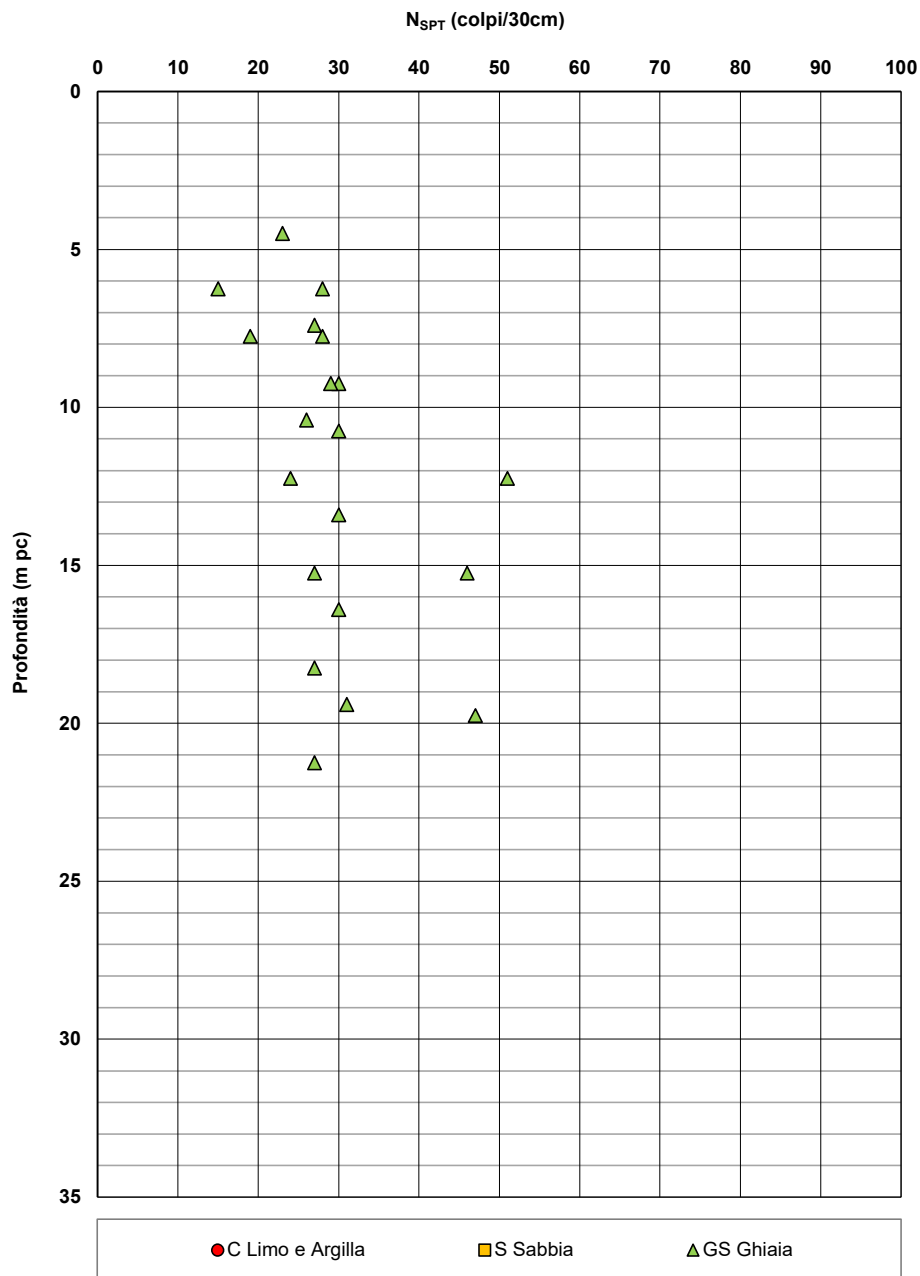
Figura 4 – Risultati delle prove SPT – RI800
