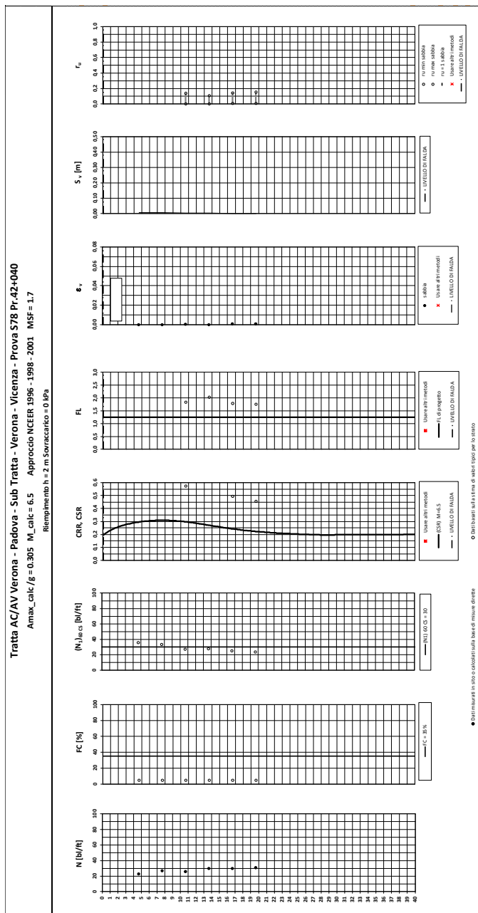
Figura 15 – Verifica Liquefazione da risultati S78
