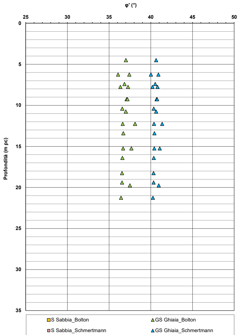
Figura 7 – Angoli di resistenza al taglio da prove SPT – RI800
