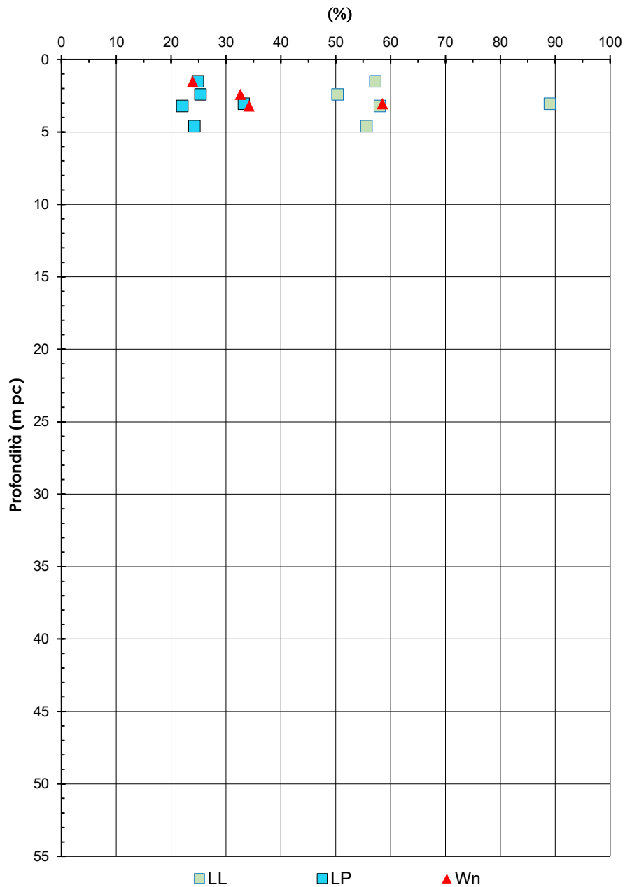
Figura 8 – Contenuto d'acqua, limite liquido e limite plastico – RI800
