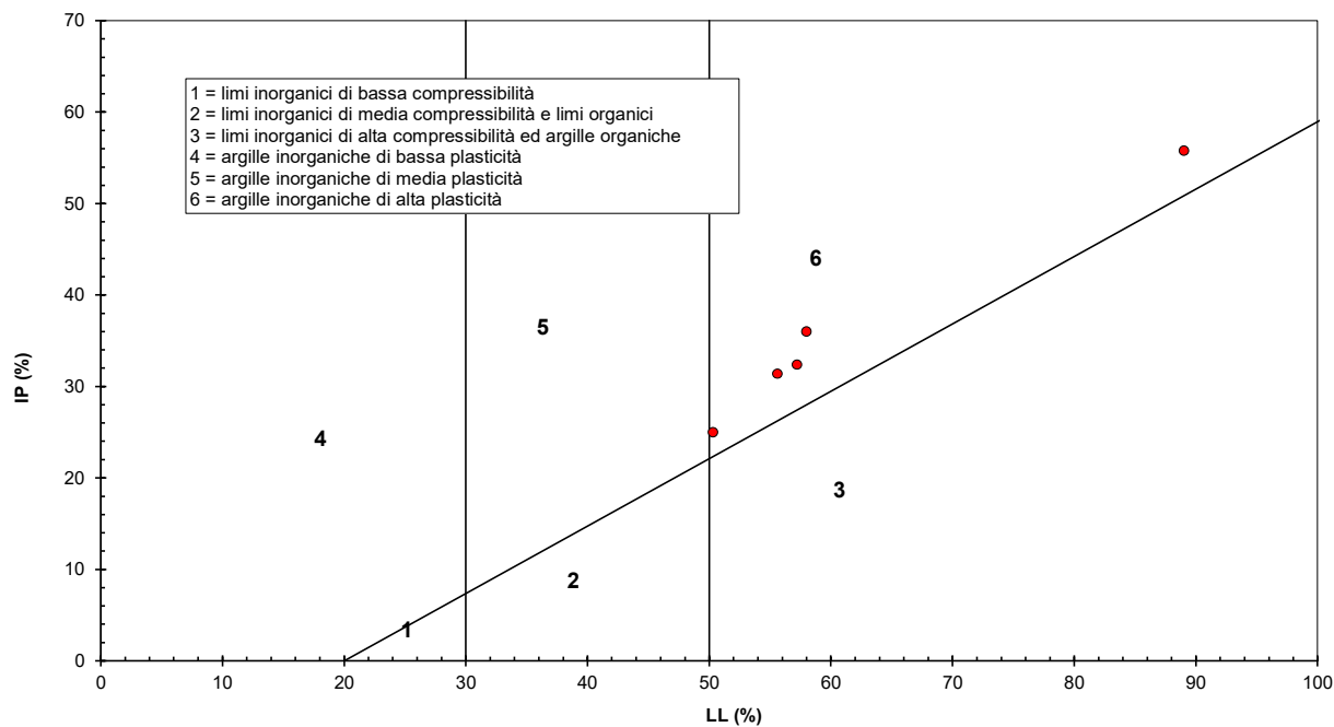
Figura 9 – Carta di Casagrande terreni Unità 2 – RI800
