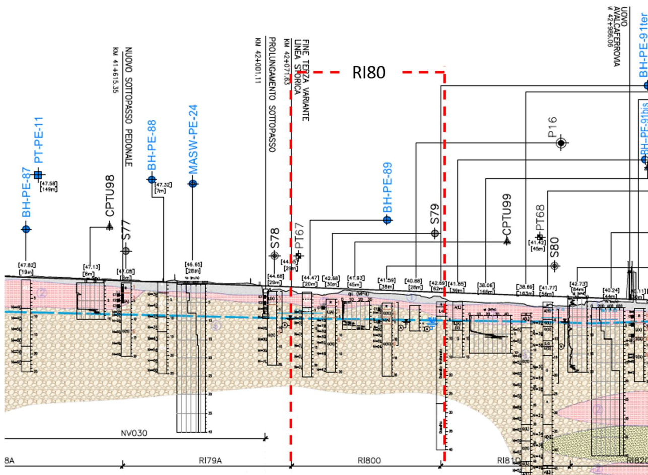
Figura 3 - Profilo Geotecnico Rilevato RI800, estratto dal Profilo Geotecnico Generale
