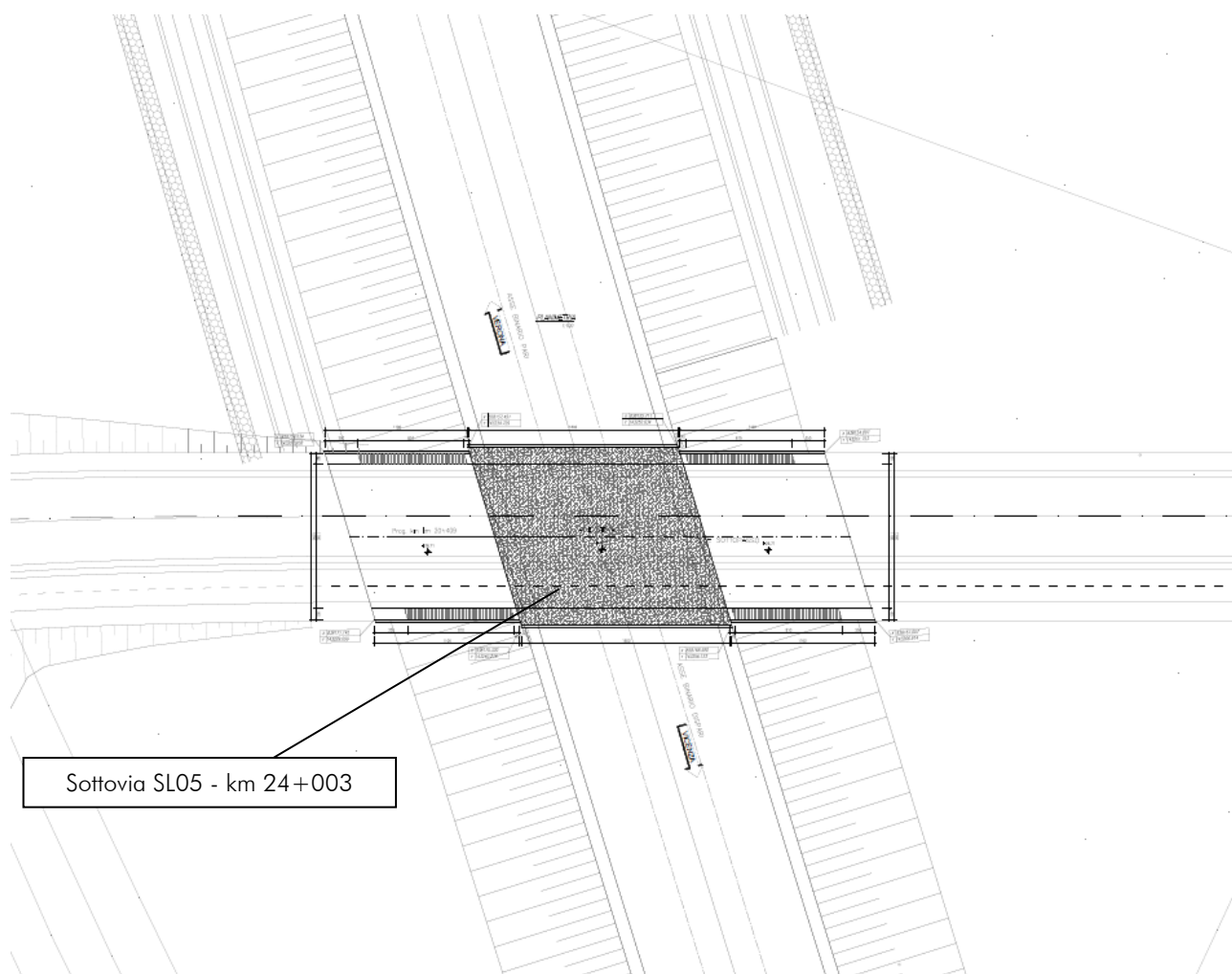
Figura 1: Stralcio planimetrico – Sottovia SL05
