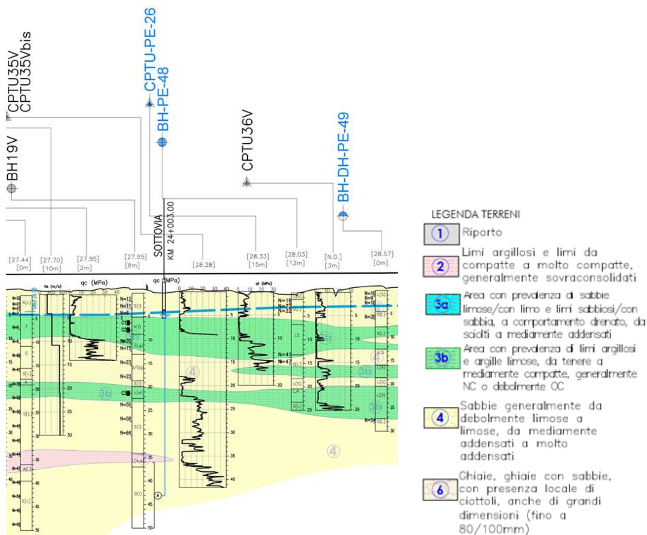
Figura 10: Profilo geotecnico di linea in corrispondenza della progressiva dell'opera in esame
