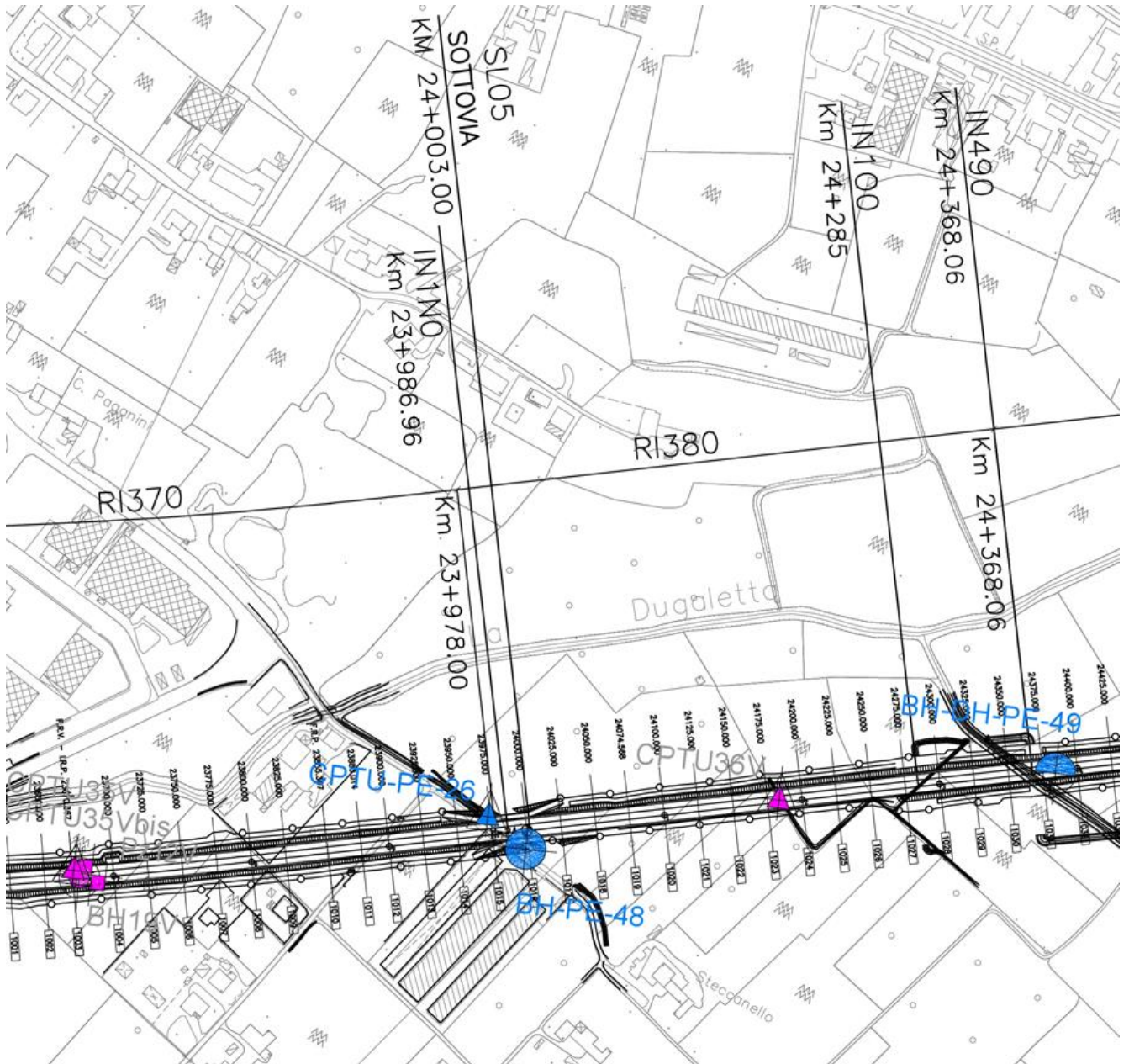
Figura 2: Stralcio planimetrico – Ubicazione indagini geotecniche di riferimento per l'opera in esame
