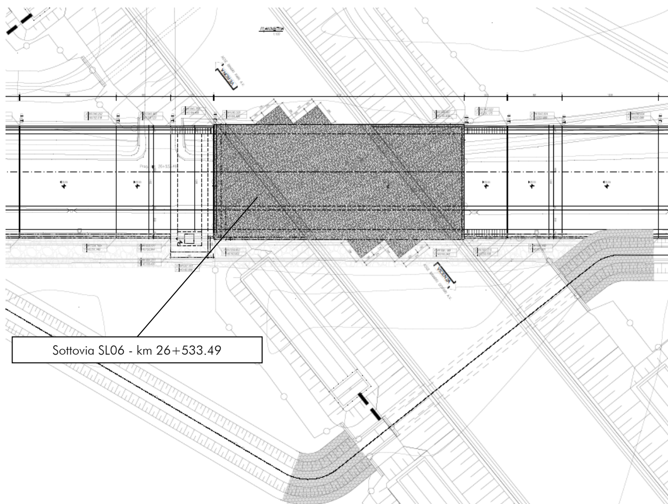
Figura 1: Stralcio planimetrico – Sottovia SL06
