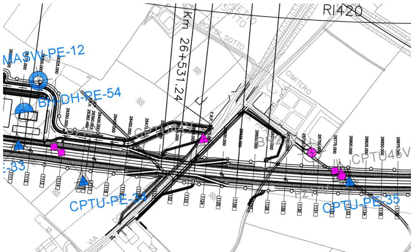
Figura 2: Stralcio planimetrico – Ubicazione indagini geotecniche di riferimento per l'opera in esame
