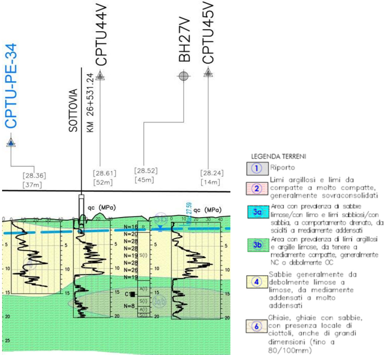
Figura 10: Profilo geotecnico di linea in corrispondenza della progressiva dell'opera in esame
