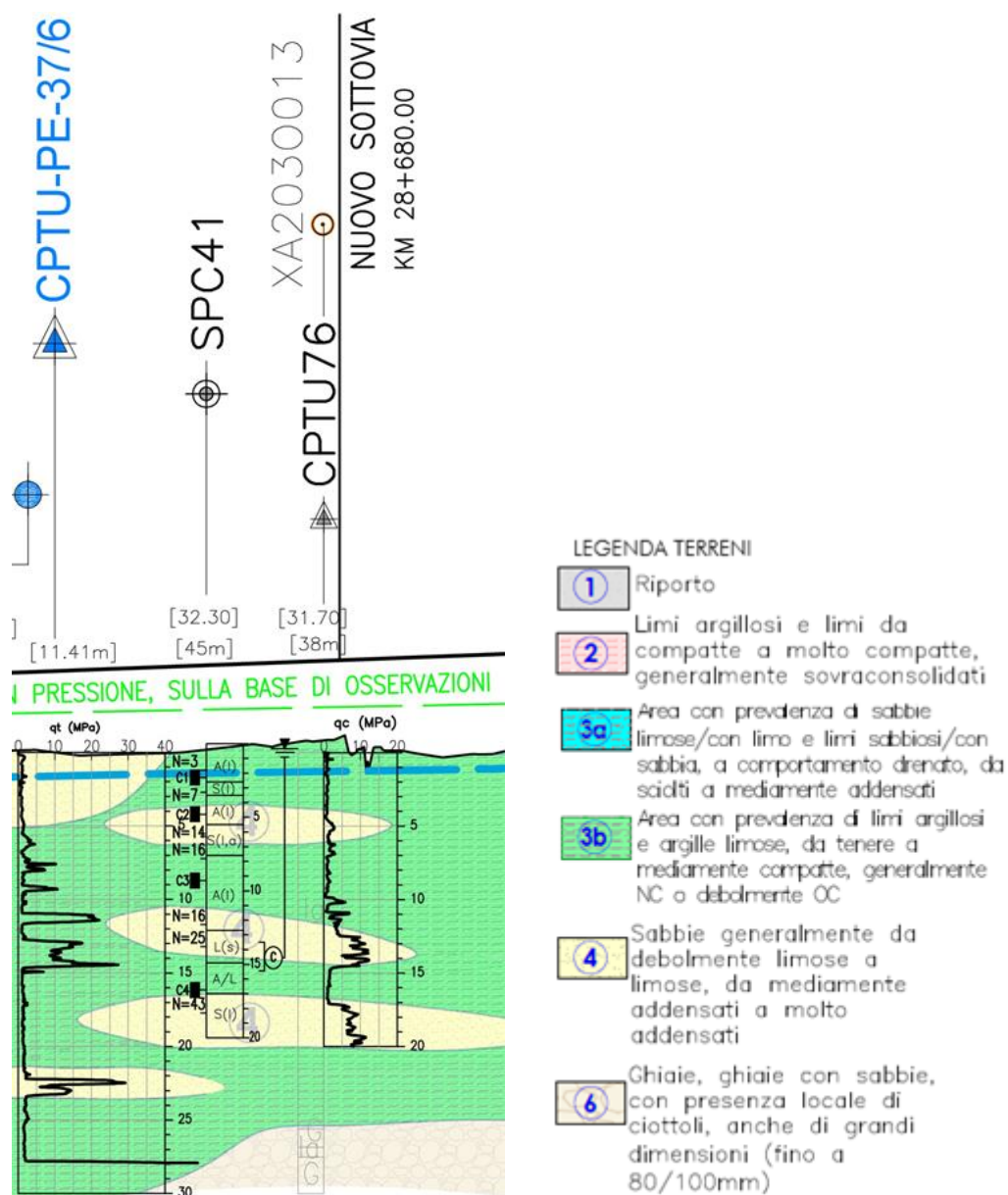
Figura 10: Profilo geotecnico di linea in corrispondenza della progressiva dell'opera in esame
