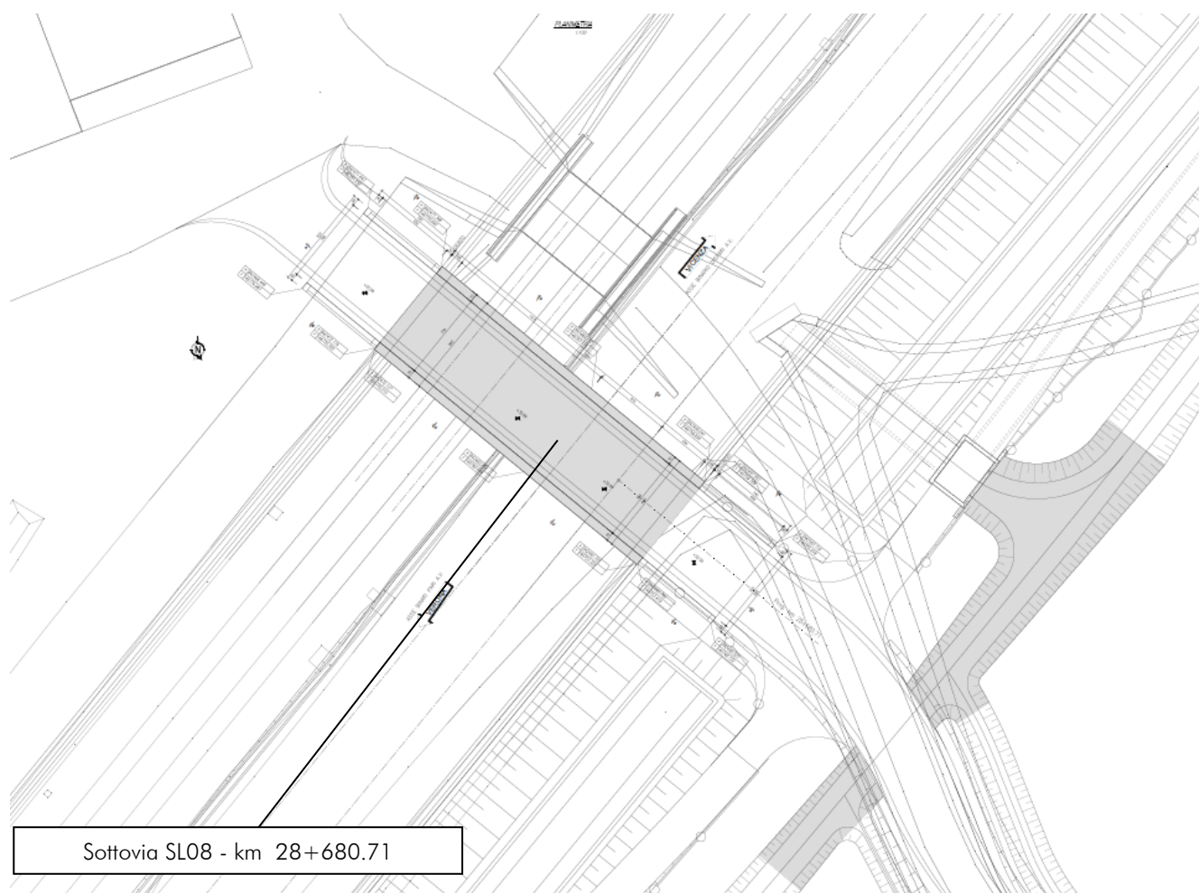
Figura 1: Stralcio planimetrico – Sottovia SL08
