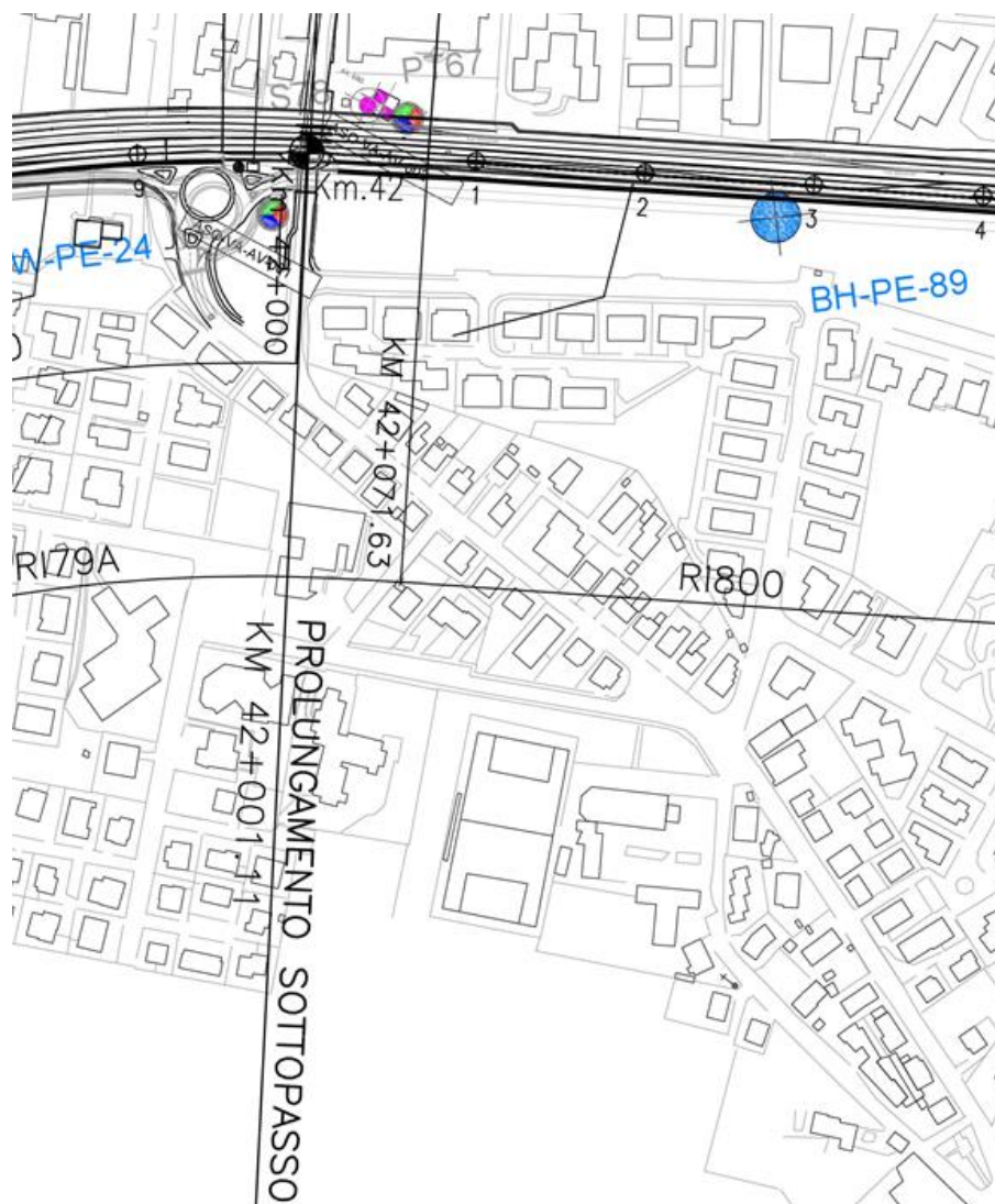
Figura 2: Stralcio planimetrico – Ubicazione indagini geotecniche di riferimento per l'opera in esame
