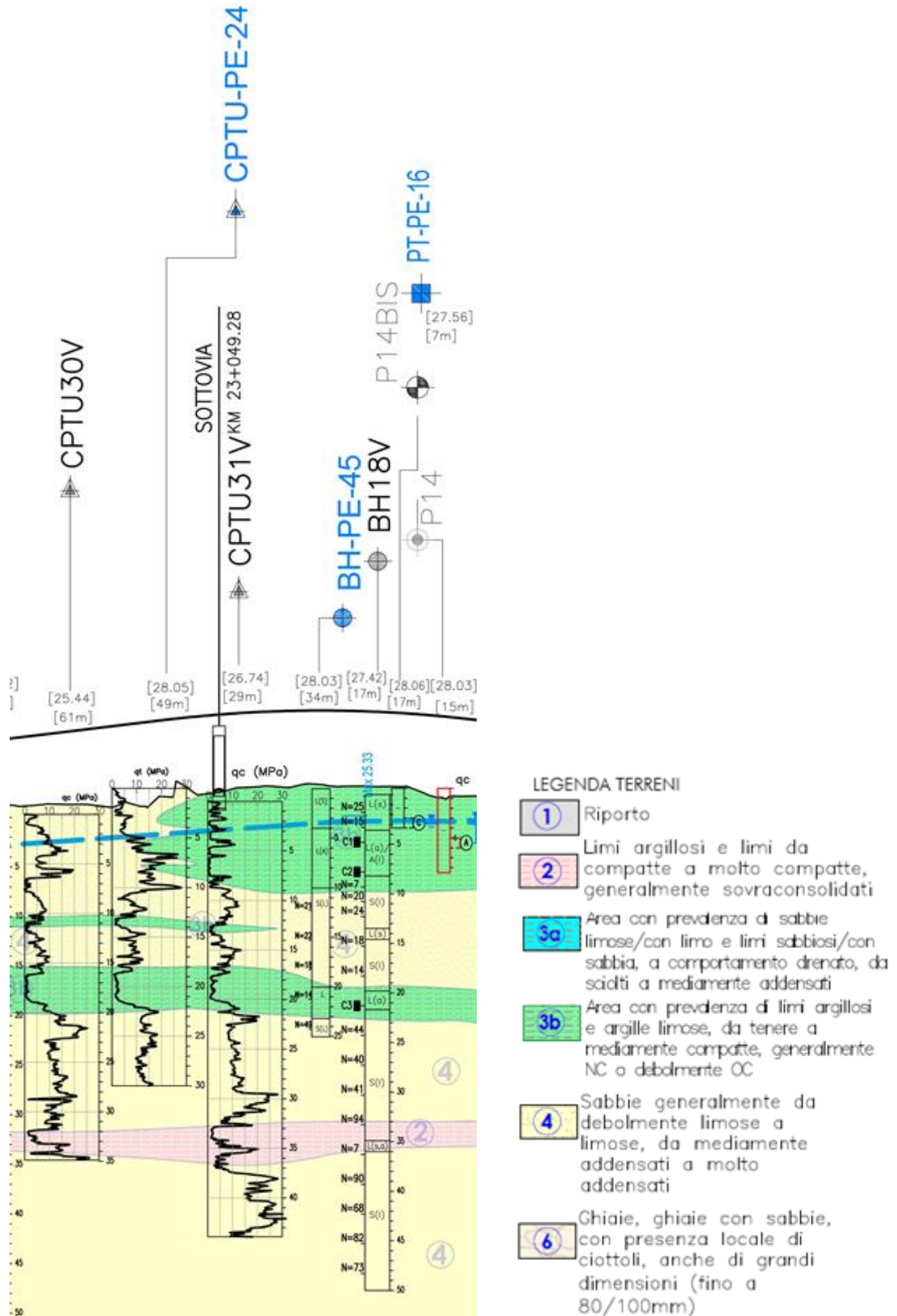
Figura 10: Profilo geotecnico di linea in corrispondenza della progressiva dell'opera in esame
