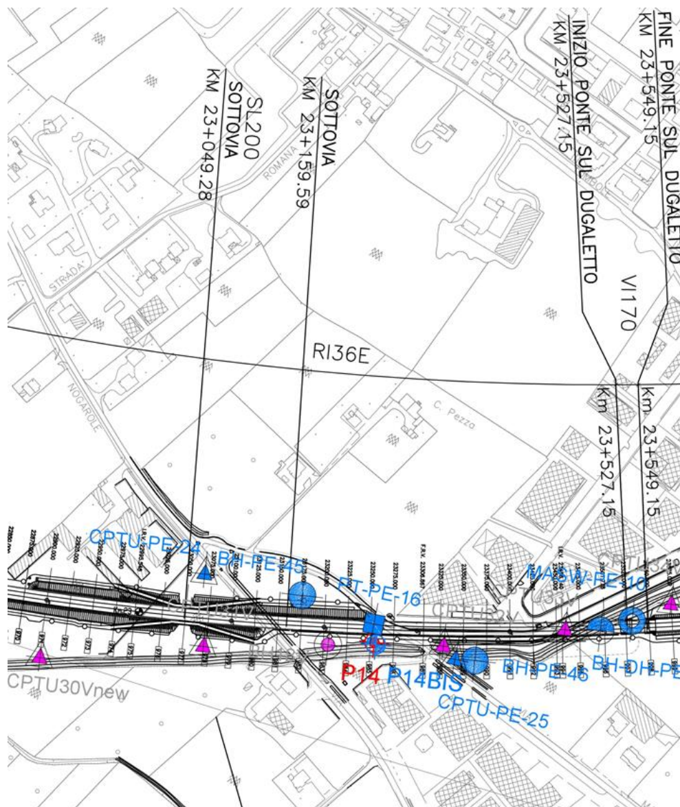
Figura 2: Stralcio planimetrico – Ubicazione indagini geotecniche di riferimento per l'opera in esame
