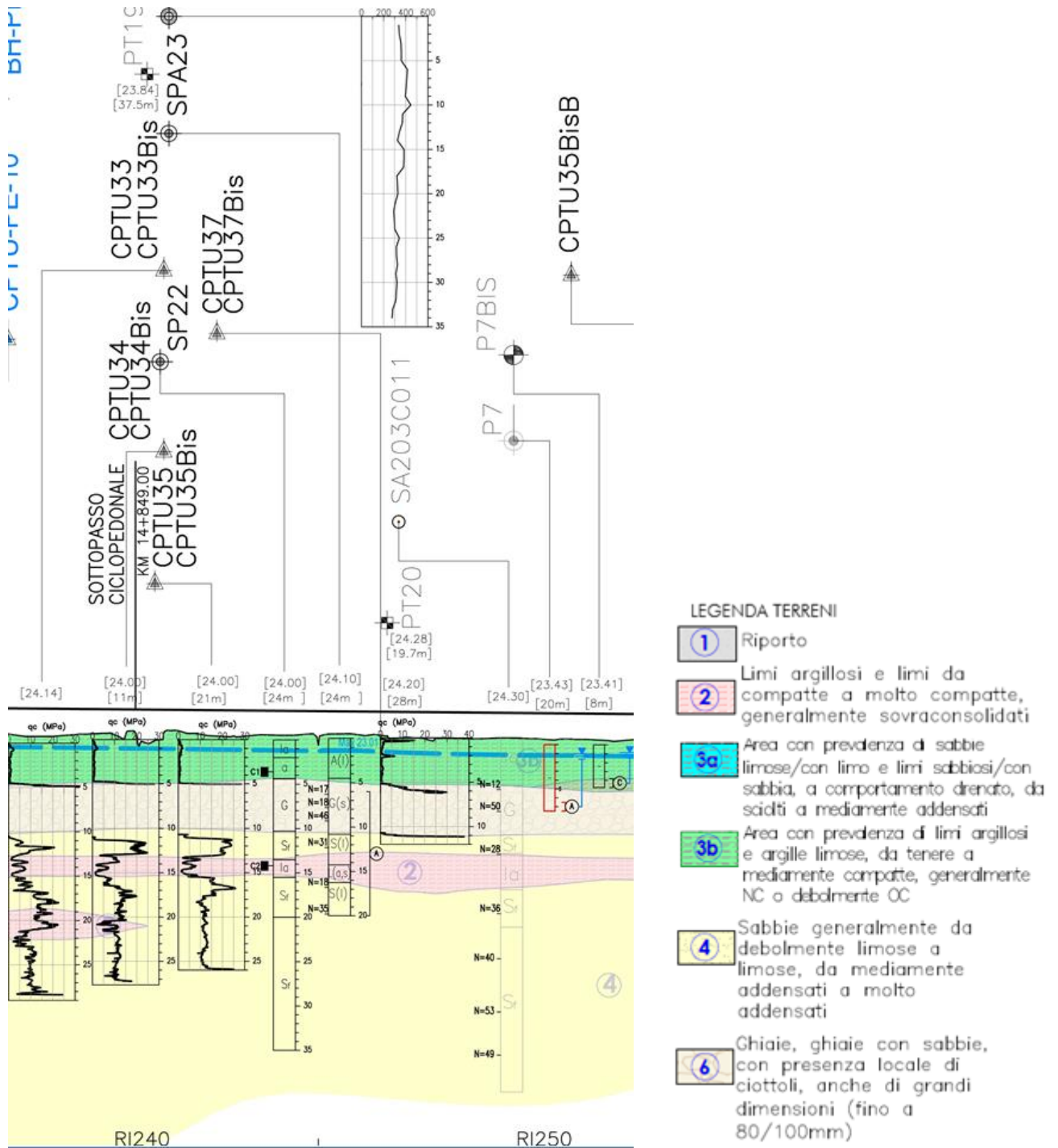
Figura 10: Profilo geotecnico di linea in corrispondenza della progressiva dell'opera in esame
