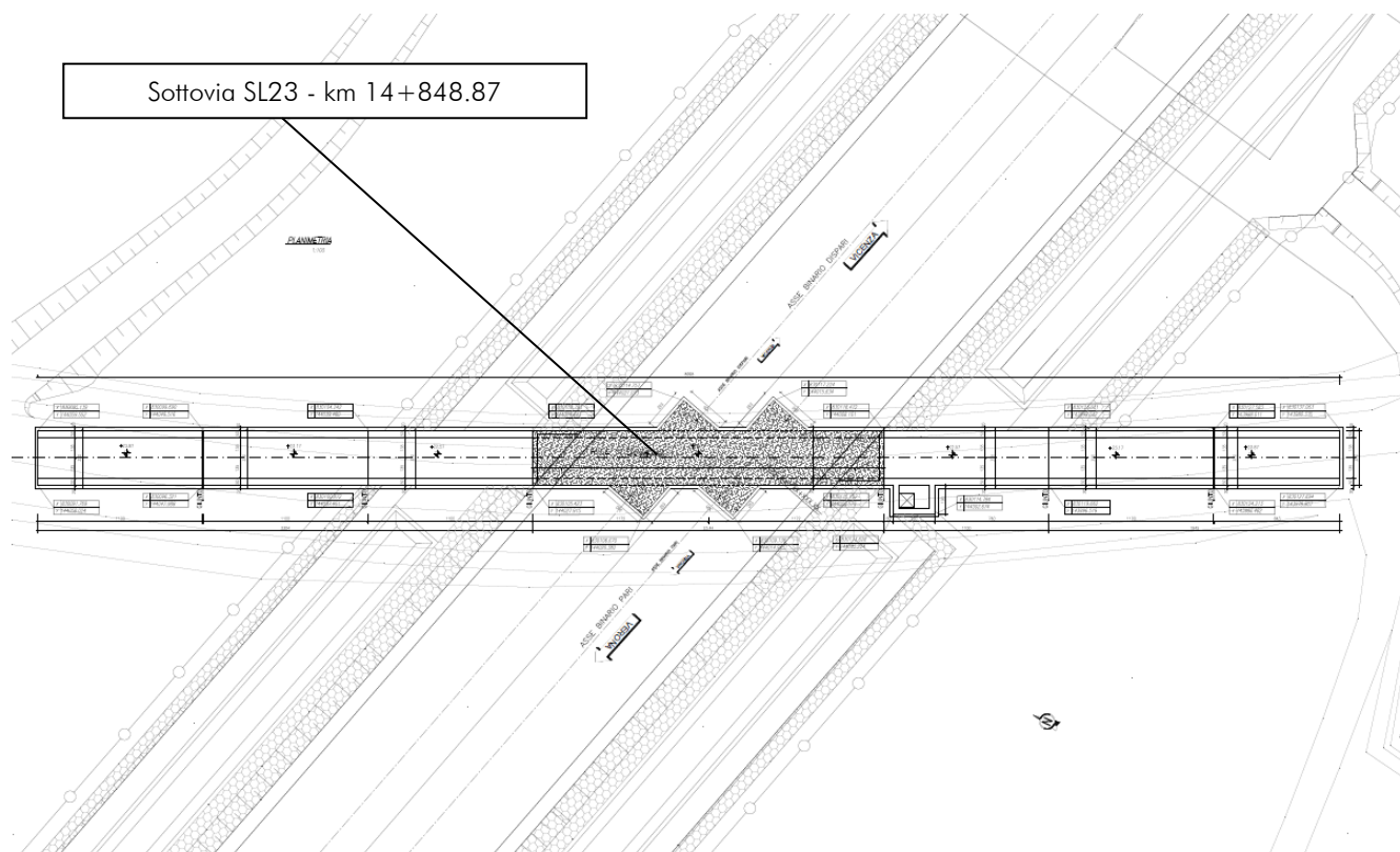
Figura 1: Stralcio planimetrico – Sottovia SL23
