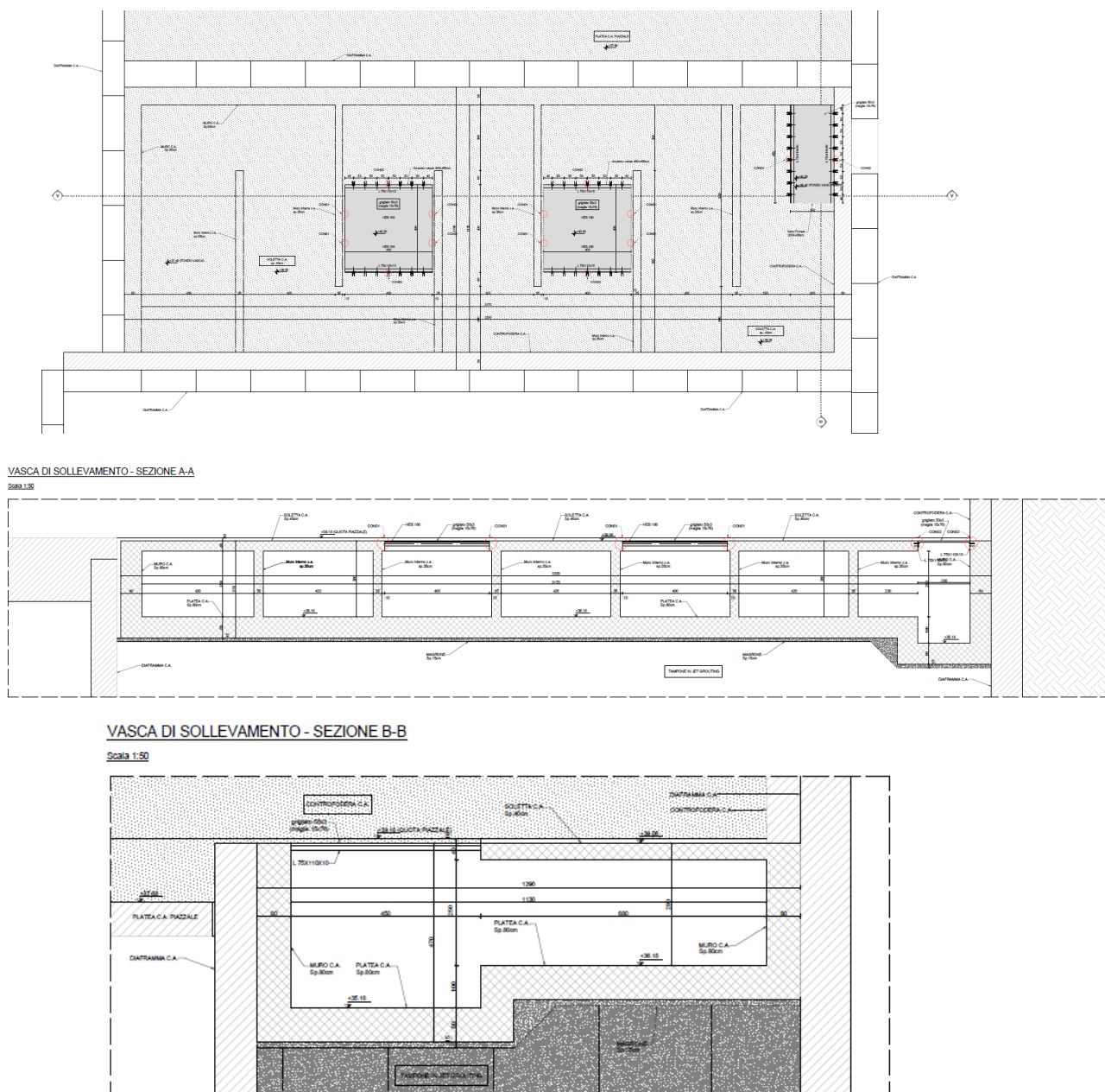
Figura 1 Pianta e sezione della vasca in c.a.
