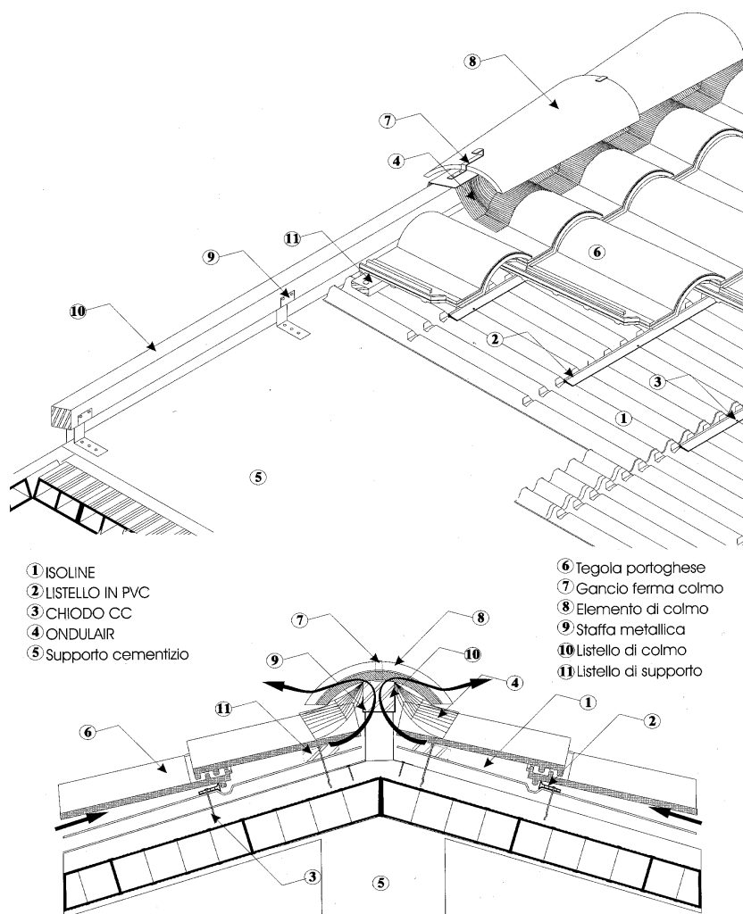
Figura 7 - Particolare tipologico di ancoraggio delle lastre sottotegola –linea di colmo
