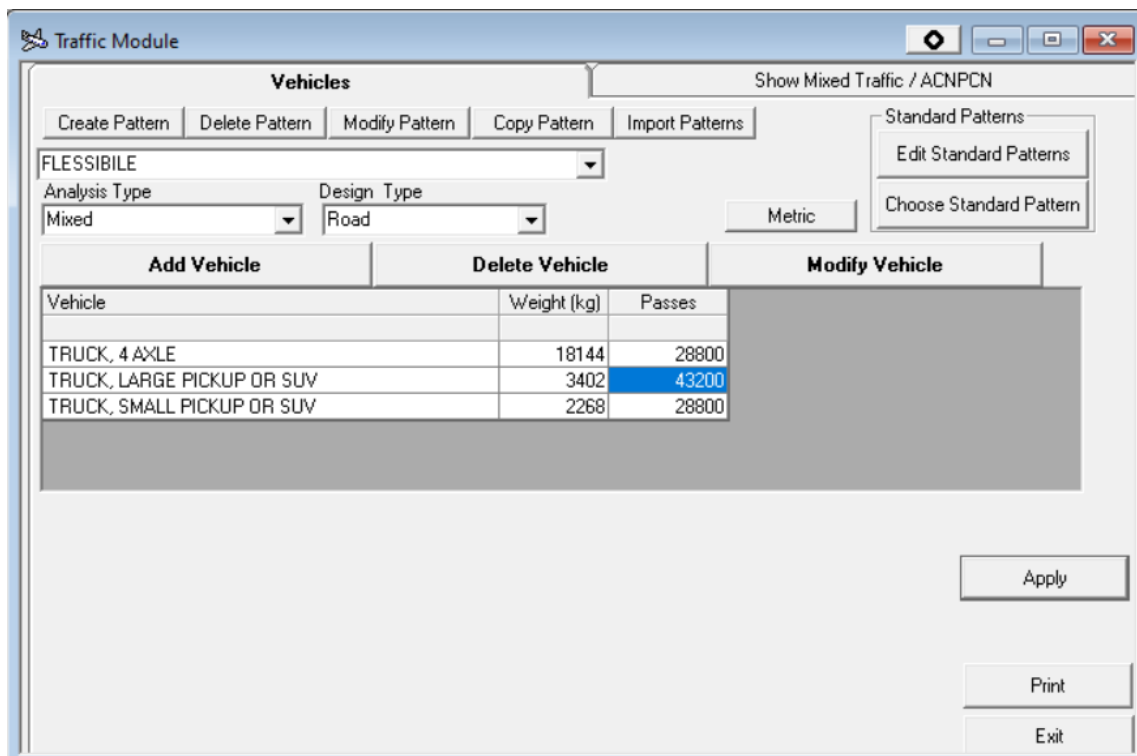
Figura 11 – Spettro di traffico pavimentazione flessibile
