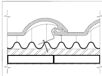
Figura 9 - Particolare tipologico del fissaggio della lastra sottotegola
