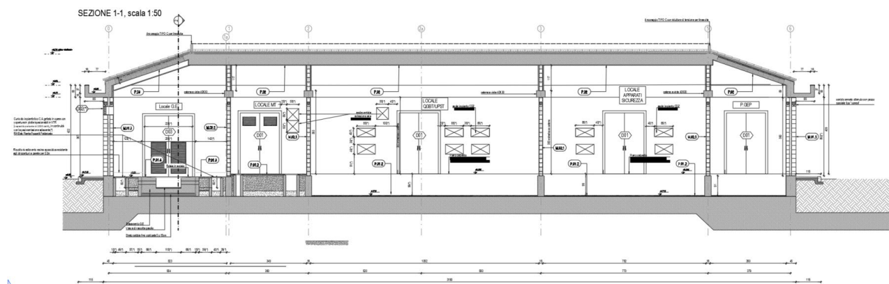
Figura 3 Sezione edificio
