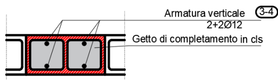
Tipologico pilastro Muratura perimetrale doppia camera
