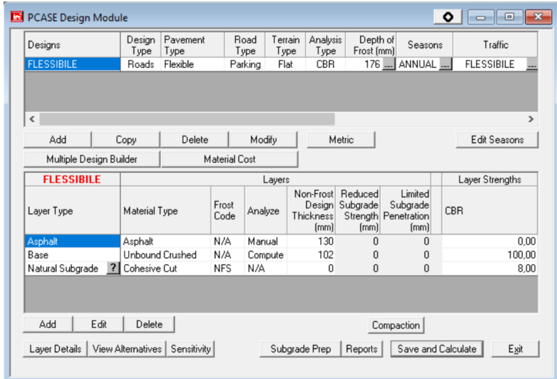
Figura 14 - Spessori minimi pavimentazione flessibile carrabile
