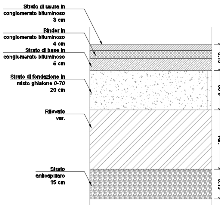
Figura 16 - Pavimentazione carrabile
