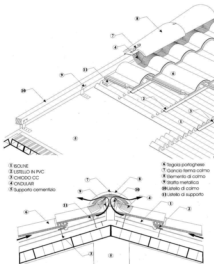
Figura 4 - Particolare tipologico di ancoraggio delle lastre sottotegola –linea di colmo
