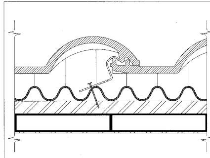
Figura 6 - Particolare del fissaggio della prima fila di tegole
