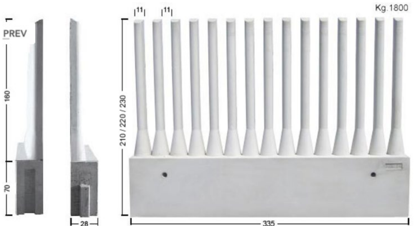
Figura 17 - Recinzione a pettine (esempio)
