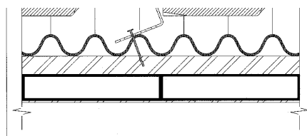
Figura 3 - Particolare del fissaggio della prima fila di tegole
