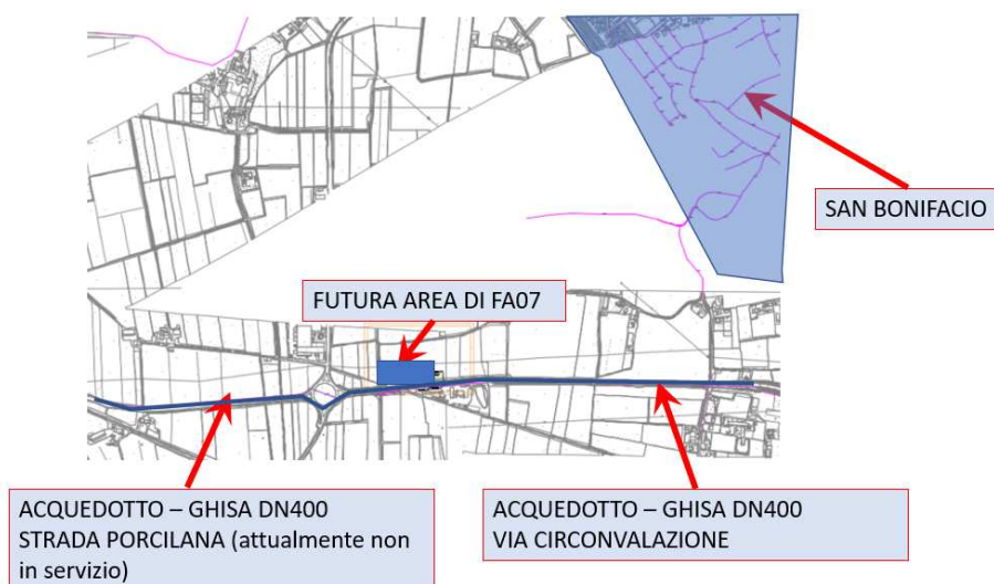
Figura 7-1: Attuale situazione dell'acquedotto presso FA07.
