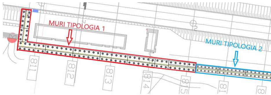
Figura 5 - Stralcio planimetrico: ubicazione muri in c.a.
