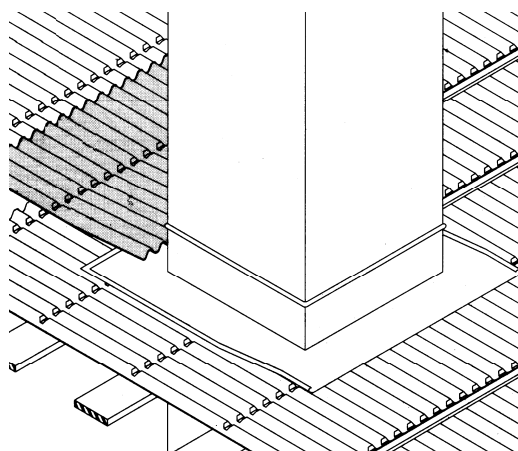
Figura 4 - Raccordo a camino
