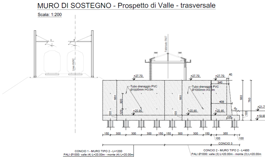
Figura 8 - Prospetto Trasversale muri di sostegno
