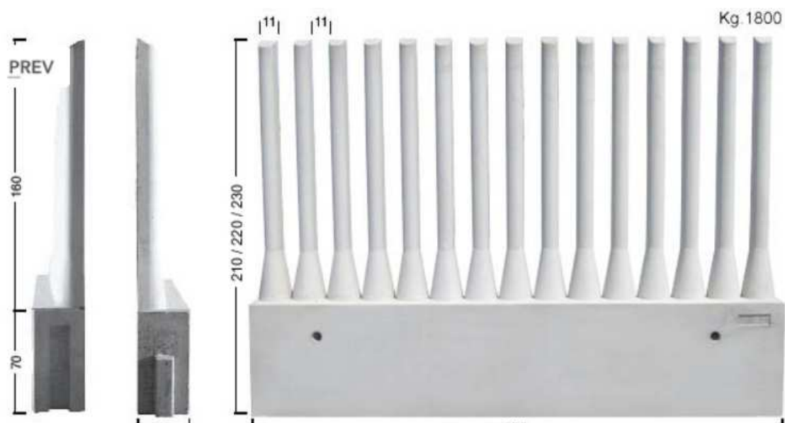
Figura 20 - Recinzione a pettine (esempio)
