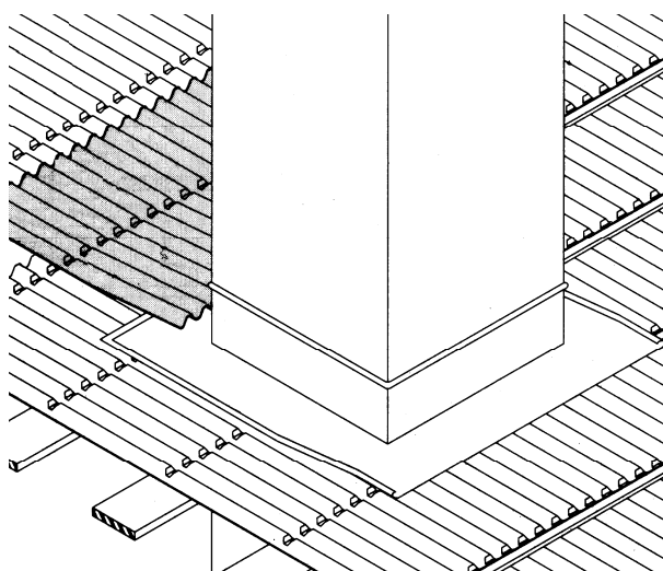
Figura 12 - Raccordo a camino
