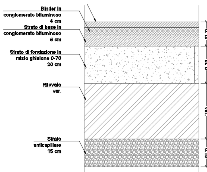
Figura 19 - Pavimentazione carrabile
