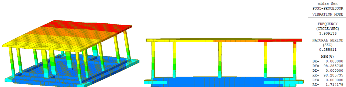
Figura 16 Cabina Terna 2° Modo di vibrare, periodo 0.2558 s, frequenza 3.9091 Hz
