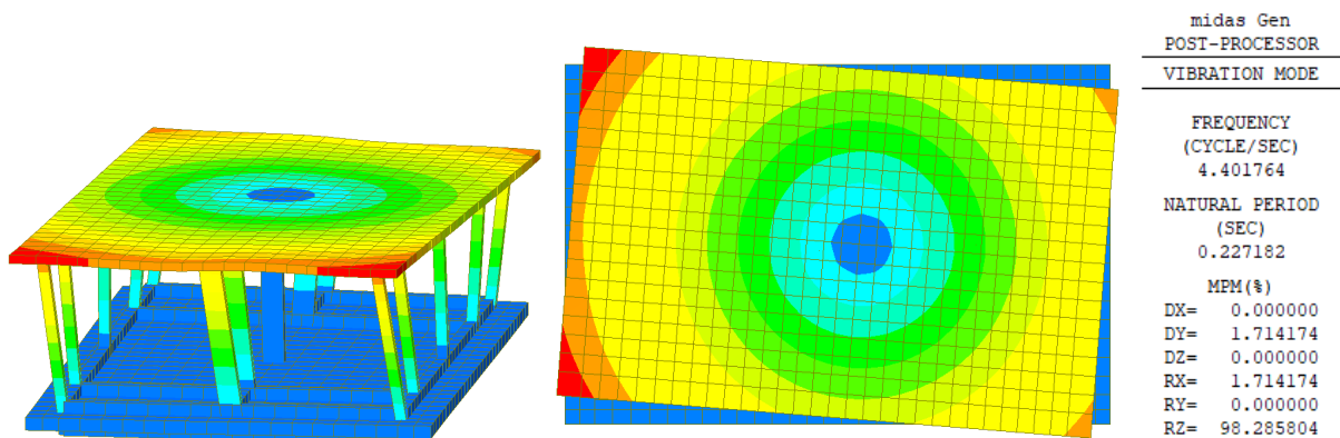
Figura 17 Cabina Terna 3° Modo di vibrare, periodo 0.2272 s, frequenza 4.4018 Hz
