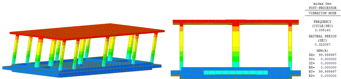
Figura 15 Cabina Terna 1° Modo di vibrare, periodo 0.323 s, frequenza 3.0951Hz
