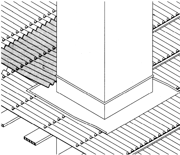
Figura 18 - Raccordo a camino
