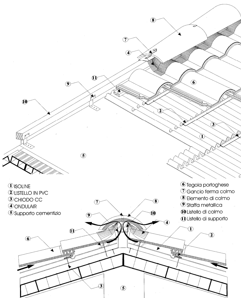
Figura 15 - Particolare tipologico di ancoraggio delle lastre sottotegola –linea di colmo
