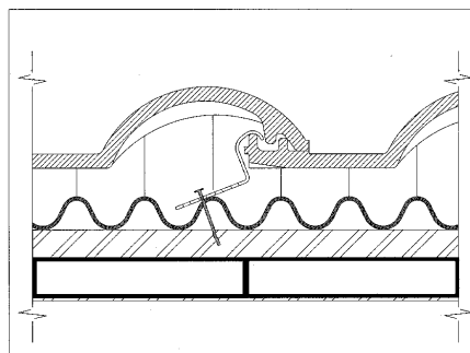
Figura 13 - Particolare del fissaggio della prima fila di tegole
