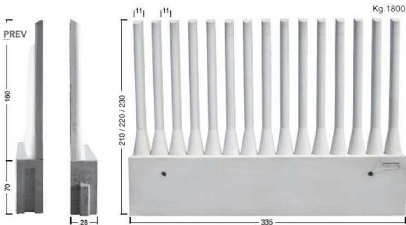
Figura 9 - Recinzione a pettine (esempio)
