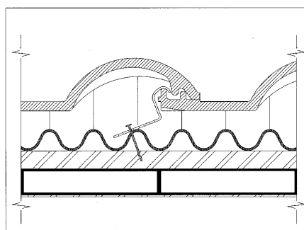
Figura 17 - Particolare tipologico del fissaggio della lastra sottotegola
