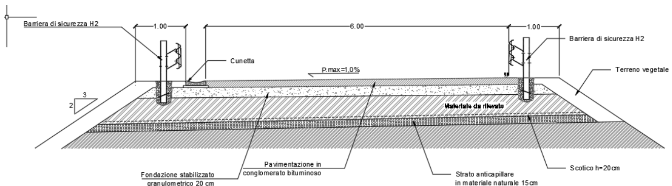
Figura 10 - Sezione tipo strada di accesso
