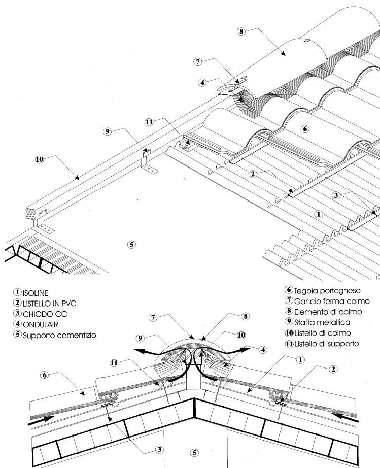
Figura 11 - Particolare tipologico di ancoraggio delle lastre sottotegola –linea di colmo
