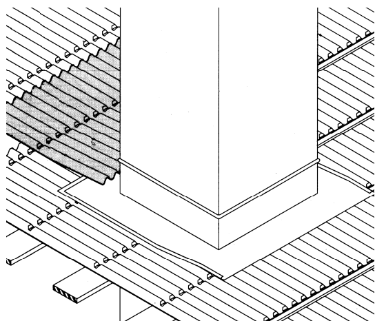
Figura 14 - Raccordo a camino
