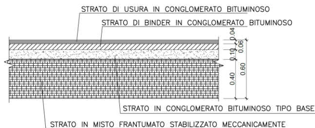
Figura 5: pavimentazione di progetto - strada Porcilana (tipo C1)
