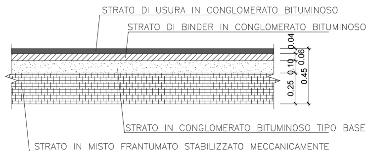
Figura 4: pavimentazione di progetto - strada Comunale (tipo F2) e Rampe
