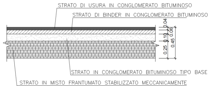
Figura 4: pavimentazione di progetto
