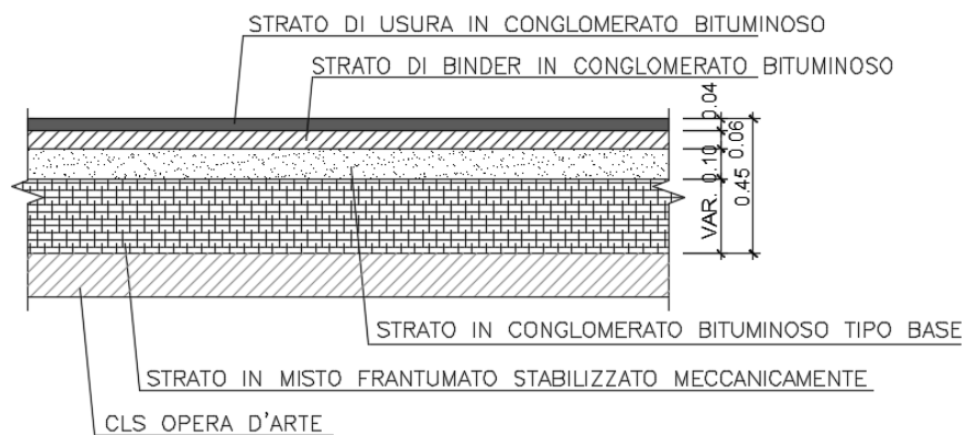
Figura 4: pavimentazione di progetto
