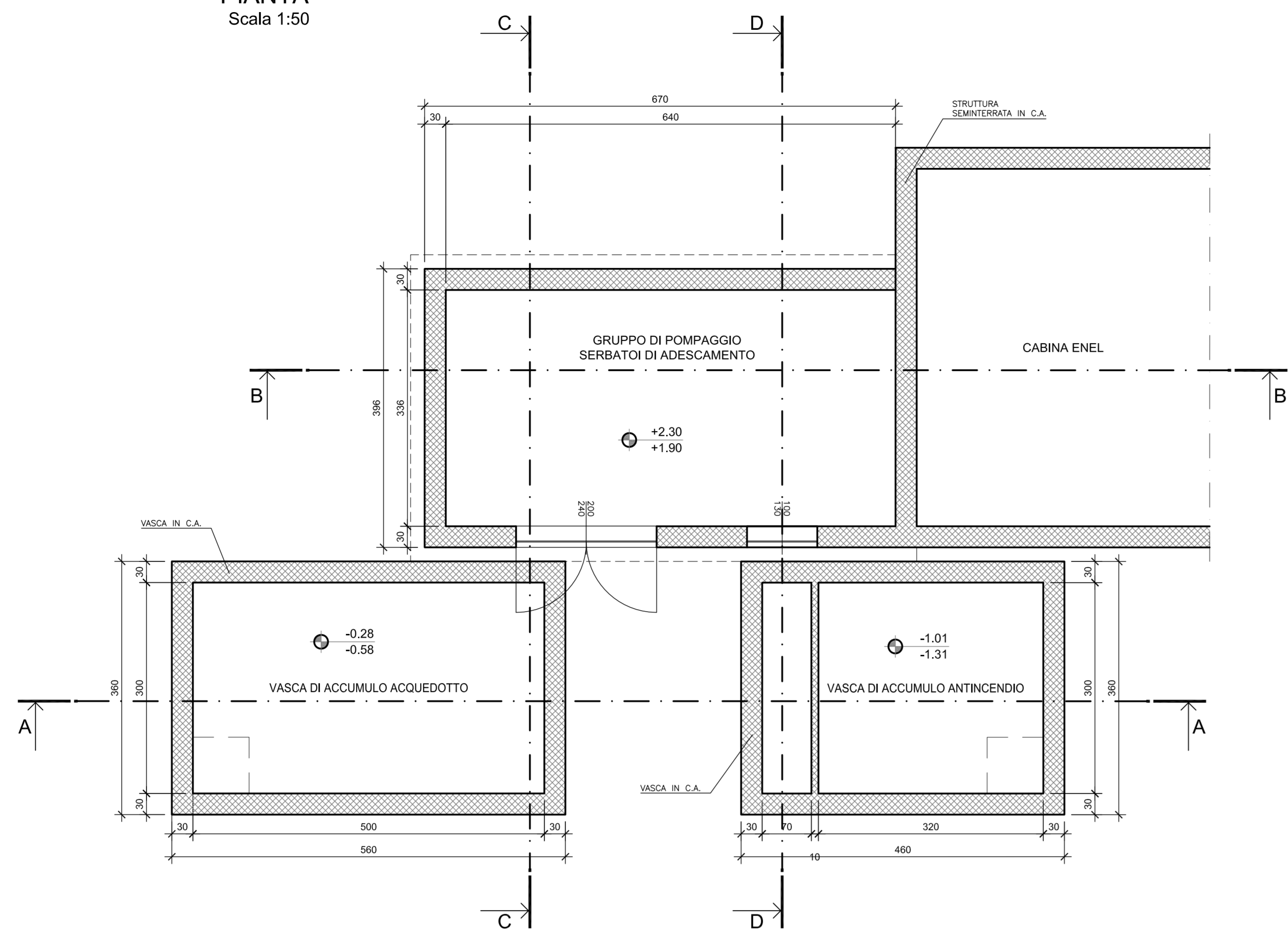
PIANTA Scala 1:50
