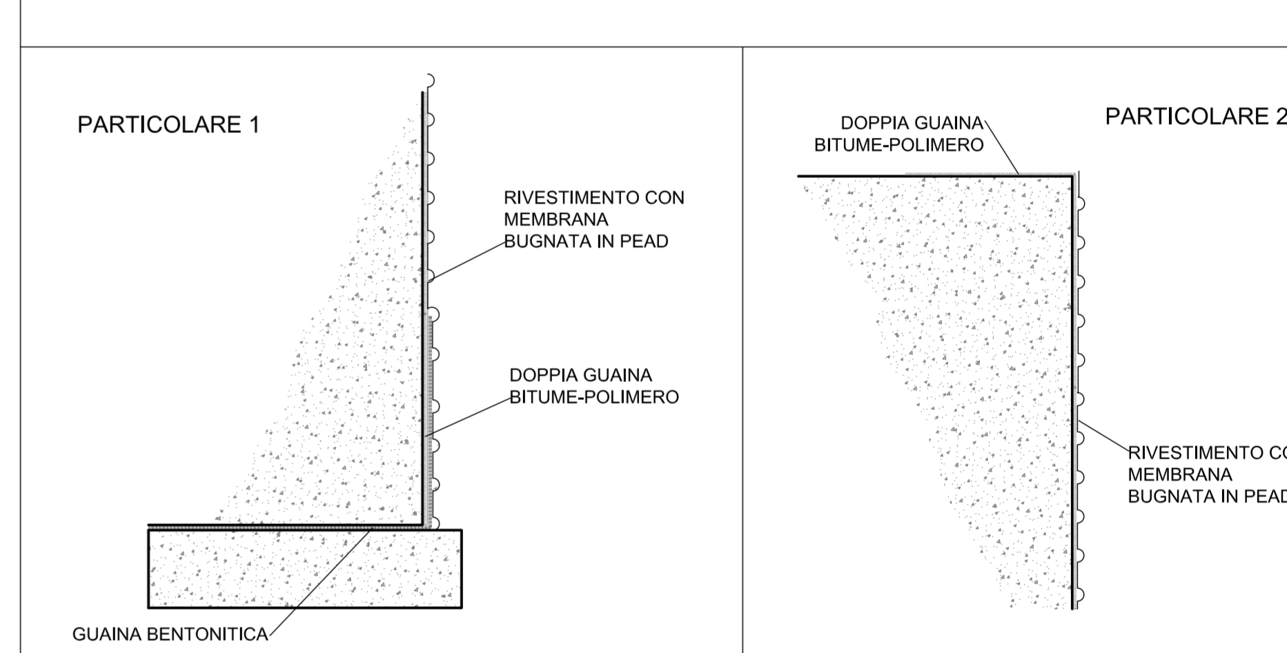
PARTICOLARE POSA GUAINE VASCHE DI ACCUMULO Scala 1:10
