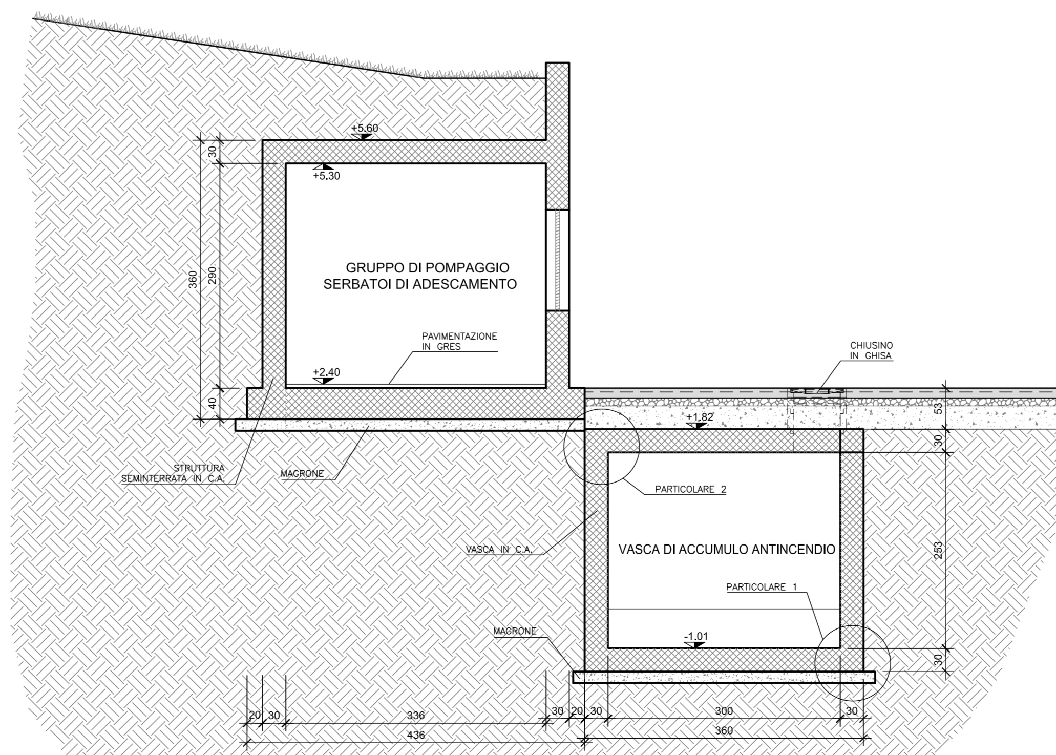
SEZIONE D-D Scala 1:50
