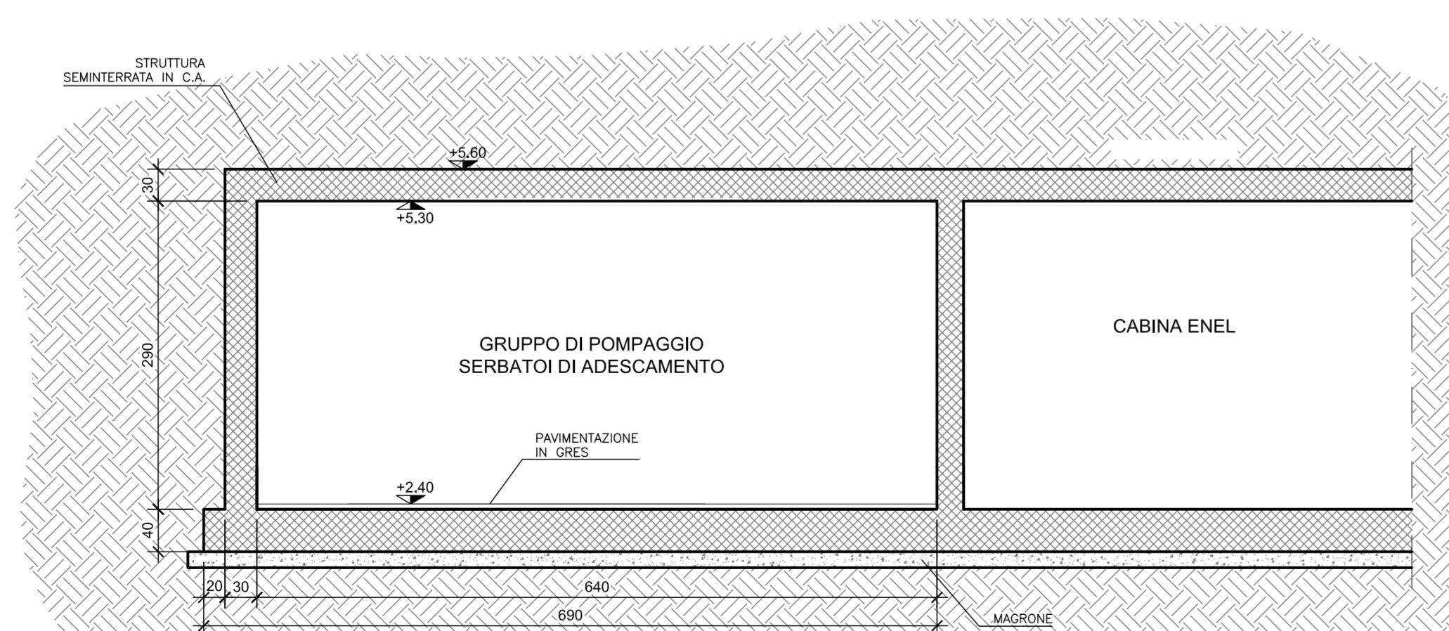
SEZIONE B-B Scala 1:50
