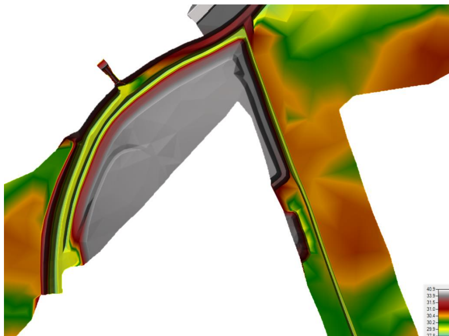
Figura 7-3 DTM ricavato da rilievo topografico (i valori riportati sono in m s. m.).
