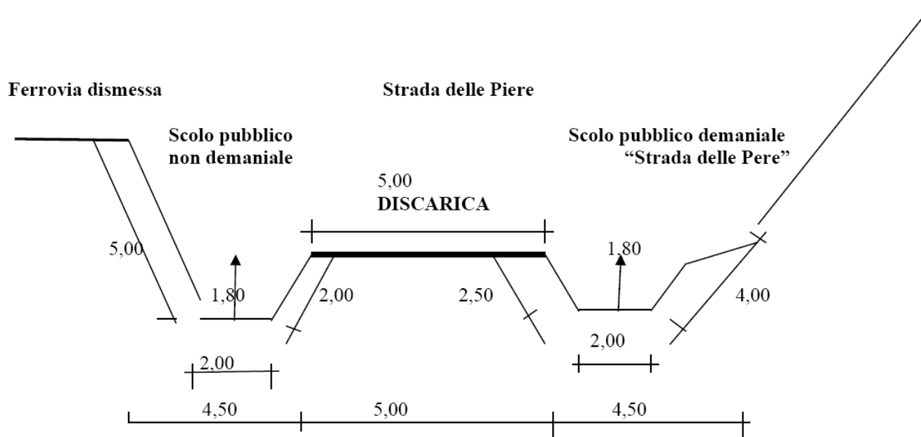
Figura 7-1 Sezione dello scolo Conterno (fonte: Consorzio di bonifica Alta pianura Veneta)
