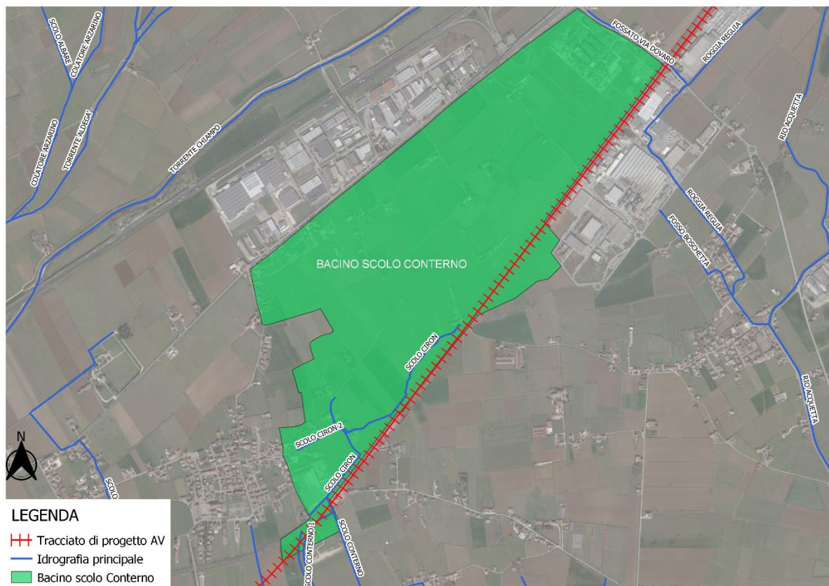
Figura 6-1 Bacino imbrifero dello scolo Conterno relativo alla deviazione di progetto
