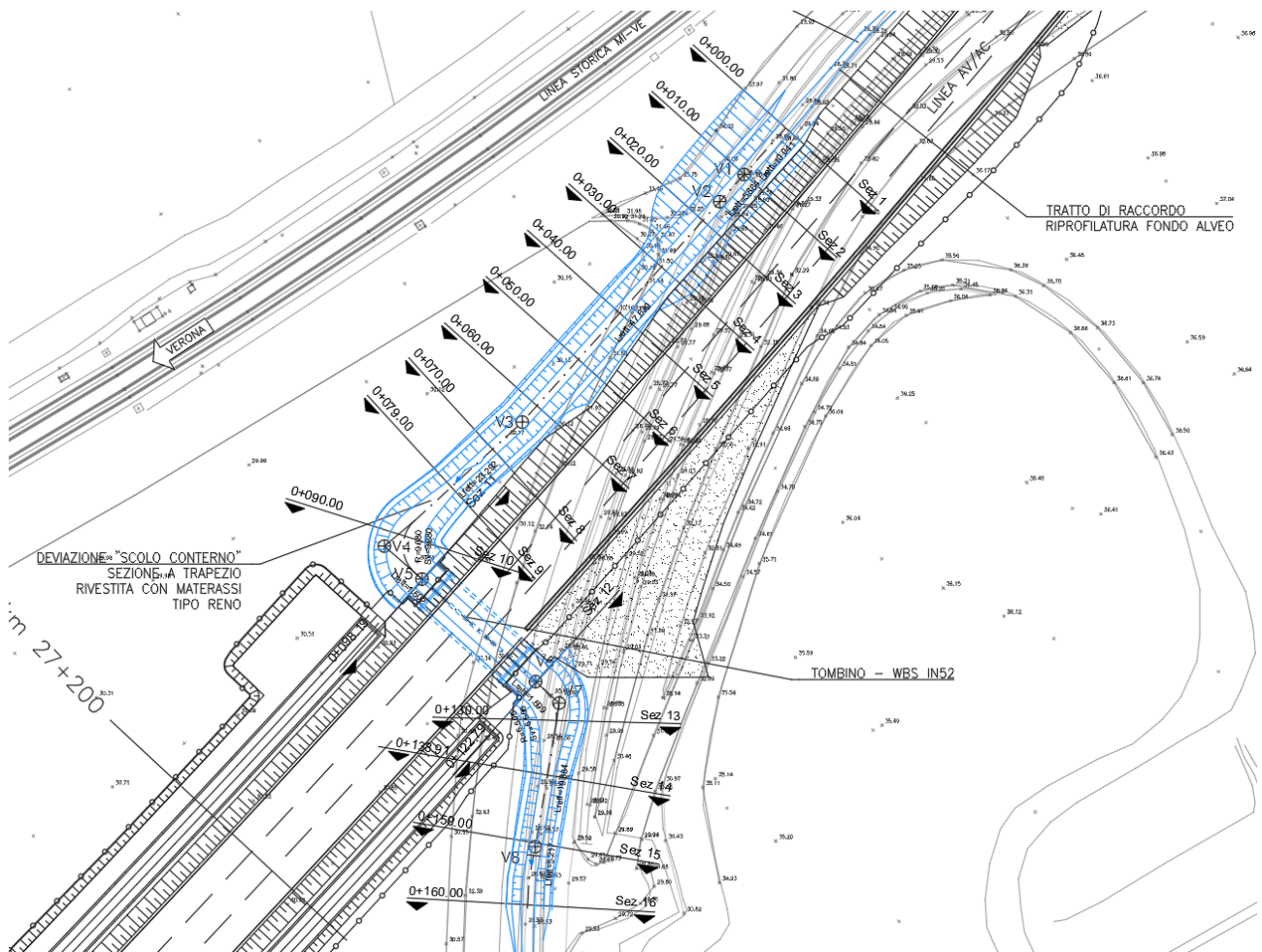
Figura 8-1 Estratto dalla planimetria di progetto post operam
