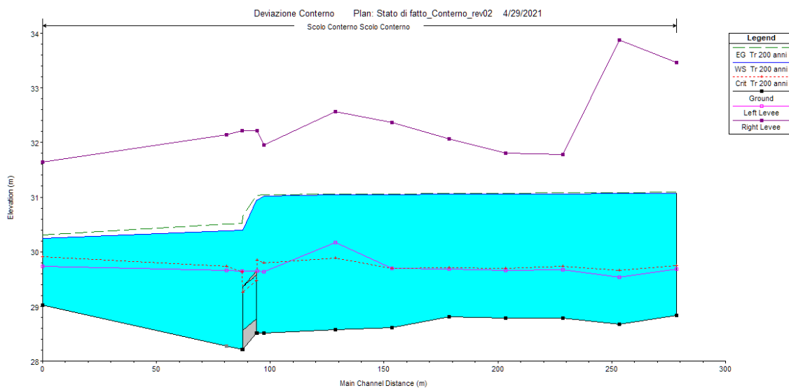
Figura 10-3 Profilo di modellazione dello scolo Conterno con portata riferita ad un Tr 200 anni, ante operam
