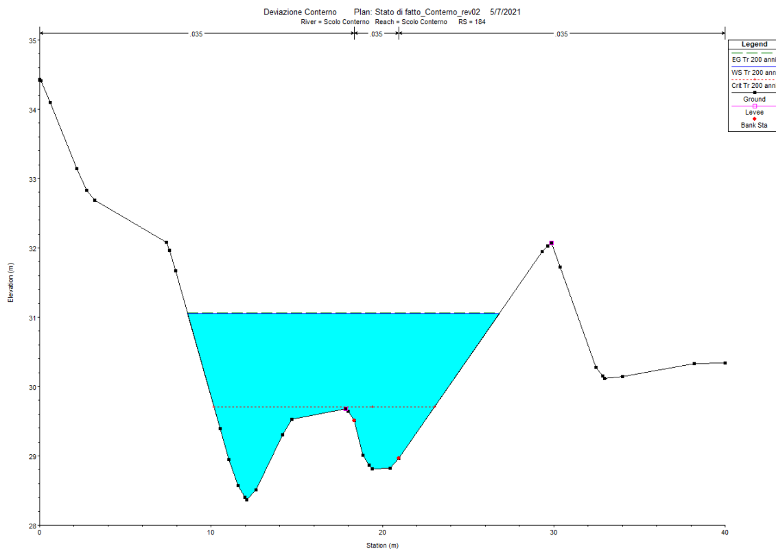
Figura 10-4 Sezione dello scolo Conterno ricavata da HEC-RAS con Tr = 200 anni
