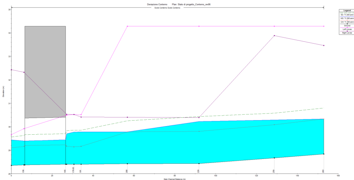
Figura 10-6 Profilo di modellazione dello scolo Conterno, post operam
