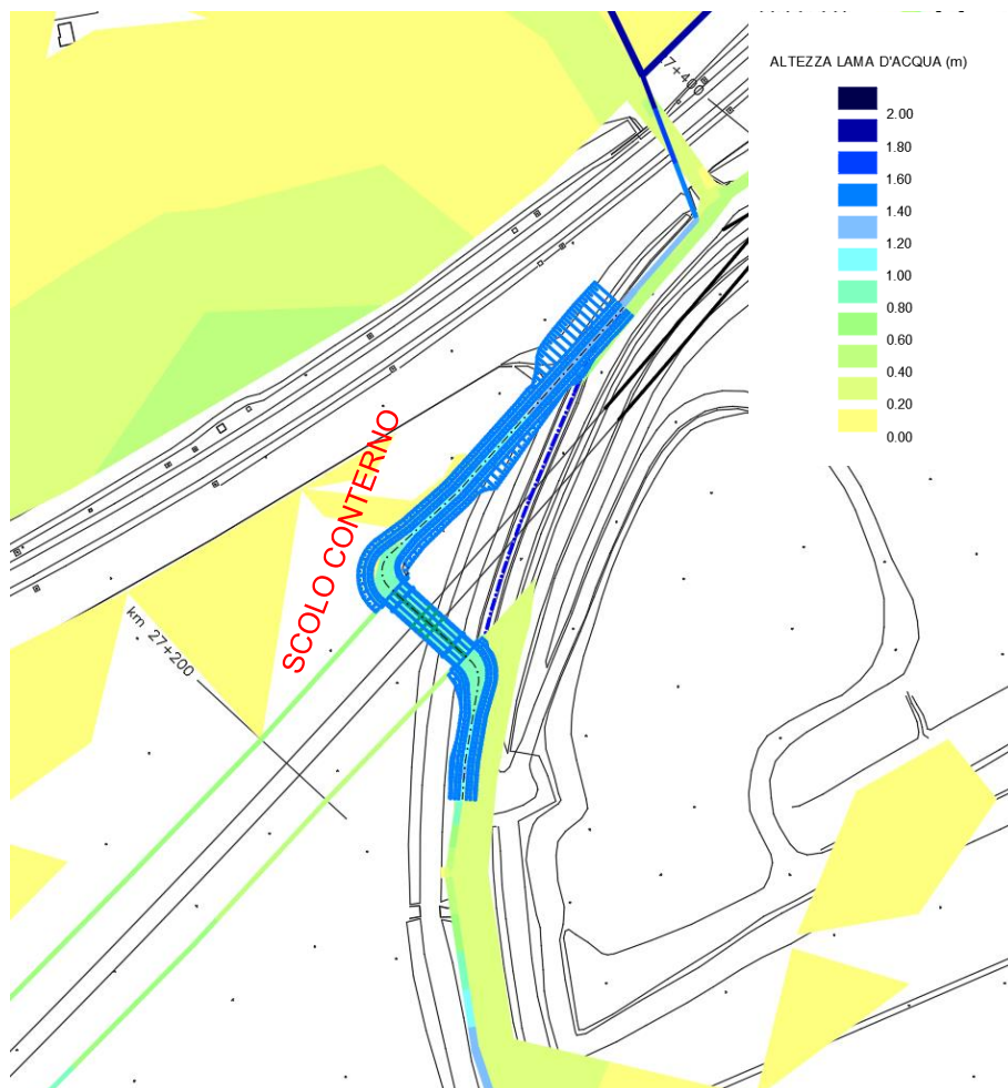
Figura 10-10 Aree di esondazione post operam, relativa alla zona dello scolo Conterno; gli allagamenti sono causati sia dall'idrografia principale sia dall'idrografia secondaria;
