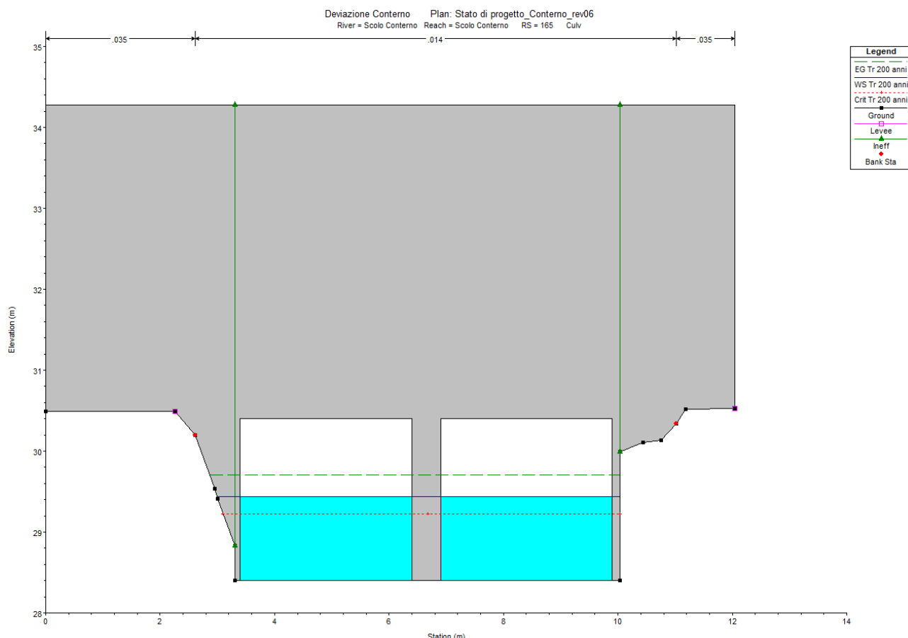
Figura 10-8 Sezione post operam estratta da HEC-RAS tombino WBS IN52
