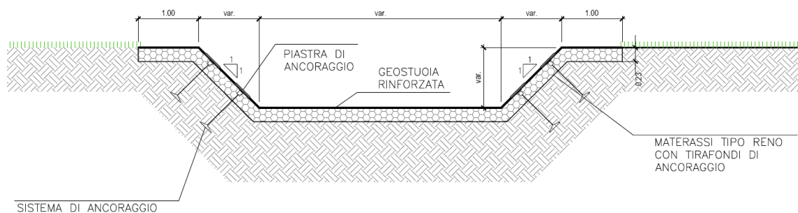
Figura 8-2 Sezione tipo trasversale scolo Conterno
