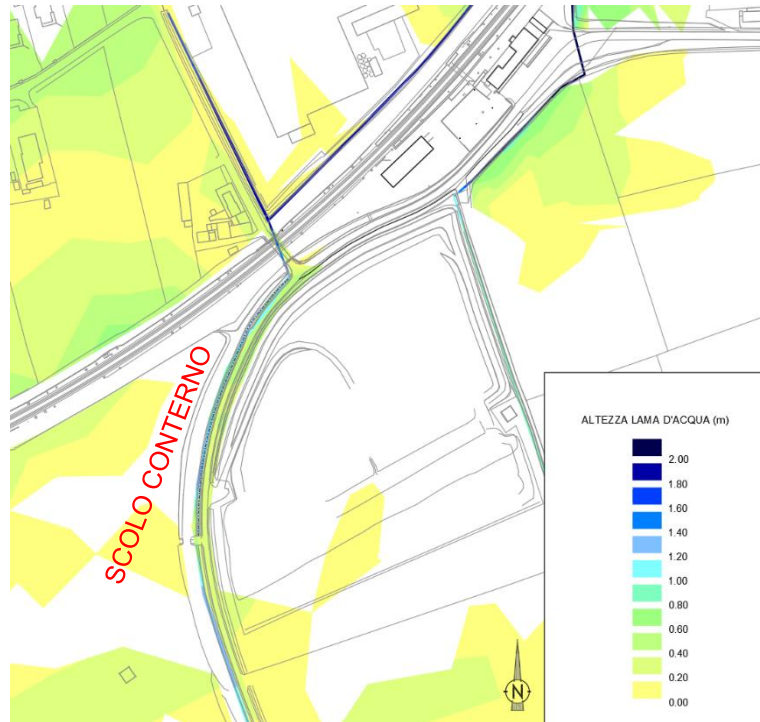
Figura 10-9 Aree di esondazione ante operam, relativa alla zona dello scolo Conterno; gli allagamenti sono causati sia dall'idrografia principale sia dall'idrografia secondaria;
