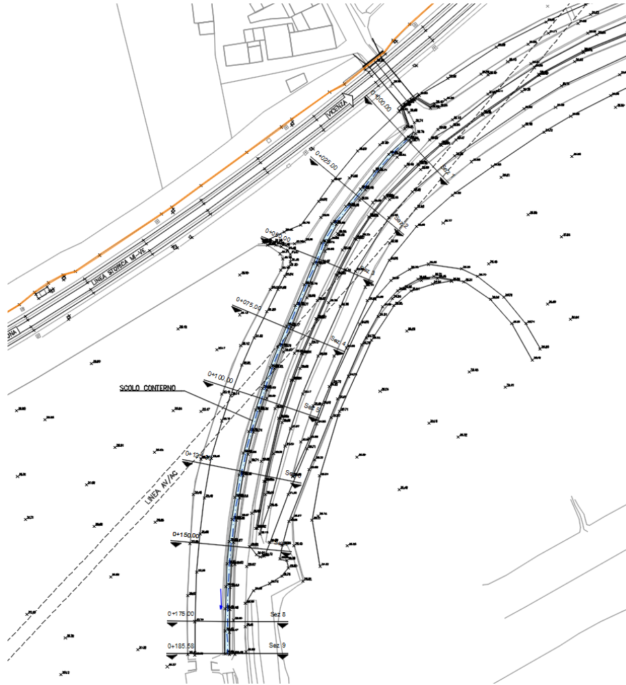
Figura 7-4 Estratto dalla tavola stato di fatto deviazione scolo Conterno
