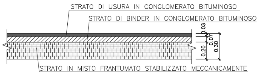
Figura 4: pavimentazione di progetto
