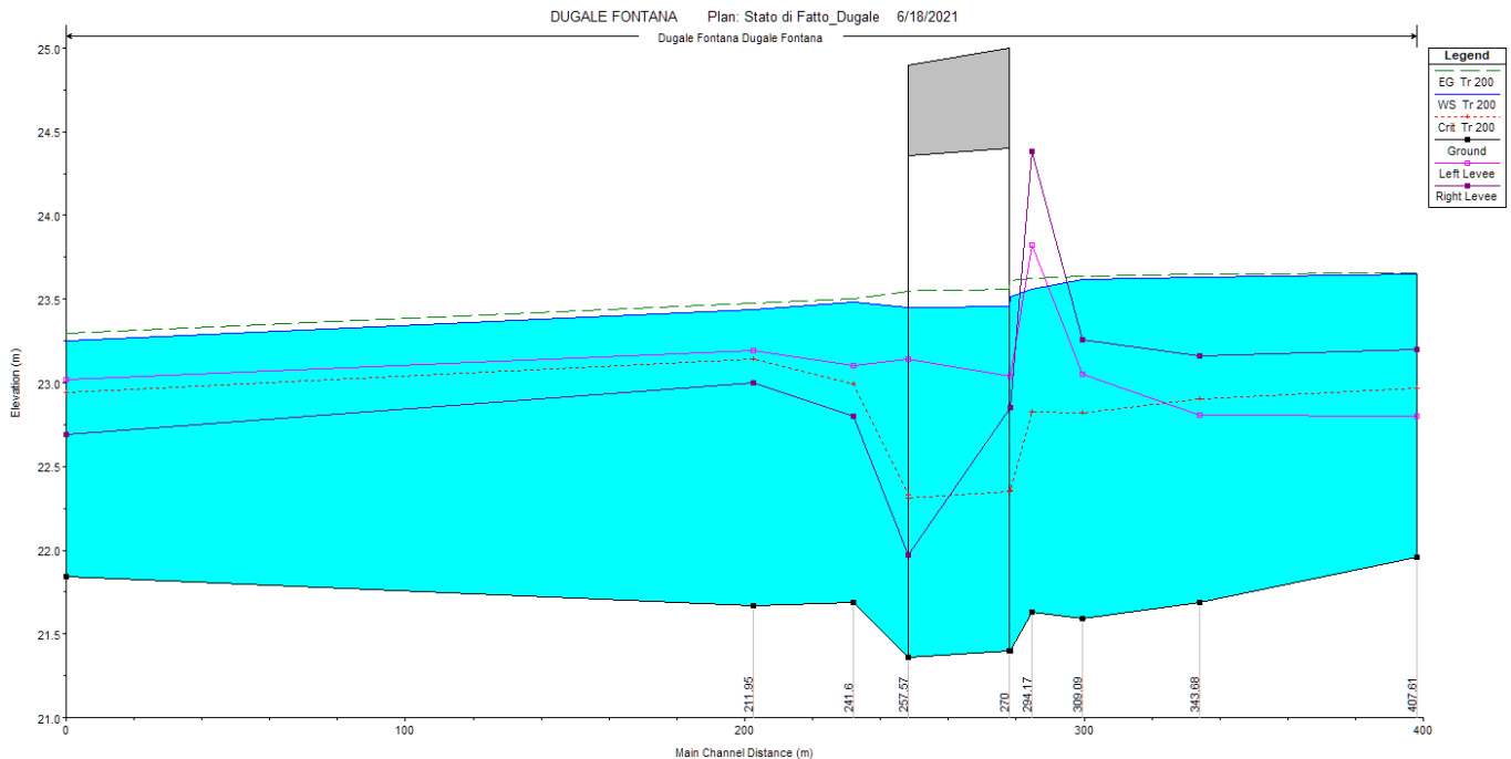
Figura 10-3 Profilo di modellazione dello Scolo Dugale con portata riferita ad un Tr 200 anni, ante operam
