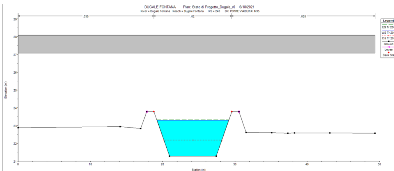
Figura 10-8 Sezione tipo post operam estratta da HEC-RAS per lo scolo Dugale in corrispondenza del ponte stradale IN35
