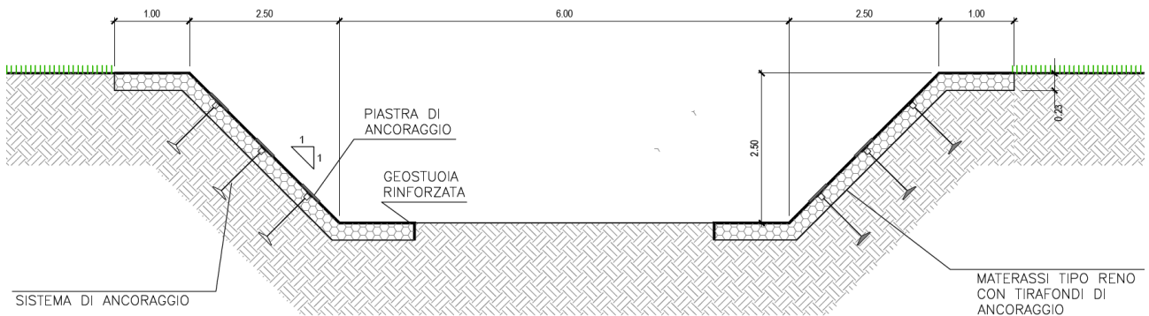
Figura 8-2 Sezione tipo trasversale scolo Dugale
