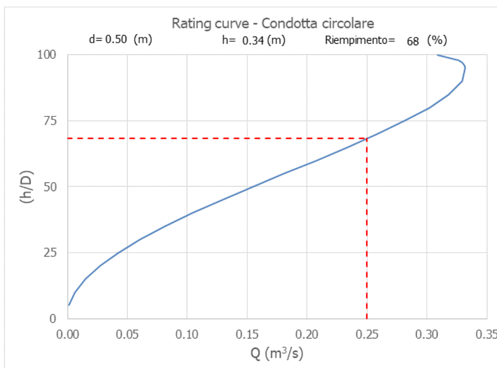
Figura 10-12 Rating curve della tubazione di drenaggio con indicazione del valore max di portata transitabile
