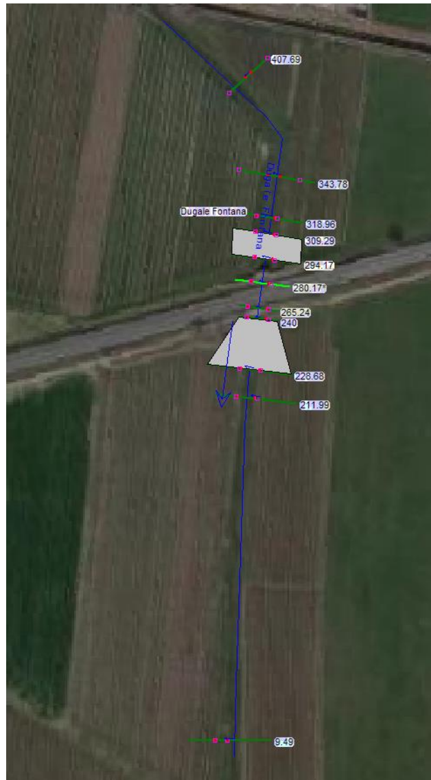
Figura 10-5 Planimetria di modellazione dello scolo Dugale, post operam
