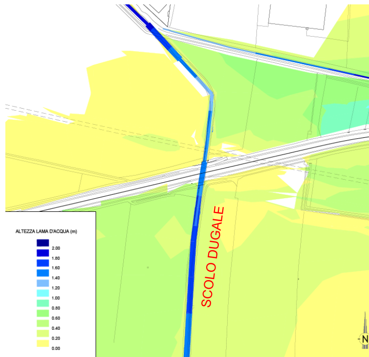
Figura 10-9 Aree di esondazione ante operam, relativa alla zona dello Scolò Dugale; gli allagamenti sono causati sia dall'idrografia principale sia dall'idrografia secondaria
