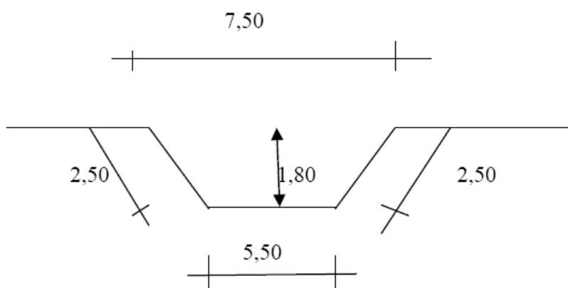
Figura 7-1 Sezione dello Scolo Dugale (fonte: Consorzio di bonifica Alta pianura Veneta)
