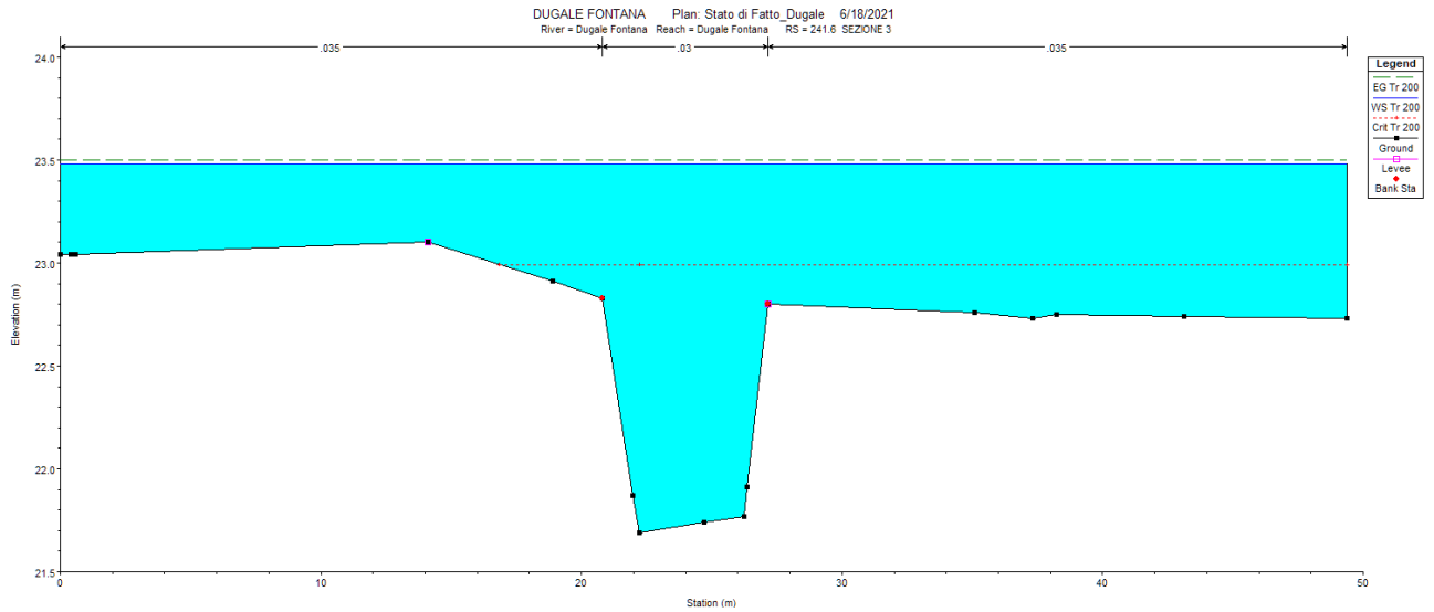
Figura 10-4 Sezione dello Scolo Dugale ricavata da HEC-RAS con un Tr = 200 anni
