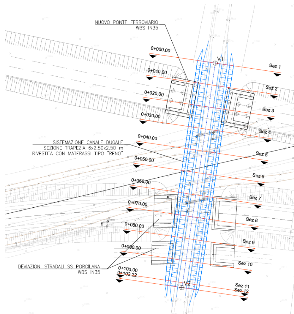
Figura 8-1 Estratto dalla planimetria di progetto post operam
