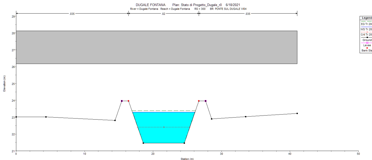
Figura 10-7 Sezione tipo post operam estratta da HEC-RAS per lo scolo Dugale in corrispondenza del ponte ferroviario VI04
