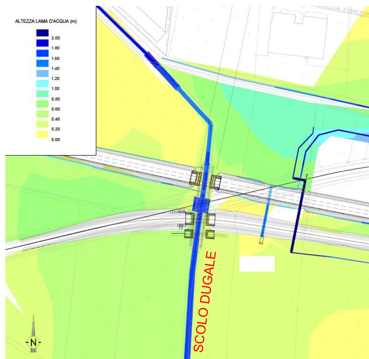
Figura 10-10 Aree di esondazione post operam, relativa alla zona dello Scolò Dugale; gli allagamenti sono causati sia dall'idrografia principale sia dall'idrografia secondaria
