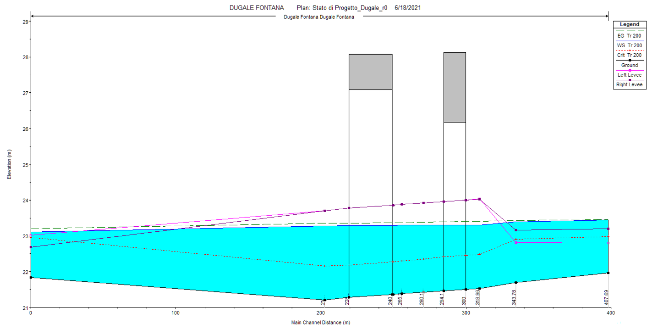
Figura 10-6 Profilo di modellazione dello Scolo Dugale, post operam
