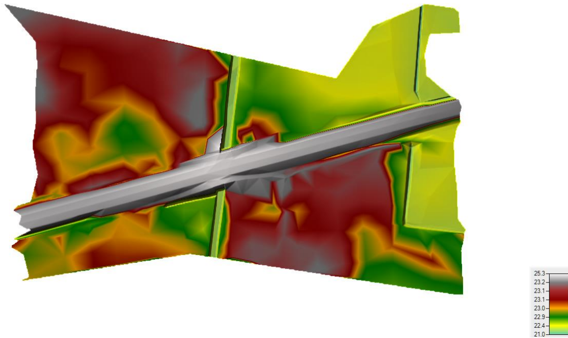
Figura 7-3 DTM ricavato da rilievo topografico (i valori riportati sono in m s. m.).
