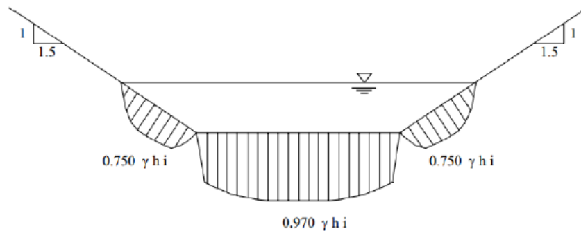
Figura 10-11 Andamento tensioni tangenziali
