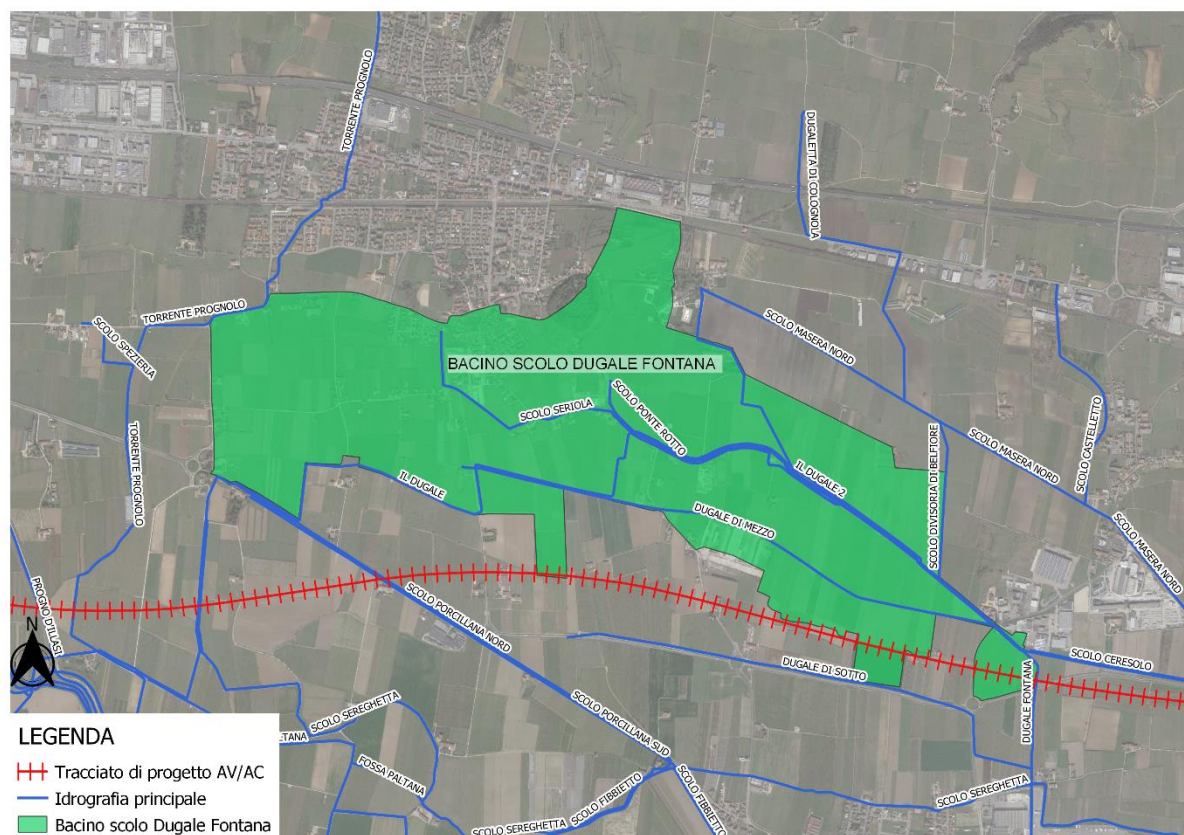
Figura 6-1 Bacino imbrifero della Scolo Dugale Fontana relativo alla sistemazione di progetto
