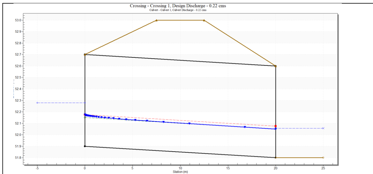
Figura 2 – Profilo di rigurgito del tombino circolare DN 600 necessario per la continuità idraulica del fosso F
