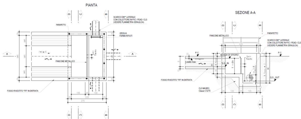
Figura 5 – Pianta e sezione tipologia dei manufatti di regolazione e scarico tipo “MC2”.
