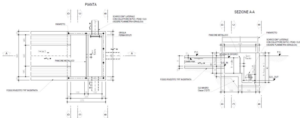
Figura 5 – Sezione tipologia dei manufatti di regolazione e scarico tipo “MC2”.
