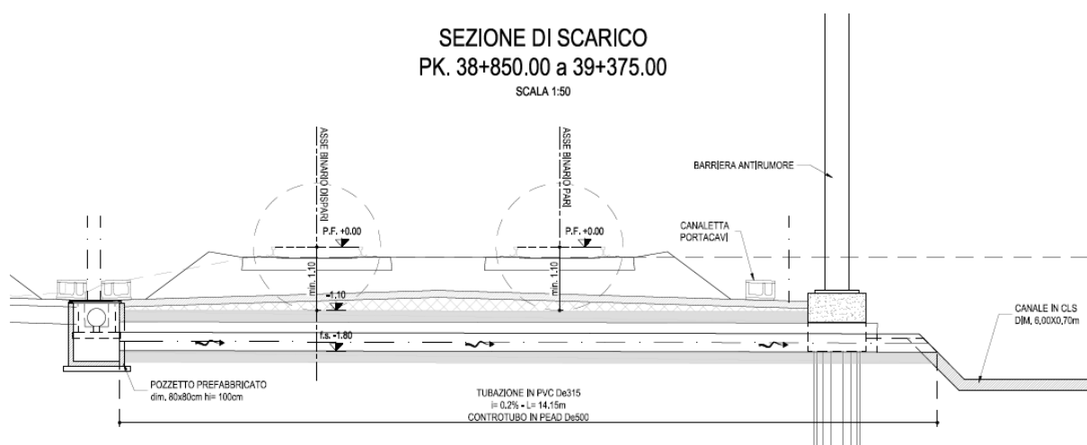
Figura 1 - Sezione di scarico delle canalette centrali nei fossi di guardia posti al piede del rilevato.
