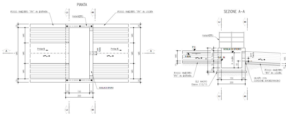
Figura 4 - Sezione tipologica dei manufatti di regolazione tipo "MC1"
