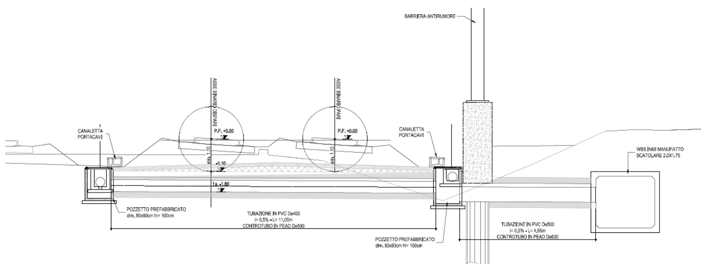
Figura 2 – Sezione del rilevato RI80 con scarico nello scolo Altavilla
