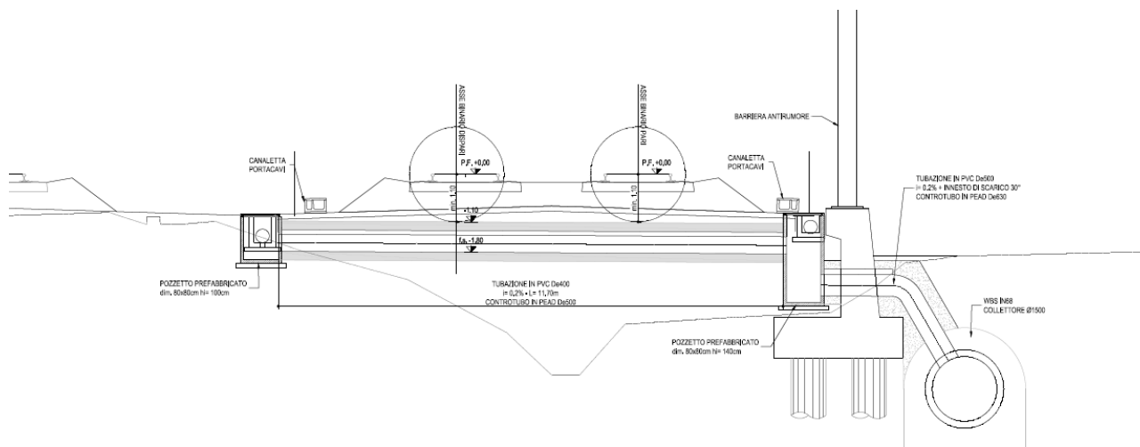
Figura 2 – Sezione del rilevato RI83 con scarico nello scolo Altavilla
