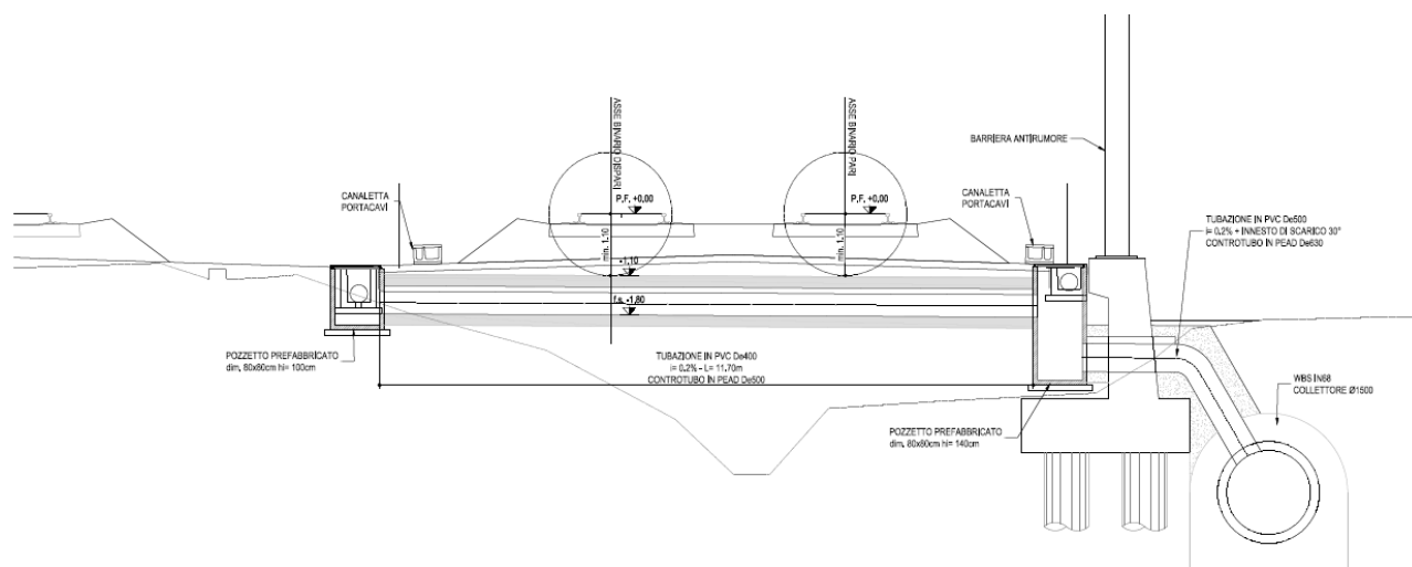
Figura 2 – Sezione del rilevato RI85 con scarico nello scolo Altavilla
