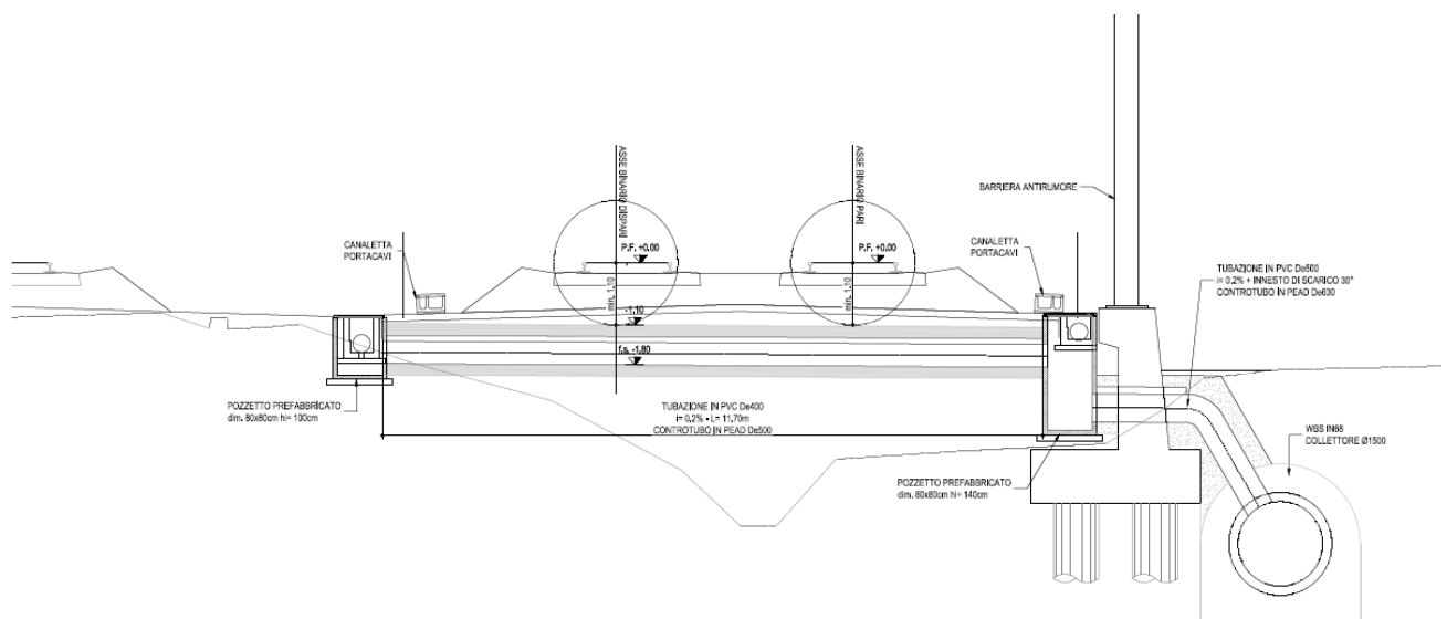
Figura 2 – Sezione del rilevato RI86 con scarico nello scolo Altavilla
