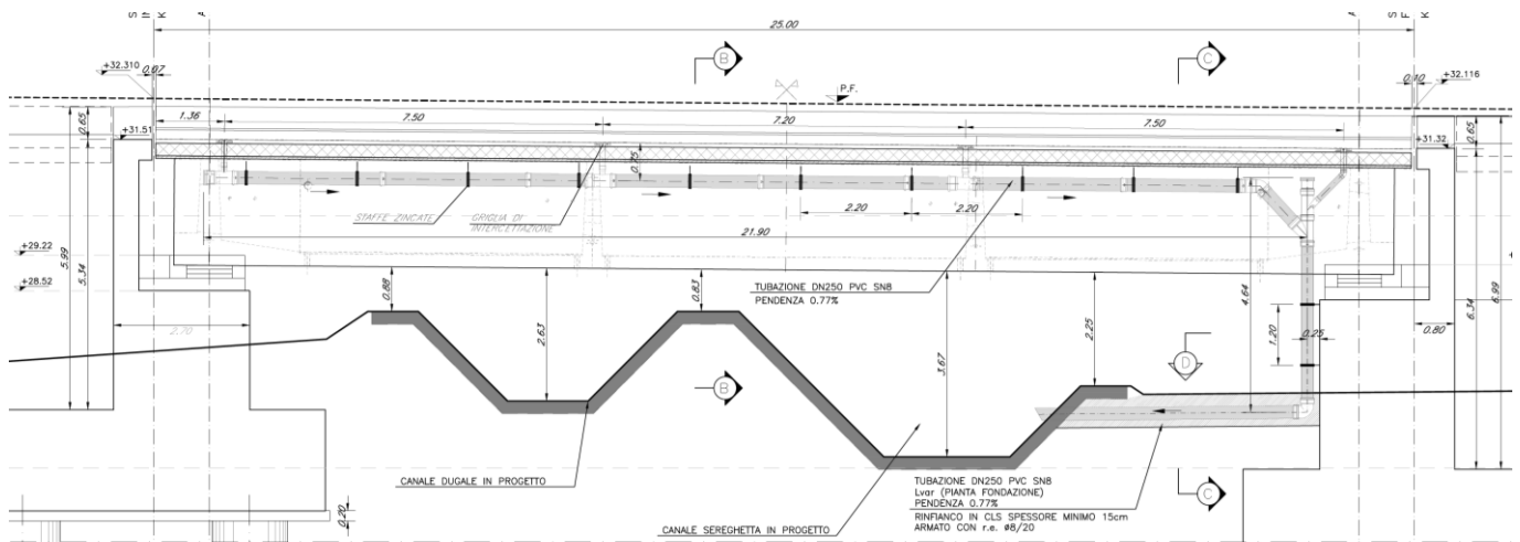
Opera di imbocco del pluviale
