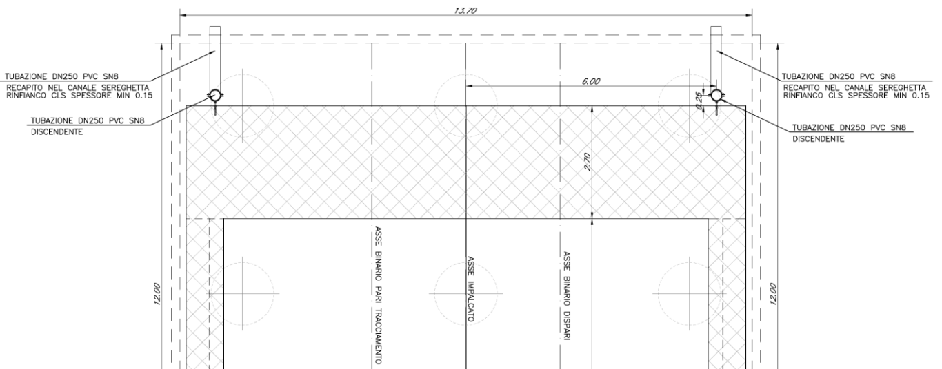
Opera di recapito L=25m
