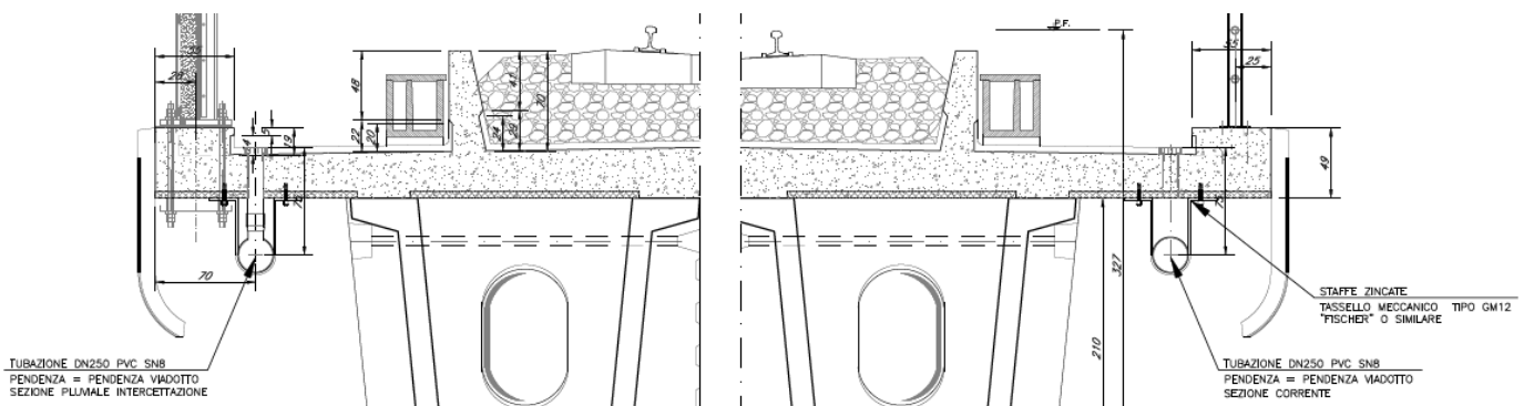
Sezione tipo di drenaggio
