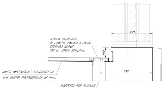
Opera di imbocco del pluviale
