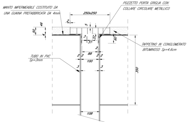
Opera di imbocco del pluviale
