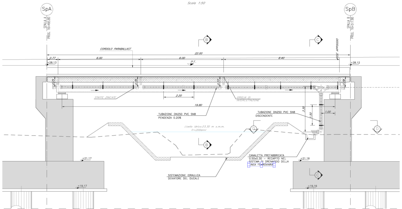
Sezione longitudinale
