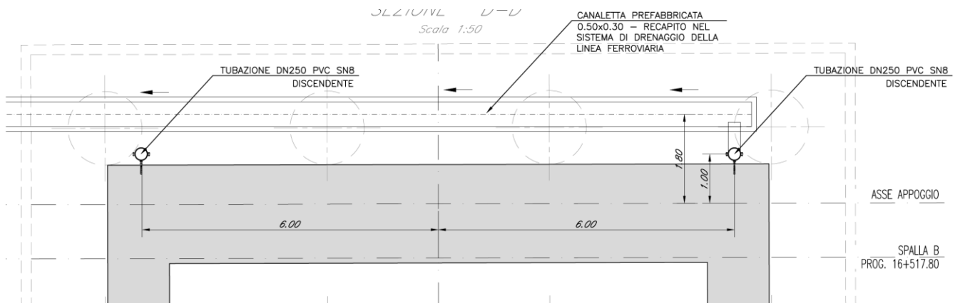
Opera di recapito Pianta
