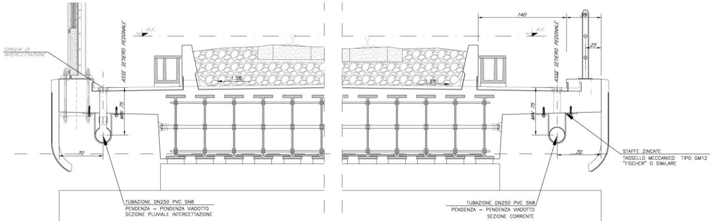
Sezione tipo di drenaggio
