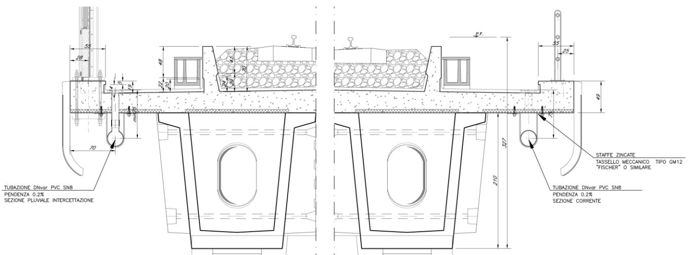
Sezione tipo di drenaggio
