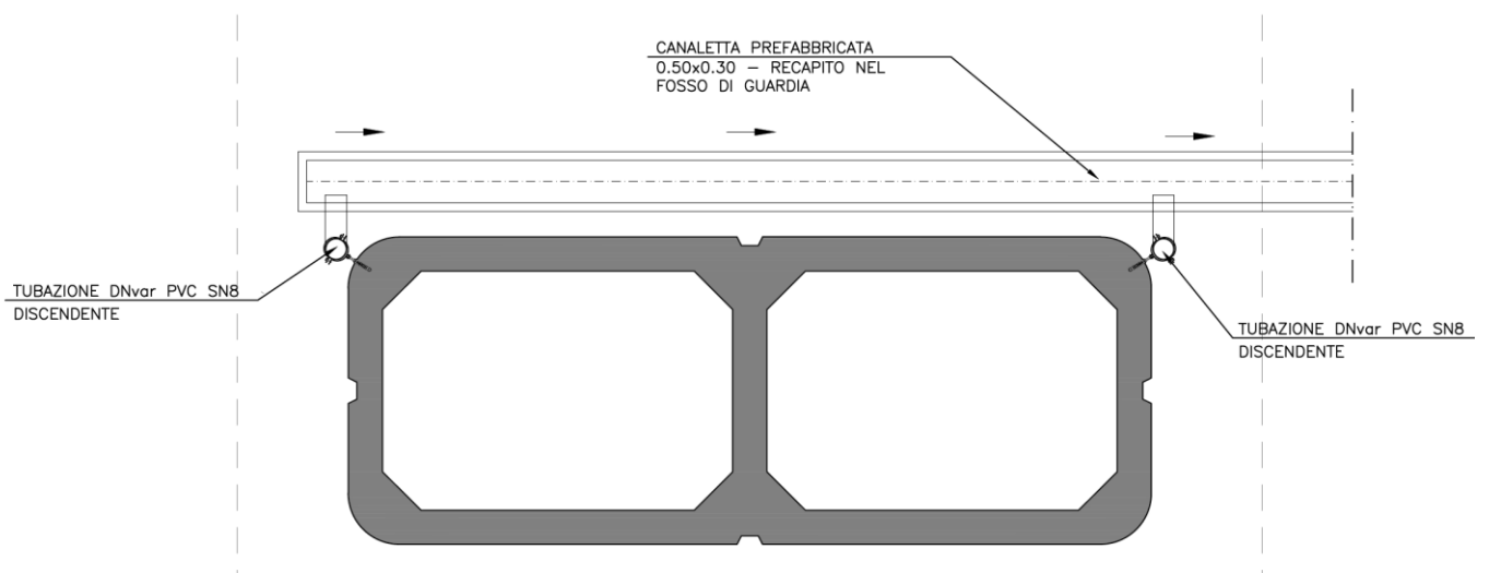
Opera di recapito L=25m - Pianta
