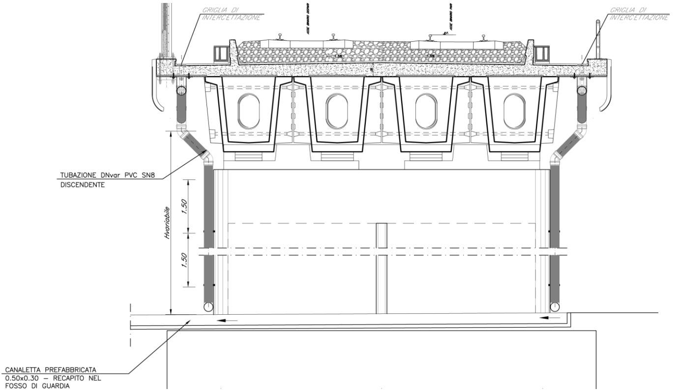
Opera di recapito L=25m - Sezione
