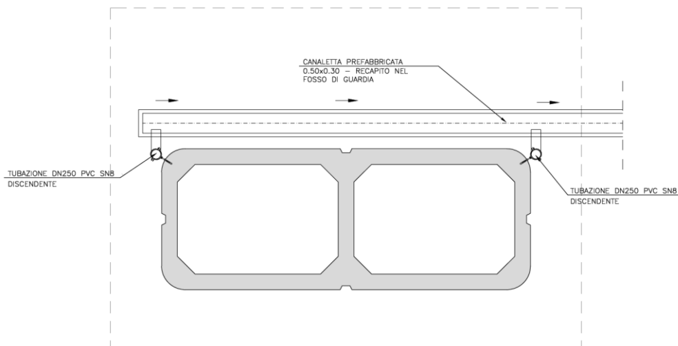
Opera di recapito L=22m
