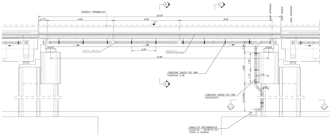
Sezione longitudinale L=22m
