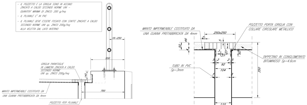
Opera di imbocco del pluviale
