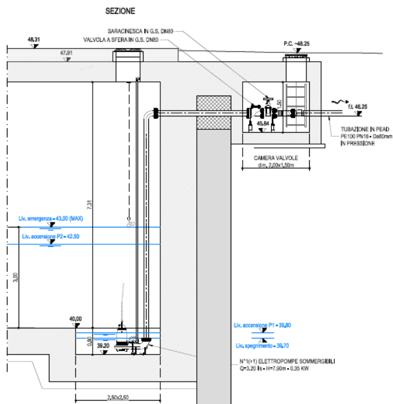
Figura 5 – Dettaglio impianto di sollevamento
