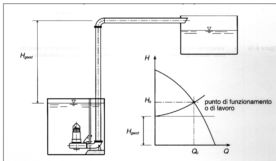
Figura 7 - Punto di lavoro: intersezione tra curva caratteristica dell'impianto e curva caratteristica della pompa
