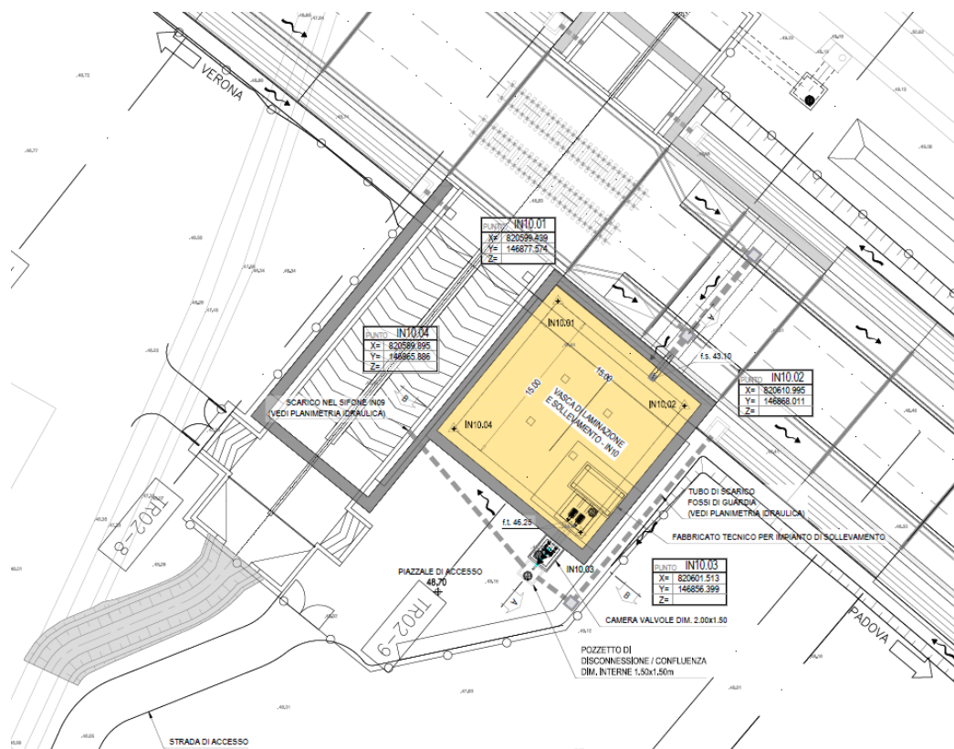
Figura 1 – Planimetria di inquadramento IN10
