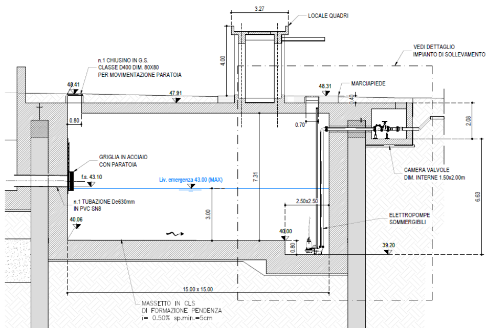
Figura 4 – Sezione longitudinale vasca di laminazione e sollevamento
