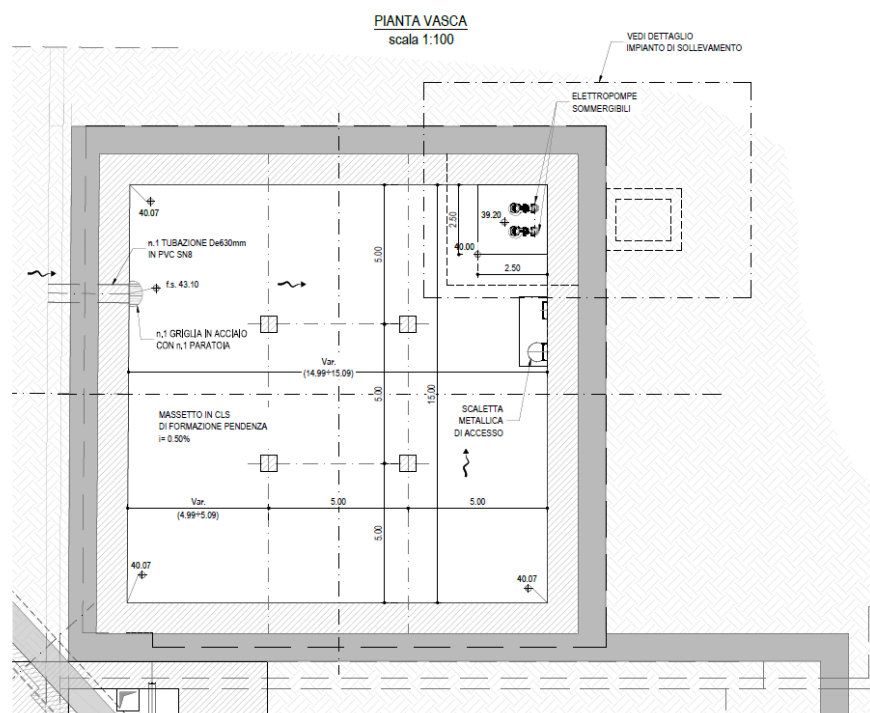
Figura 3 – Pianta vasca di laminazione e sollevamento
