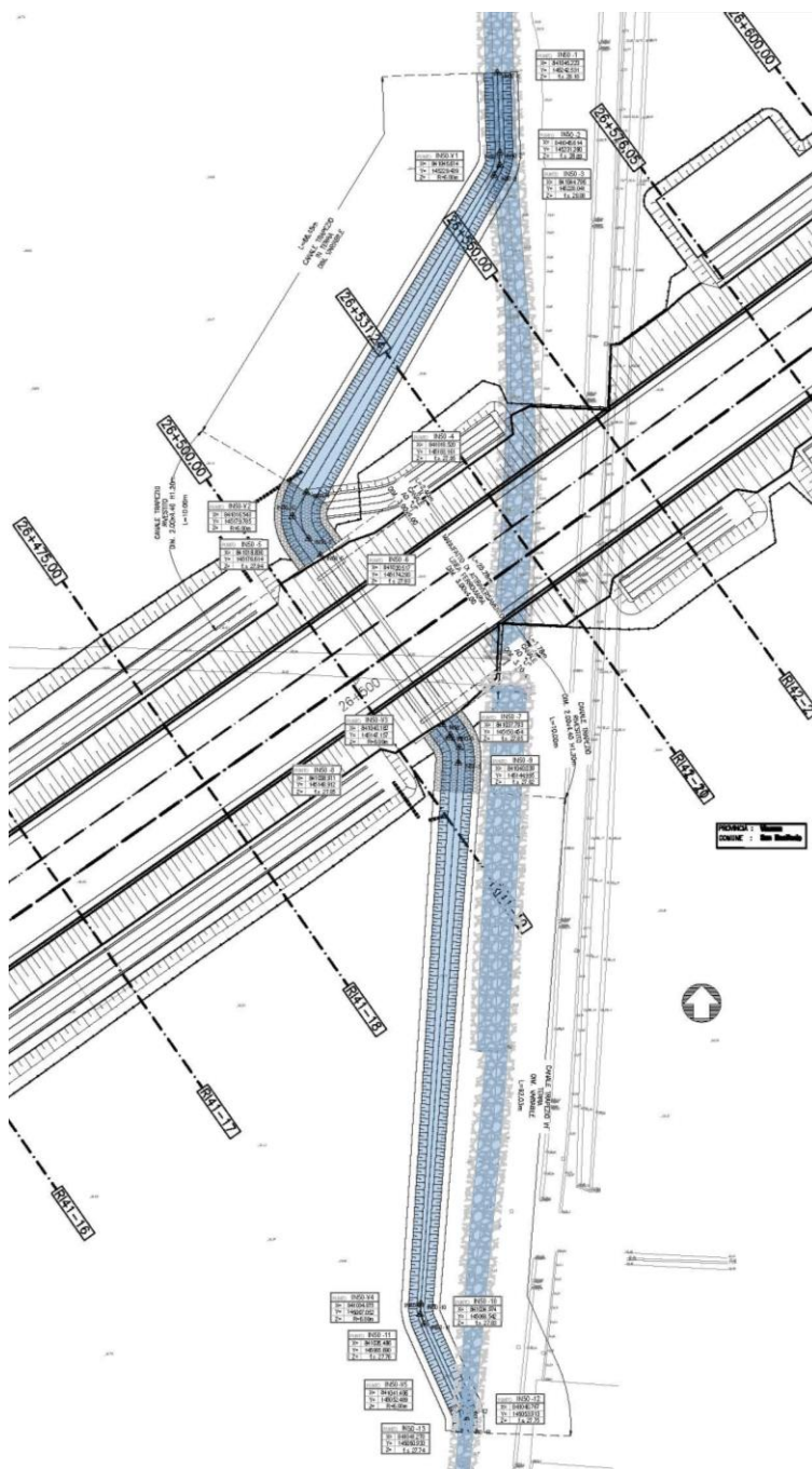
Figura 2 – Planimetria stato di progetto
