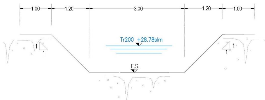
Figura 4 – Sezione tipo del canale in terra
