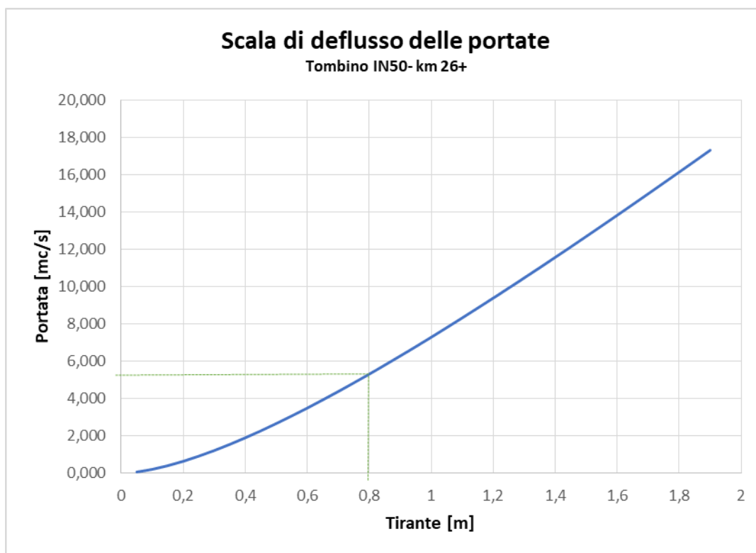
Figura 8 – Scala delle portate del tombino ferroviario IN50
