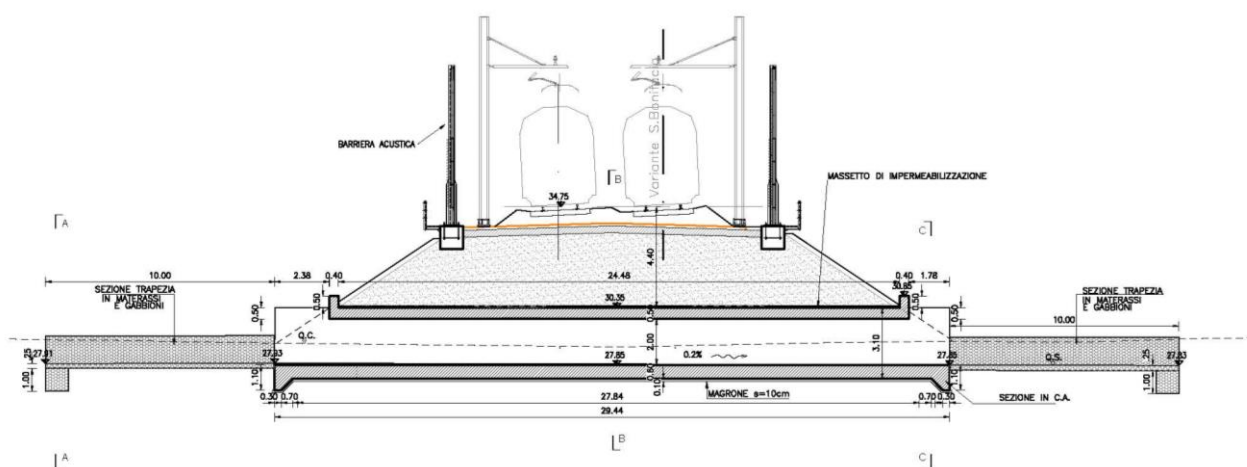
Figura 3 – Profilo di progetto del tombino IN50
