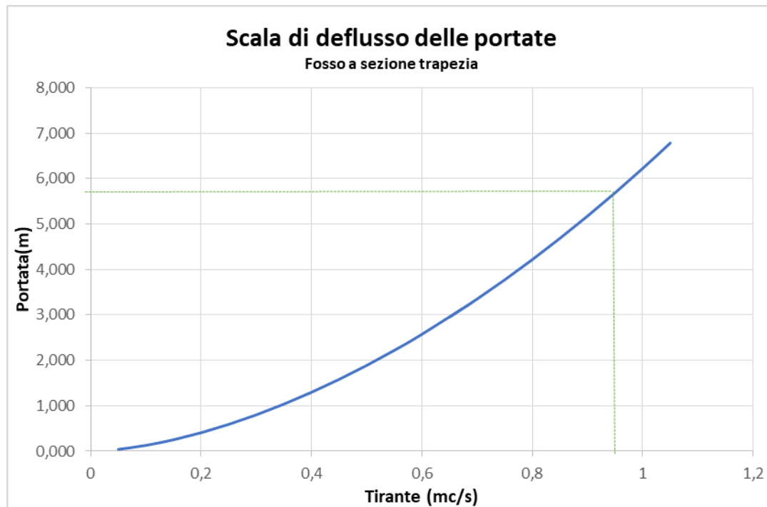
Figura 2 9– Tombino IN50 - Scala di deflusso delle portate sezione trapezia
