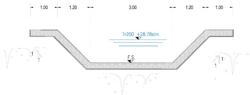
Figura 5 – Sezione tipo del canale rivestito in materassi tipo reno.
