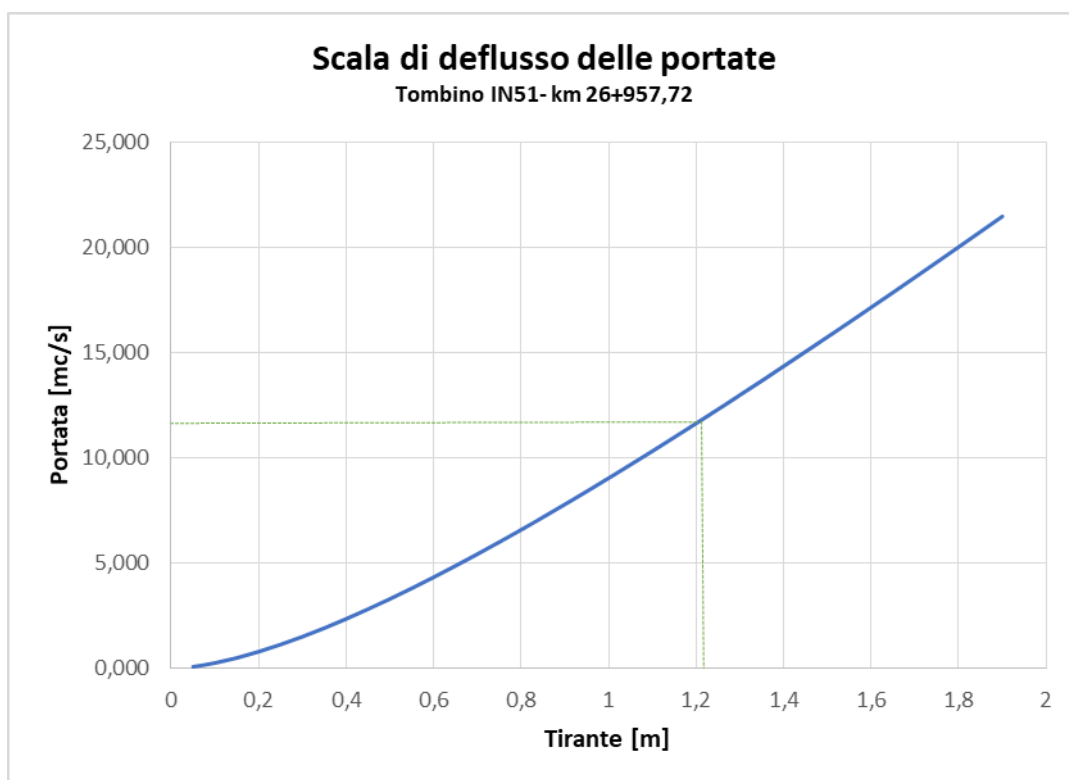
Figura 8 – Scala delle portate del tombino ferroviario IN51
