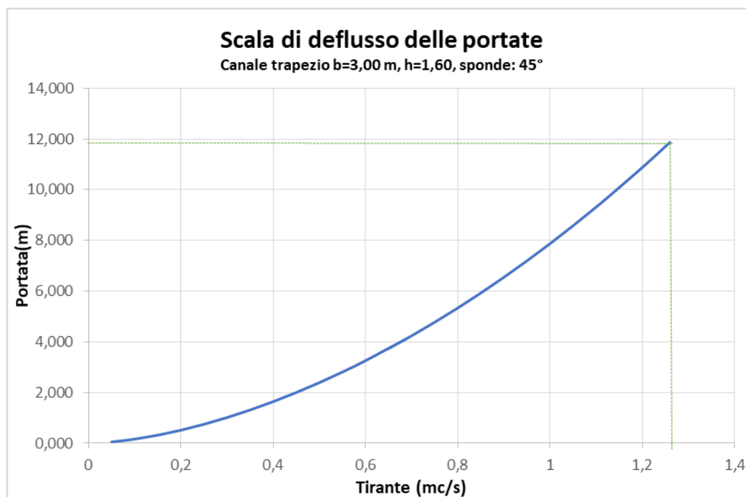
Figura 9– Tombino IN51 - Scala di deflusso delle portate sezione trapezia
