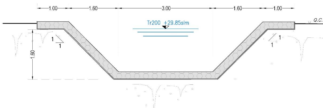
Figura 5– Sezione tipo del canale rivestito in materassi reno
