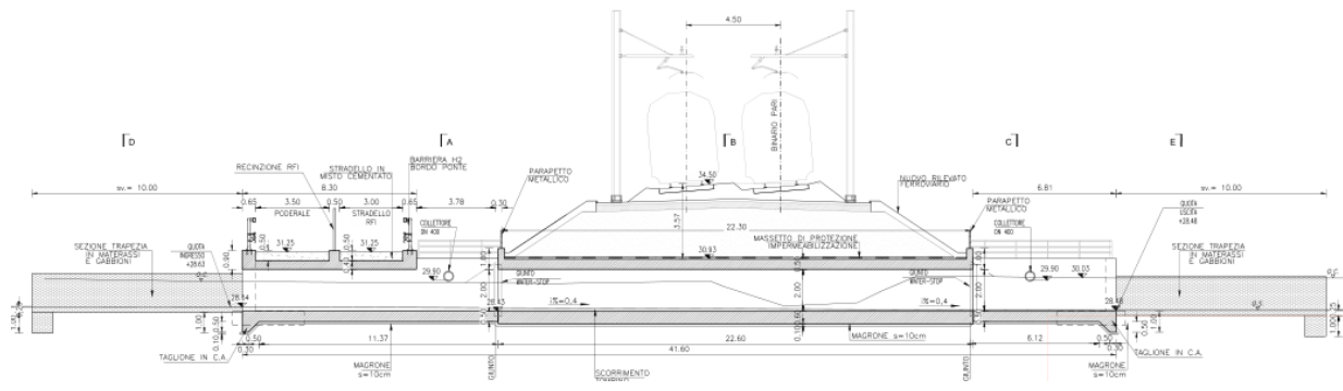
Figura 3 – Profilo di progetto del tombino IN51
