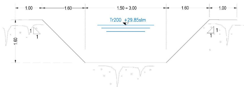
Figura 4– Sezione tipo del canale in terra
