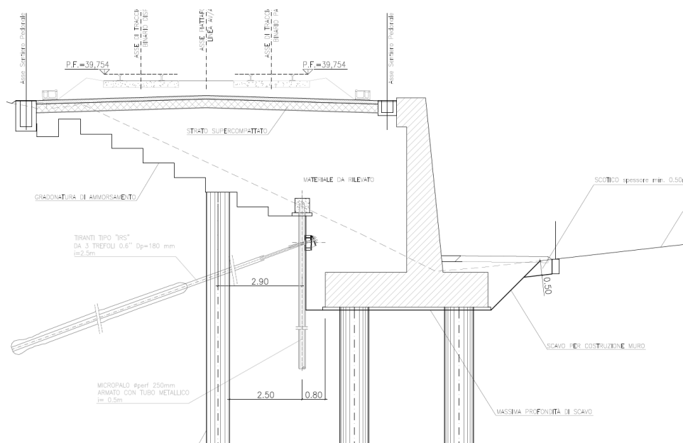
Figura 1 - Progetto Esecutivo - sezione di intervento Ri52
