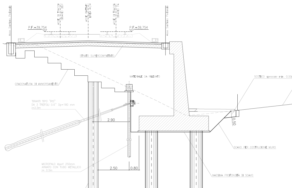
Figura 1 - Progetto Esecutivo - sezione di intervento Ri53
