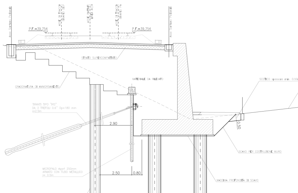
Figura 1 - Progetto Esecutivo - sezione di intervento Ri55
