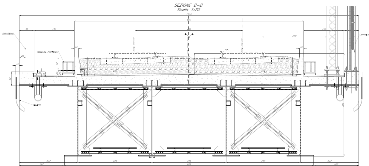
Fig. 3: Sezione trasversale dell'impalcato misto a 4 travi
