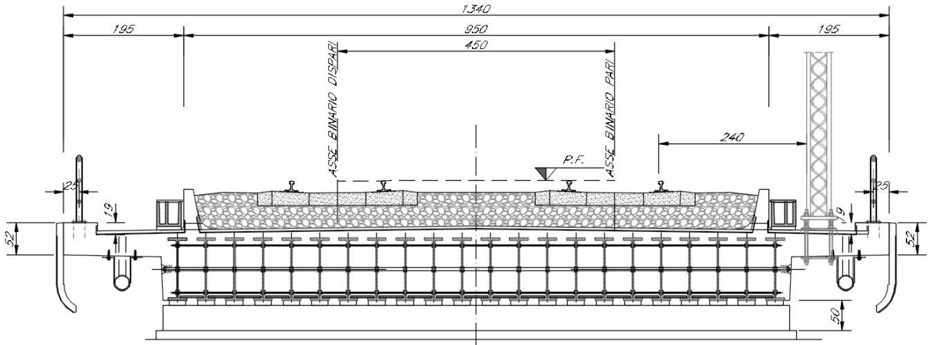
Fig. 7: Sezione trasversale dell'impalcato a travi incorporate
