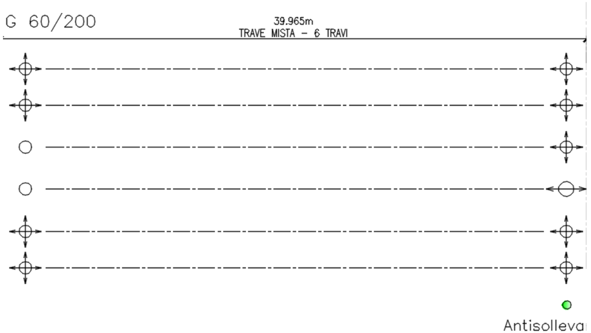
Fig. 6: Schema appoggi misto 6 travi
