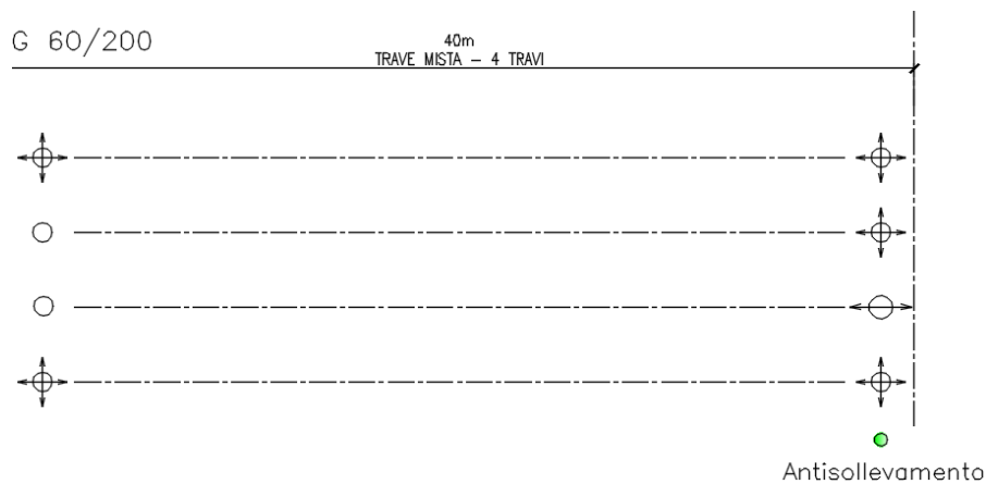
Fig. 4: Schema appoggi misto 4 travi
