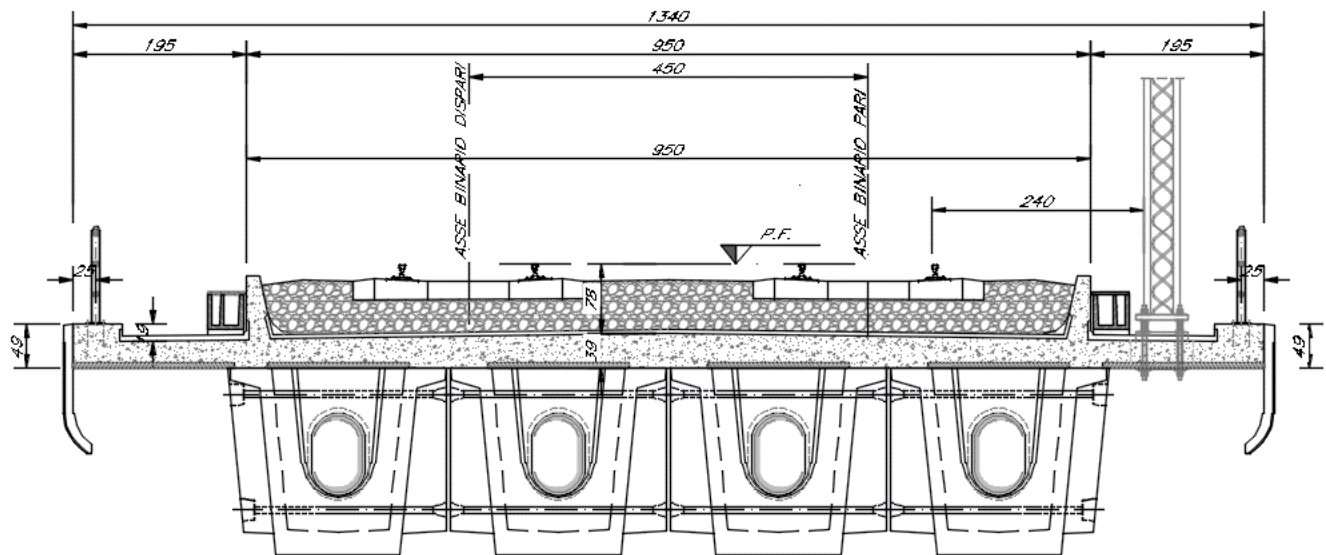
Fig. 1: Sezione trasversale dell'impalcato in c.a.p.
