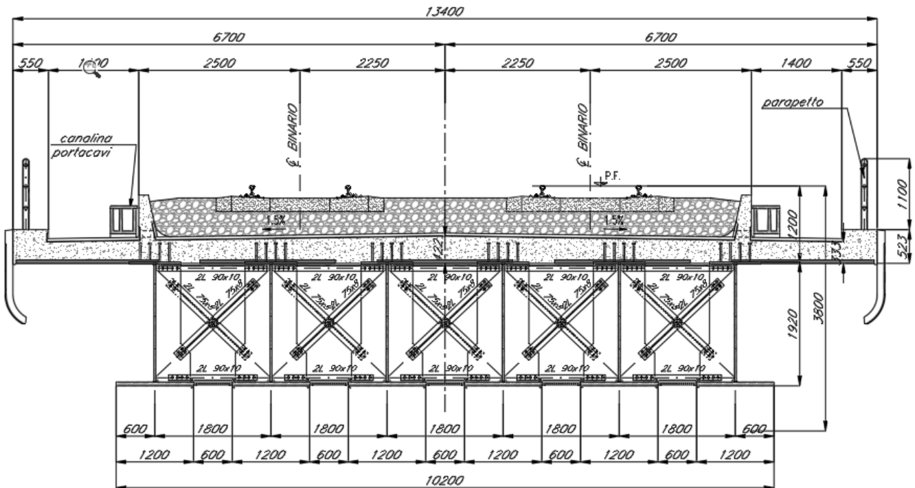
Fig. 5: Sezione trasversale dell'impalcato misto a 6 travi
