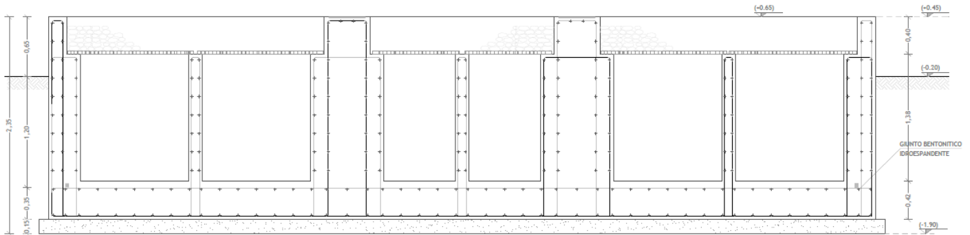
Fig. Pianta e sezione Trasformatore di potenza 150 kW
