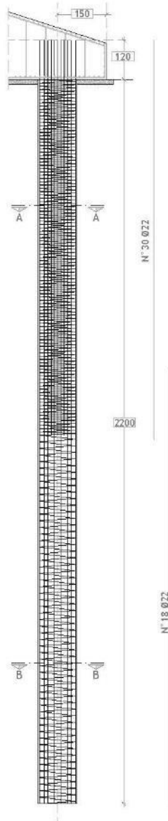
DETTAGLIO ARMATURA PALI
