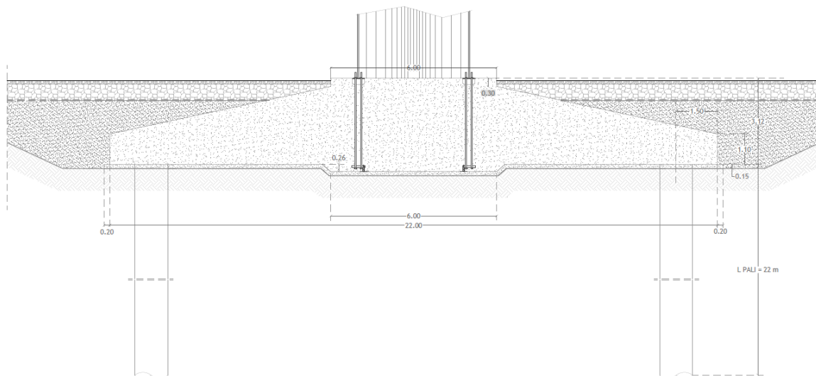
fig. Dettaglio sezione fondazione
