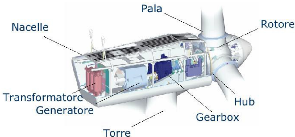
Figura 1 – Elementi dell'aerogeneratore
