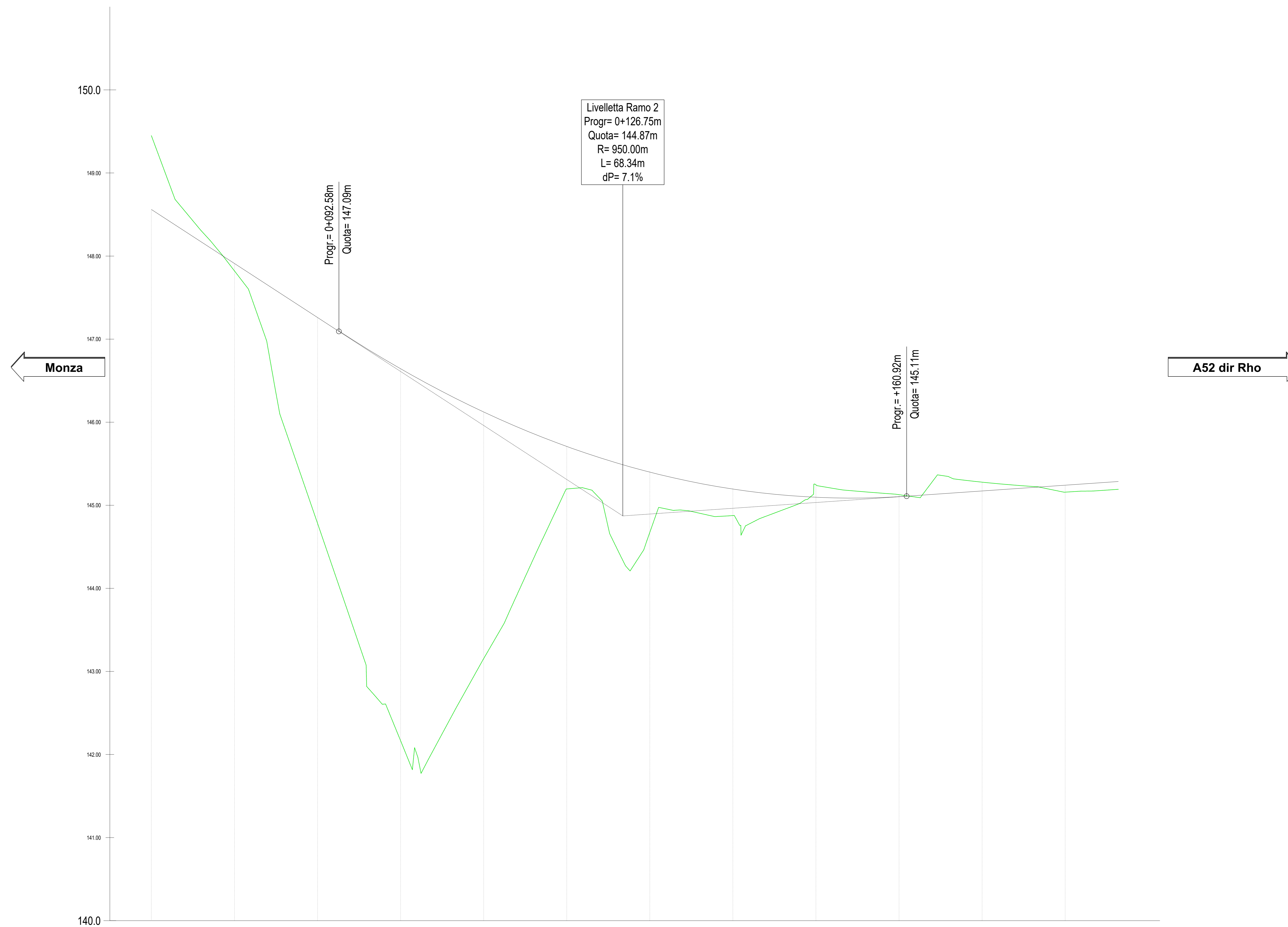
Profilo: Vista Profilo - (2) Scala : 200:20 Q.Rif. : 140.00
